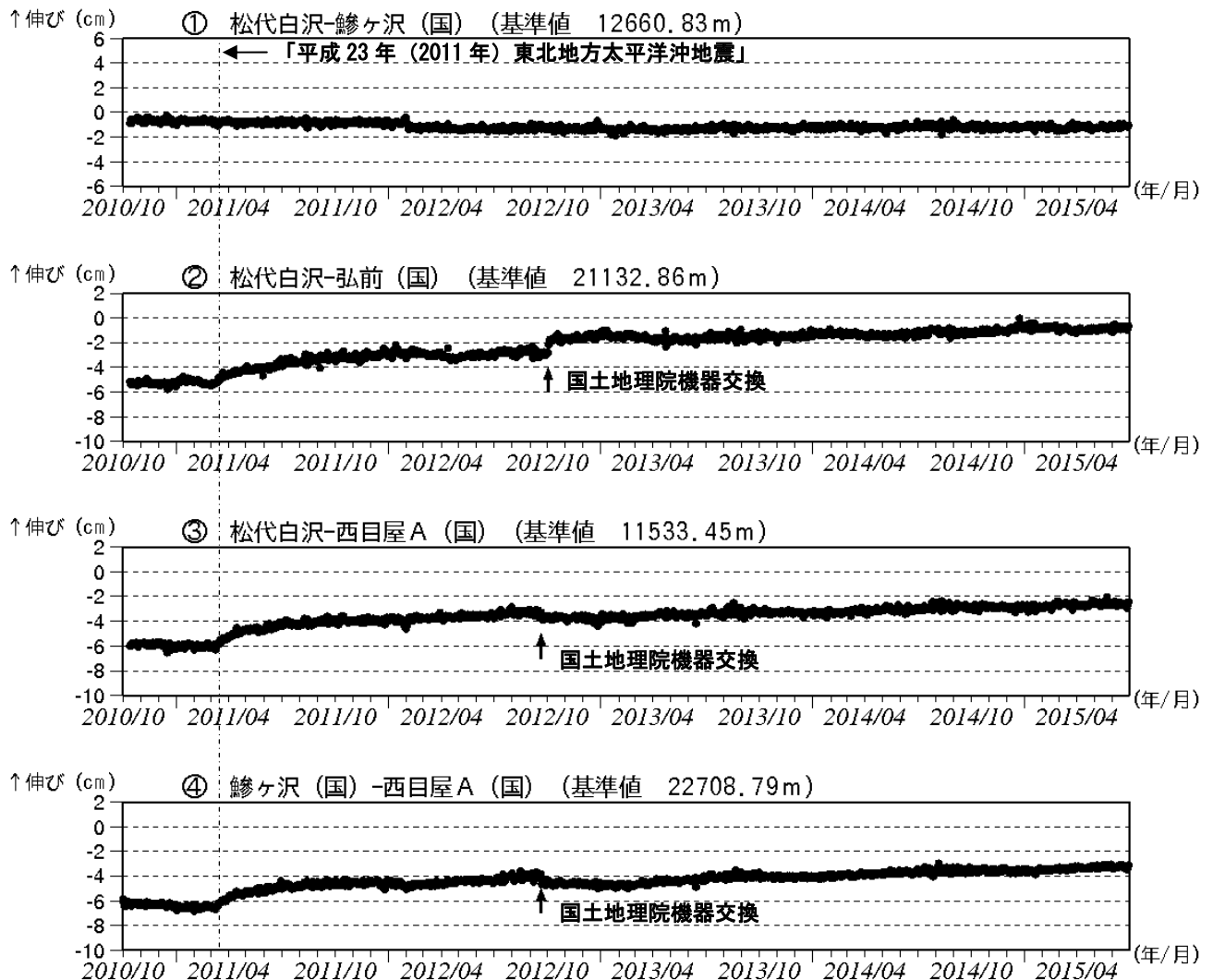
図3 岩木山 GNSS 1) 基線長変化図（2010年10月～2015年6月）
