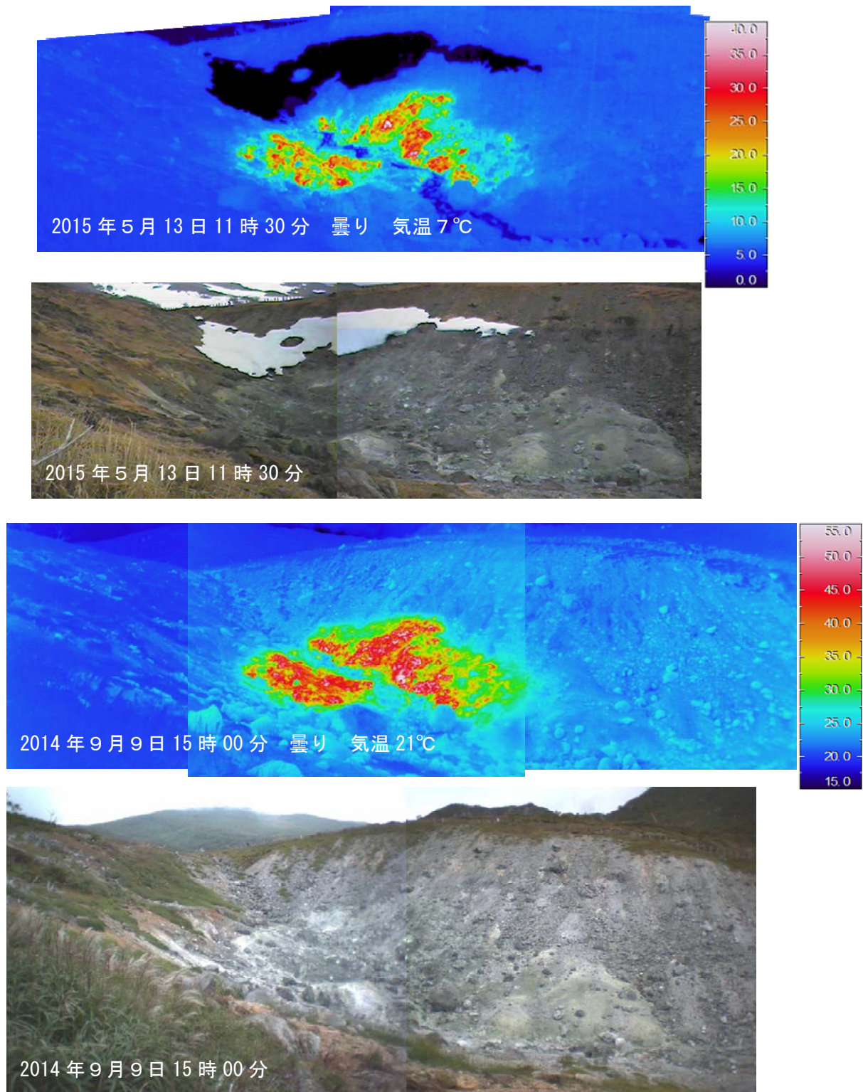
図5 栗駒山 北東から撮影したゼッタ沢上流の状況と地表面温度分布
