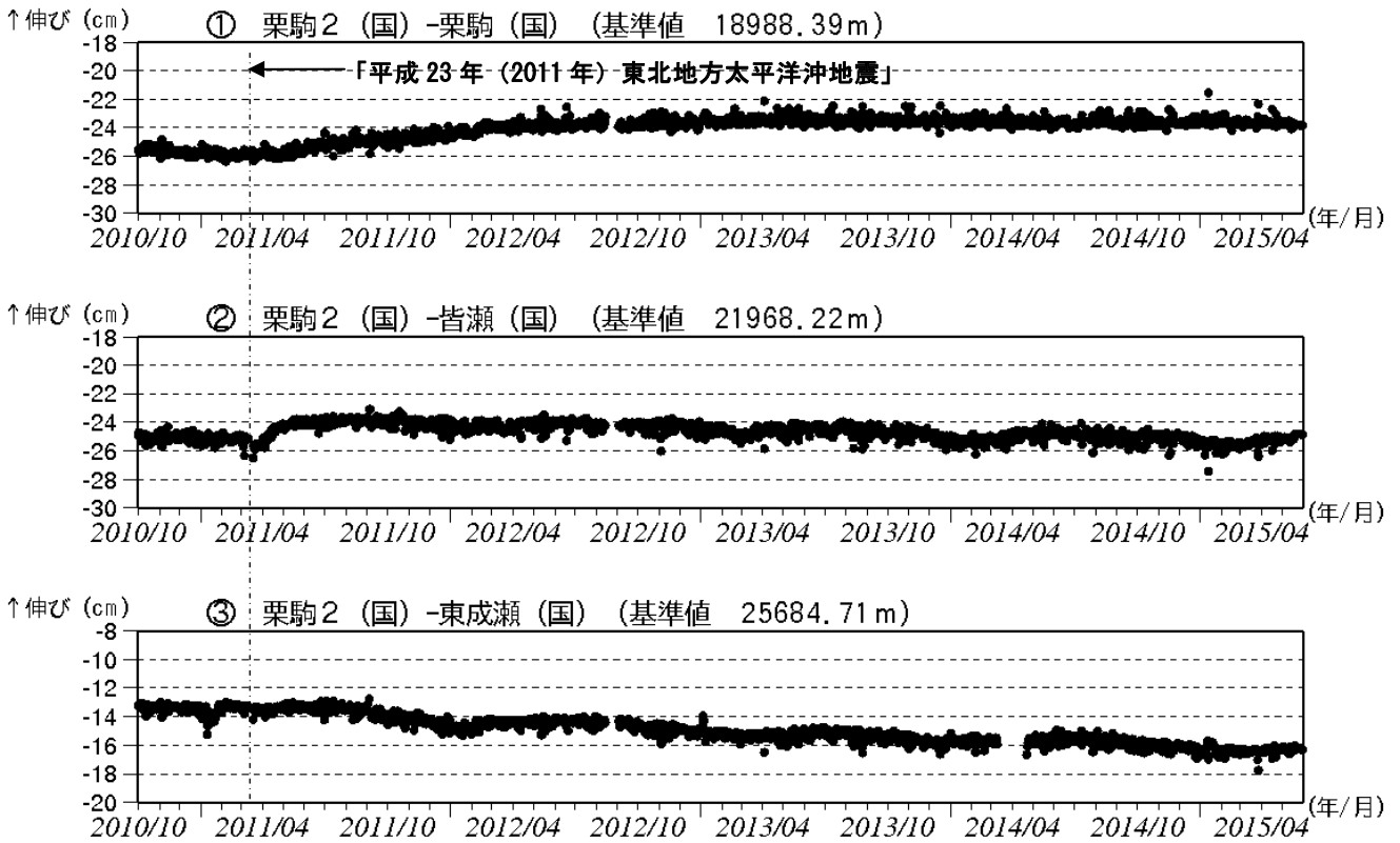
図 10 栗駒山 GNSS 2) 基線長変化図 (2010 年 10 月～2015 年 5 月)
