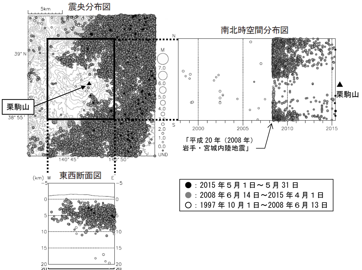
図 9 栗駒山 広域地震観測網による栗駒山周辺の地震活動（1997 年 10 月～2015 年 5 月）
