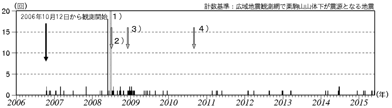
図 8 栗駒山 日別地震回数（2006 年 10 月～2015 年 5 月）
