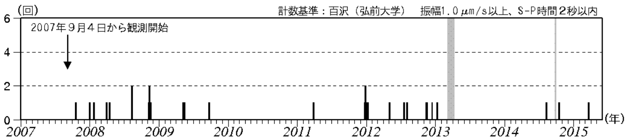
図2 岩木山 日別地震回数（2007年9月～2015年5月）
