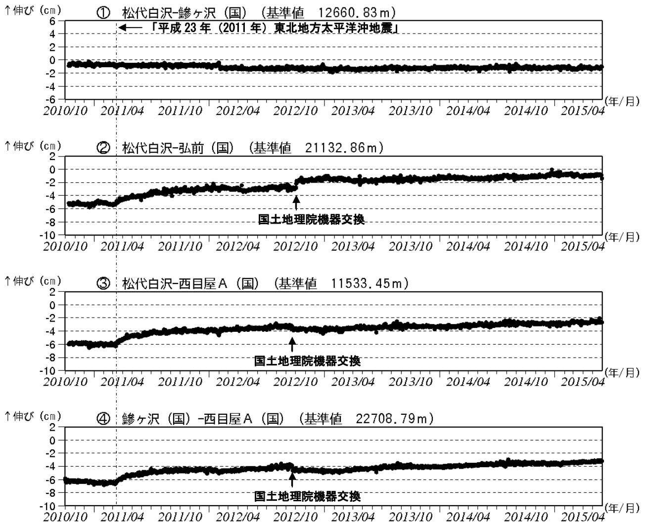
図3 岩木山 GNSS 1) 基線長変化図（2010年10月～2015年5月）
