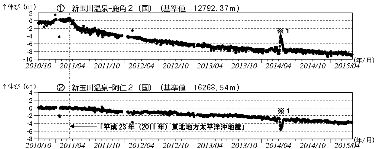
図3 秋田焼山 GNSS 1) 基線長変化図（2010年10月～2015年4月）
