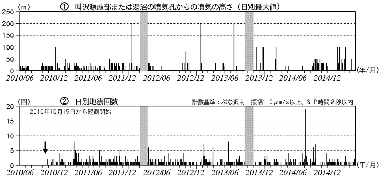
図2 秋田焼山 火山活動経過図（2010年6月～2015年4月）
