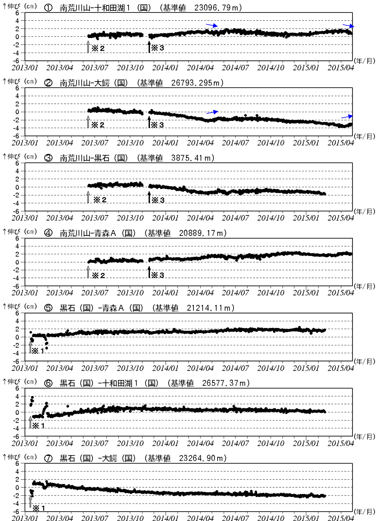
図5-① 八甲田山 GNSS 基線長変化図 (2013 年 1 月～2015 年 4 月)
