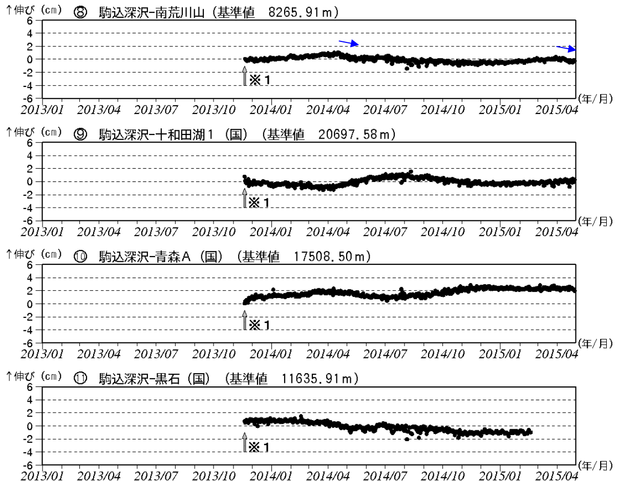
図5-② 八甲田山 GNSS 基線長変化図 (2013 年 1 月～2015 年 4 月)
