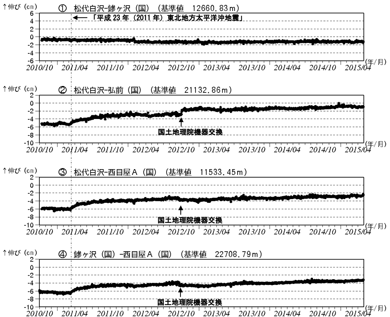
図3 岩木山 GNSS 1) 基線長変化図（2010年10月～2015年4月）
