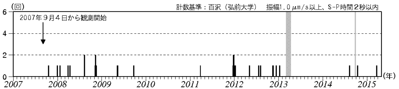
図2 岩木山 日別地震回数（2007年9月～2015年4月）
