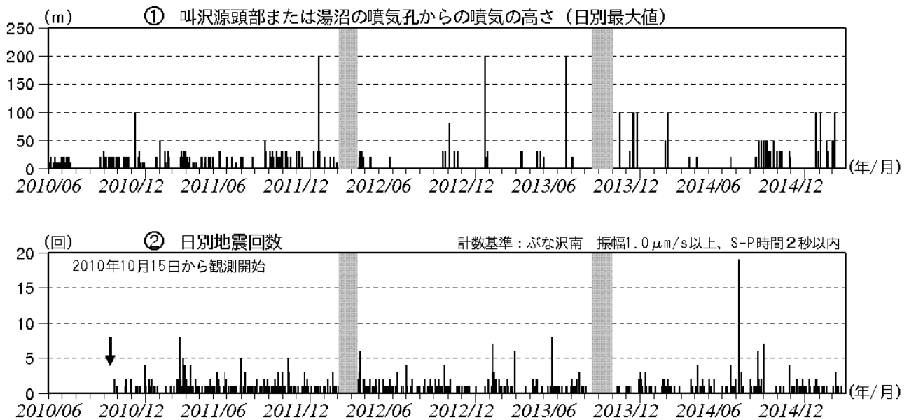
図 2 秋田焼山 火山活動経過図（2010 年 6 月～2015 年 3 月）
