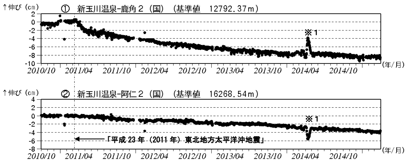
図 3 秋田焼山 GNSS 1) 基線長変化図（2010 年 10 月～2015 年 3 月）
