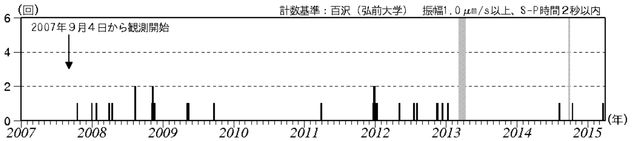
図2 岩木山 日別地震回数（2007年9月～2015年3月）
