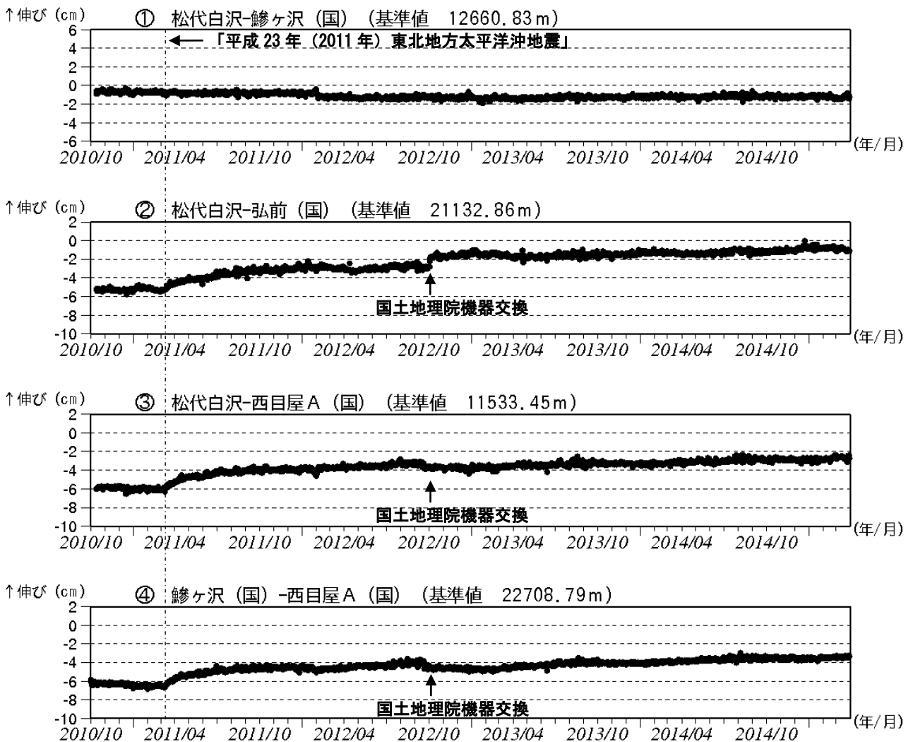
図3 岩木山 GNSS 1) 基線長変化図（2010年10月～2015年3月）
