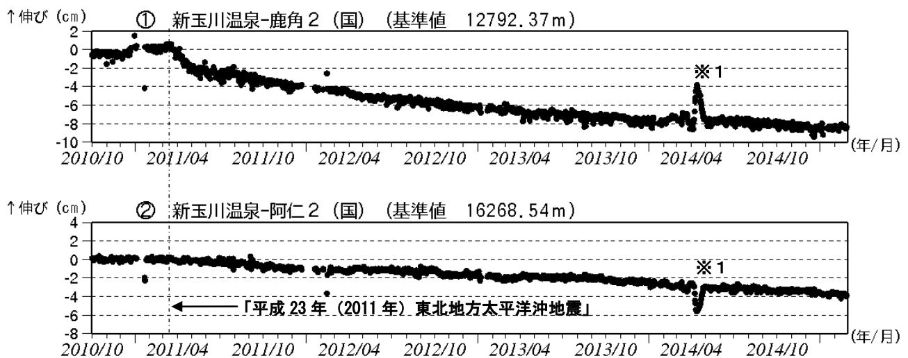
図3 秋田焼山 GNSS 1) 基線長変化図（2010年10月～2015年2月）
