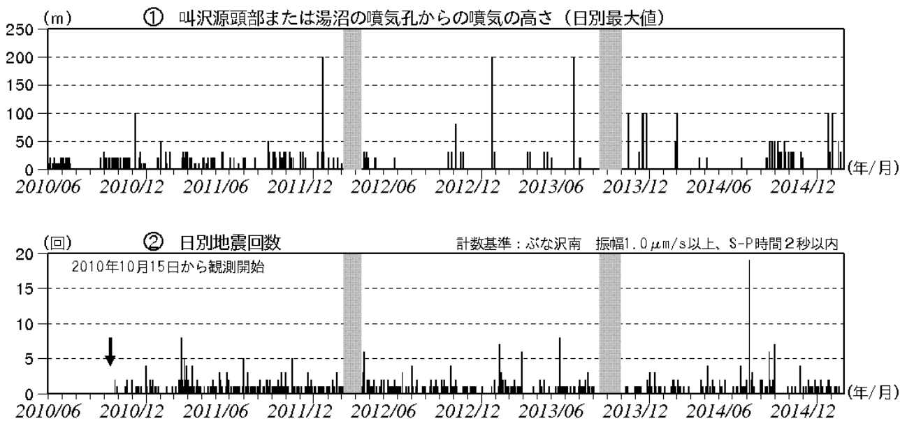
図2 秋田焼山 火山活動経過図（2010年6月～2015年2月）
