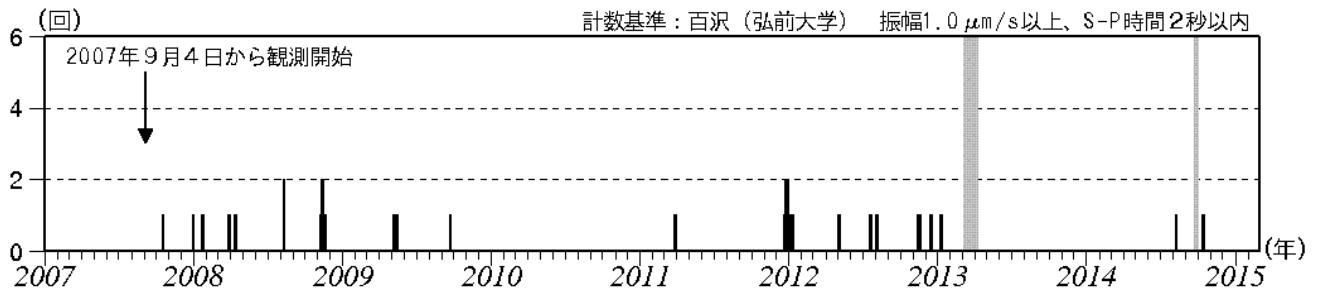
図 2 岩木山 日別地震回数（2007 年 9 月～2015 年 2 月）
