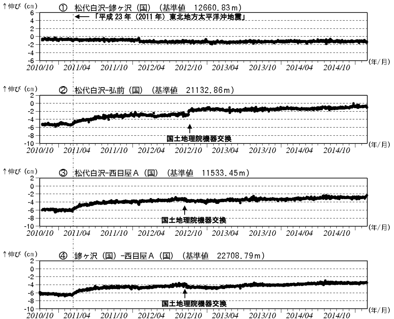
図 3 岩木山 GNSS 1) 基線長変化図（2010 年 10 月～2015 年 2 月）
