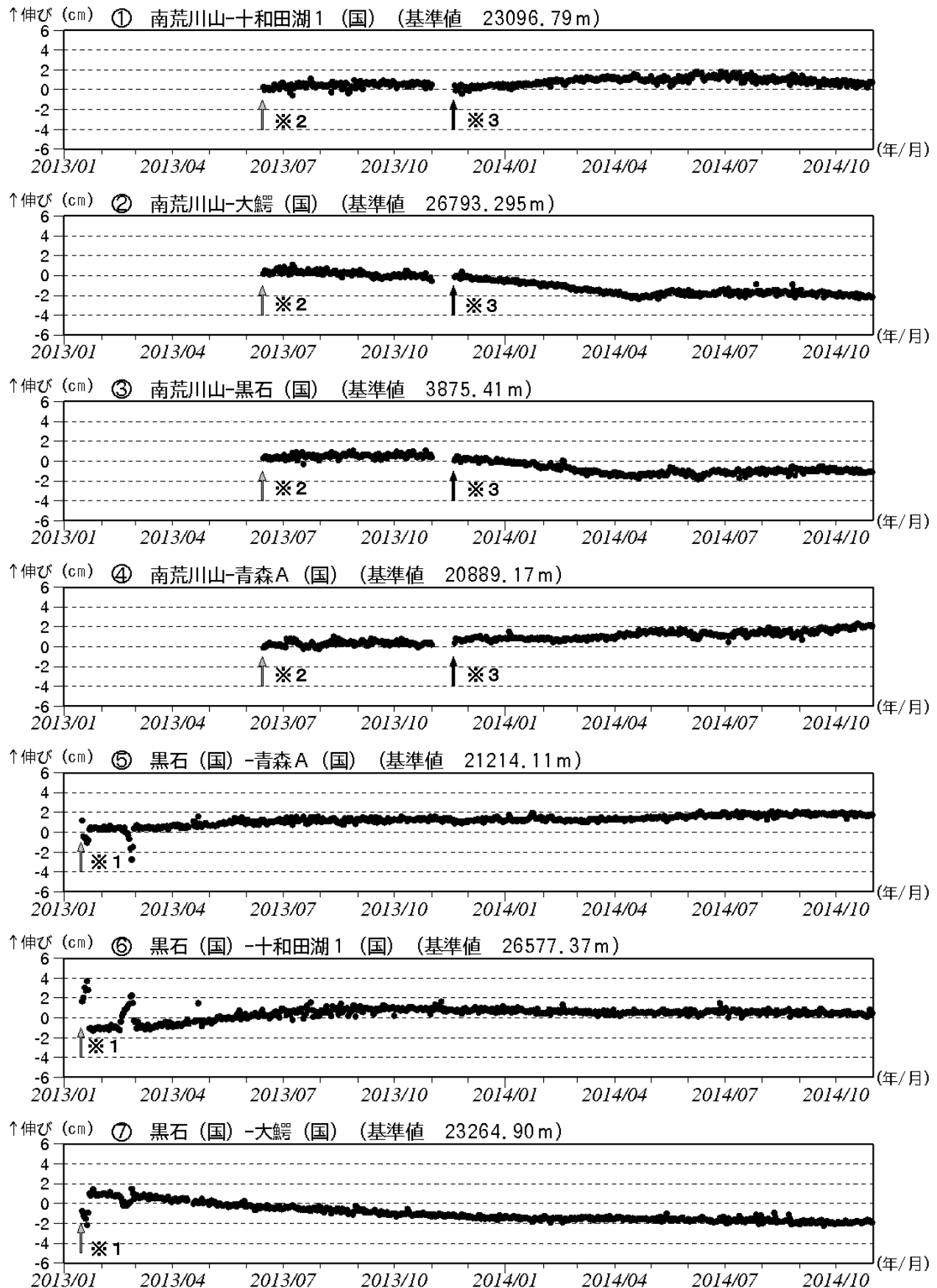
図5-① 八甲田山 GNSS 基線長変化図 (2013 年 1 月～2014 年 10 月)
