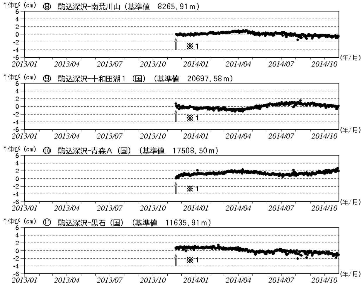
図 5-② 八甲田山 GNSS 基線長変化図 (2013 年 1 月～2014 年 10 月)
