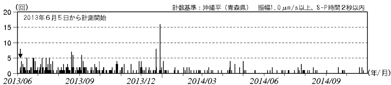
図2 八甲田山 日別地震回数 (2013年6月~2014年10月)
