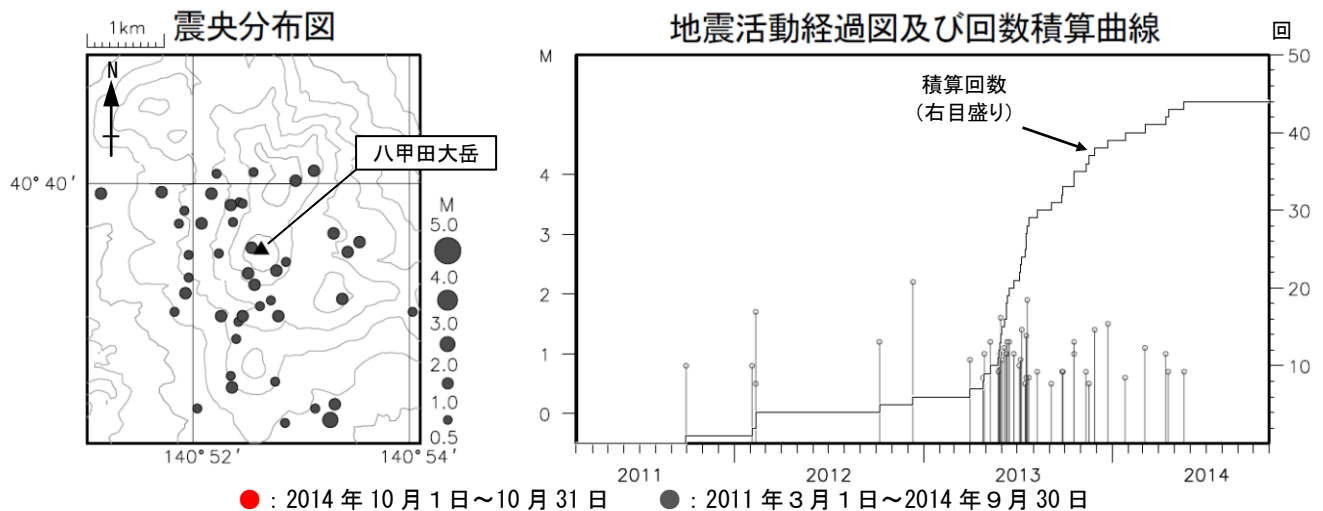
図 4 八甲田山 広域地震観測網による八甲田大岳山頂付近の地震活動図（2011 年 3 月～2014 年 10 月）
