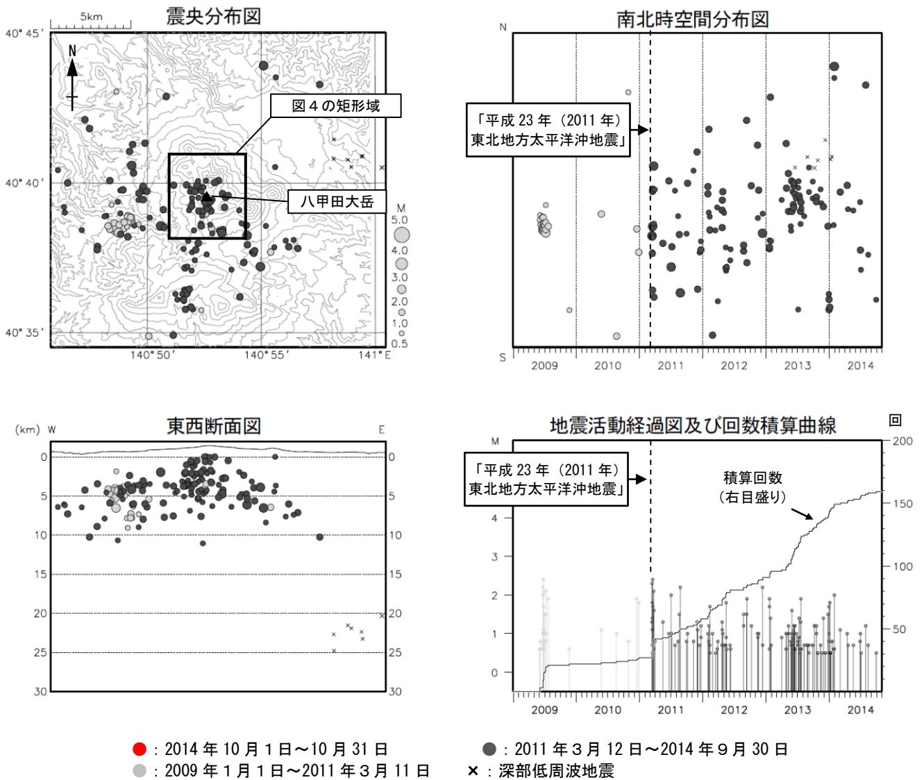
図 3 八甲田山 広域地震観測網による八甲田山周辺の地震活動図（2009 年 1 月～2014 年 10 月）
