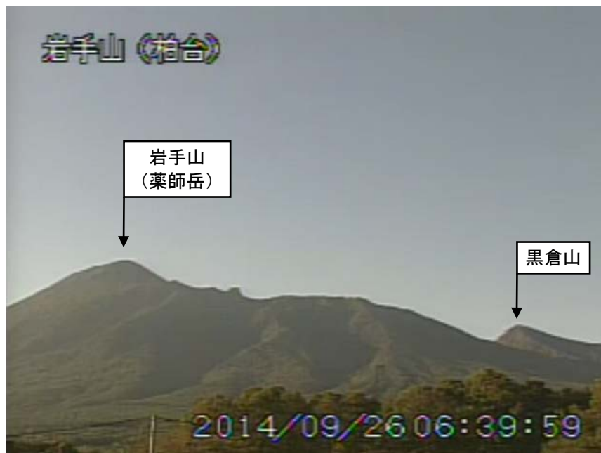
図 1 岩手山 東岩手火山と西岩手火山の状況（9 月 26 日）
