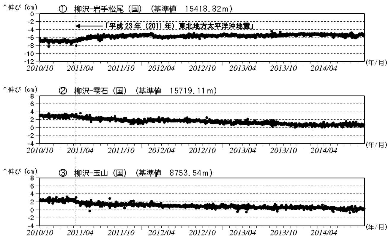
図 4 岩手山 GNSS 基線長変化図 (2010 年 10 月～2014 年 9 月)
