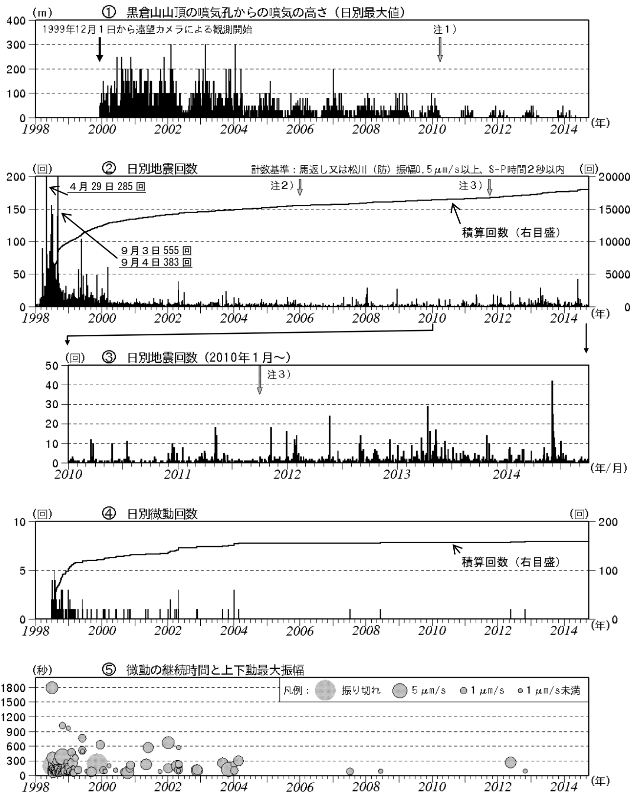
図2 岩手山 火山活動経過図（1998年1月～2014年9月）
