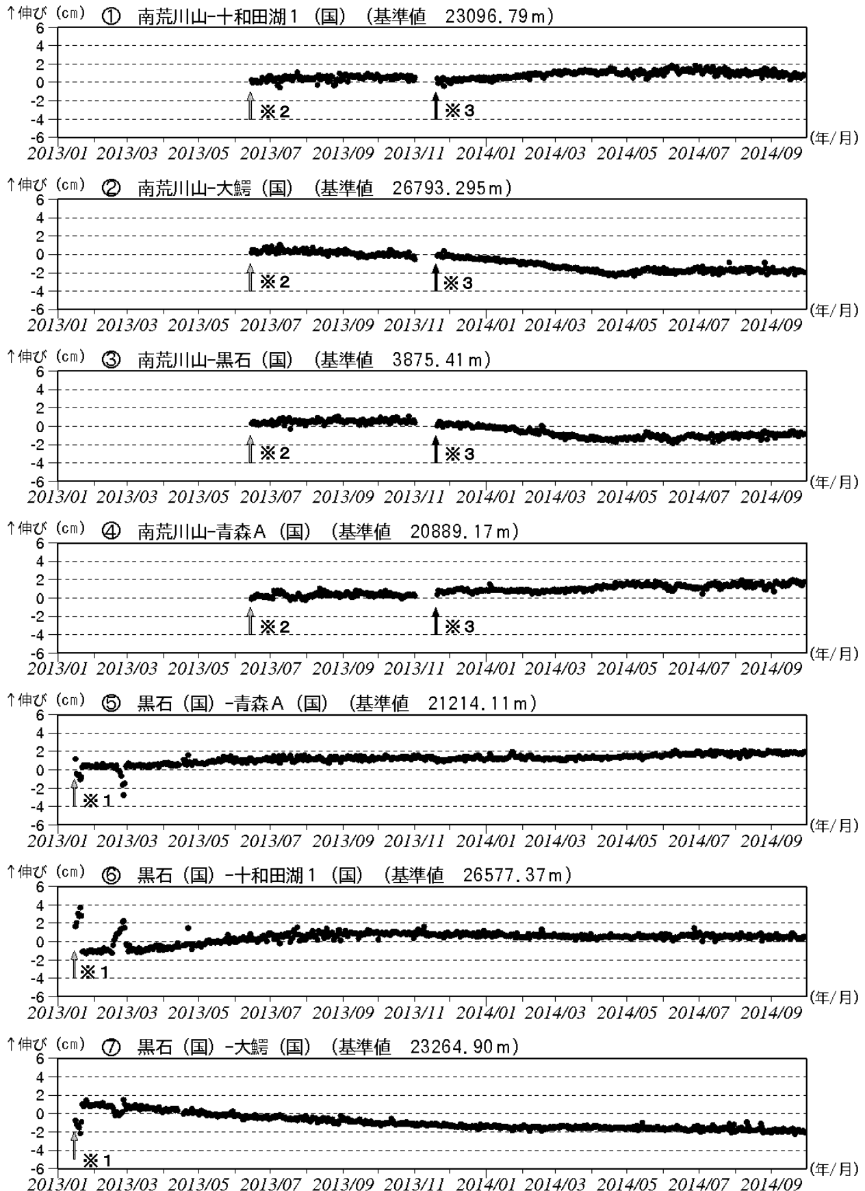
図 5-1 八甲田山 GNSS 基線長変化図 (2013 年 1 月～2014 年 9 月)
