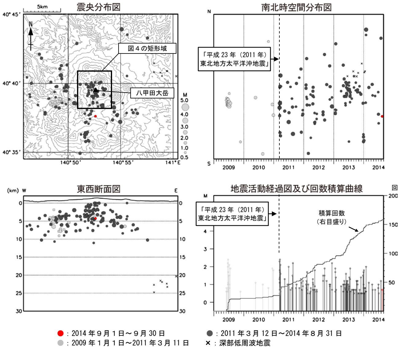
図 3 八甲田山 広域地震観測網による八甲田山周辺の地震活動図（2009 年 1 月～2014 年 9 月）
