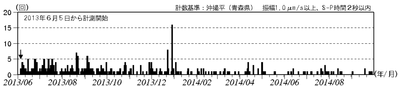
図2 八甲田山 日別地震回数 (2013年6月~2014年9月)
