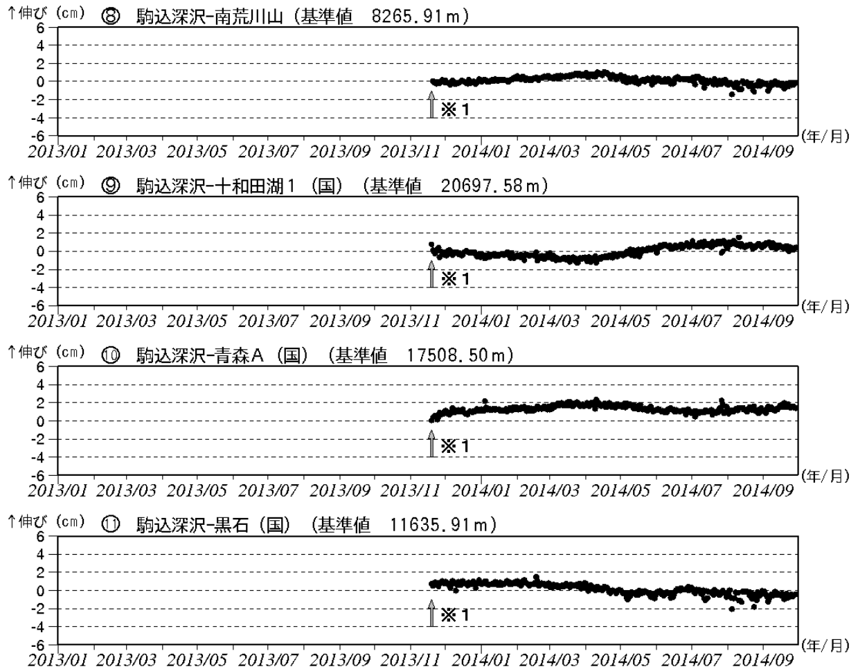
図 5-2 八甲田山 GNSS 基線長変化図 (2013 年 1 月～2014 年 9 月)
