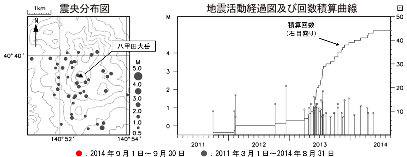
図 4 八甲田山 広域地震観測網による八甲田大岳山頂付近の地震活動図（2011 年 3 月～2014 年 9 月）
