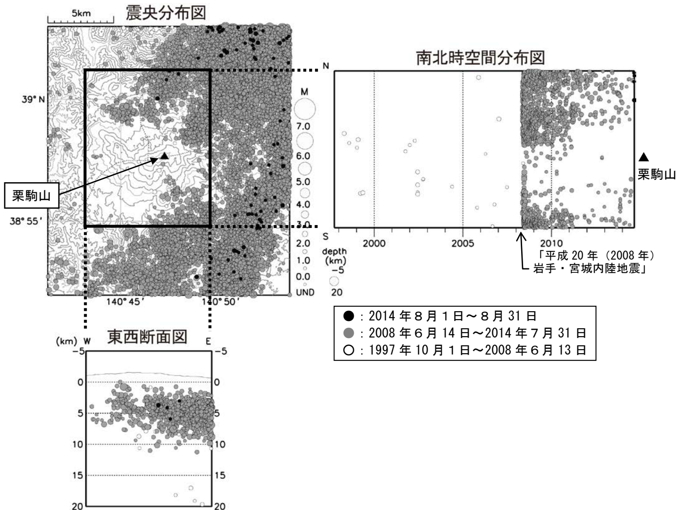
図4 栗駒山 広域地震観測網による栗駒山周辺の地震活動（1997年10月～2014年8月）
