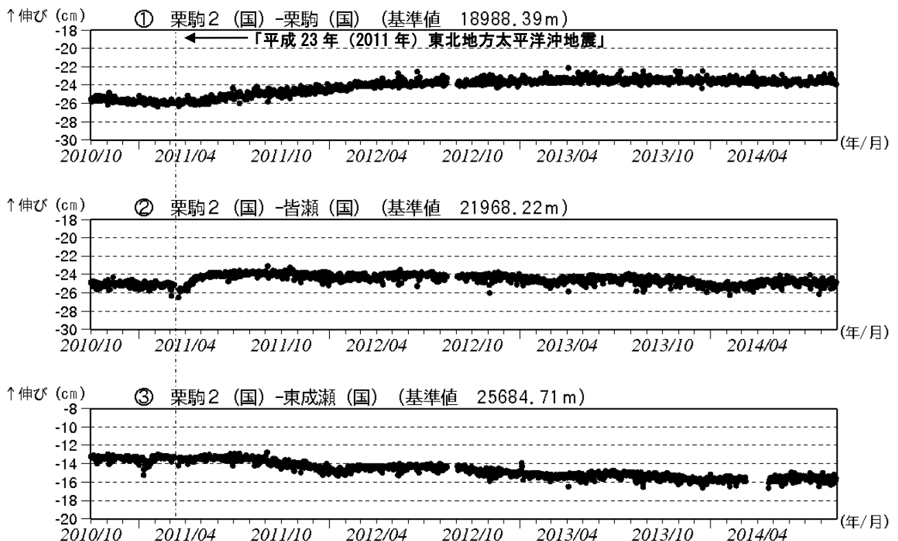
図6 栗駒山 GNSS 基線長変化図 (2010 年 10 月～2014 年 8 月)
