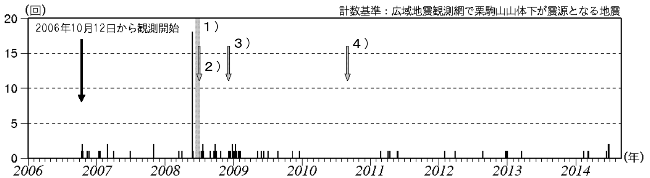
図3 栗駒山 日別地震回数（2006年10月～2014年8月）
