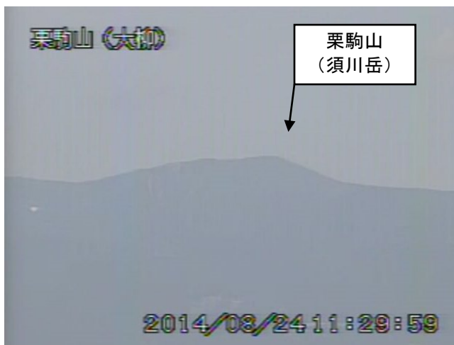
図 1 栗駒山 山頂周辺の状況（8 月 24 日）
