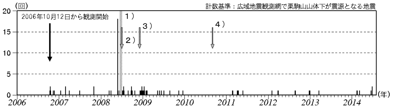
図3 栗駒山 日別地震回数（2006年10月～2014年7月）
