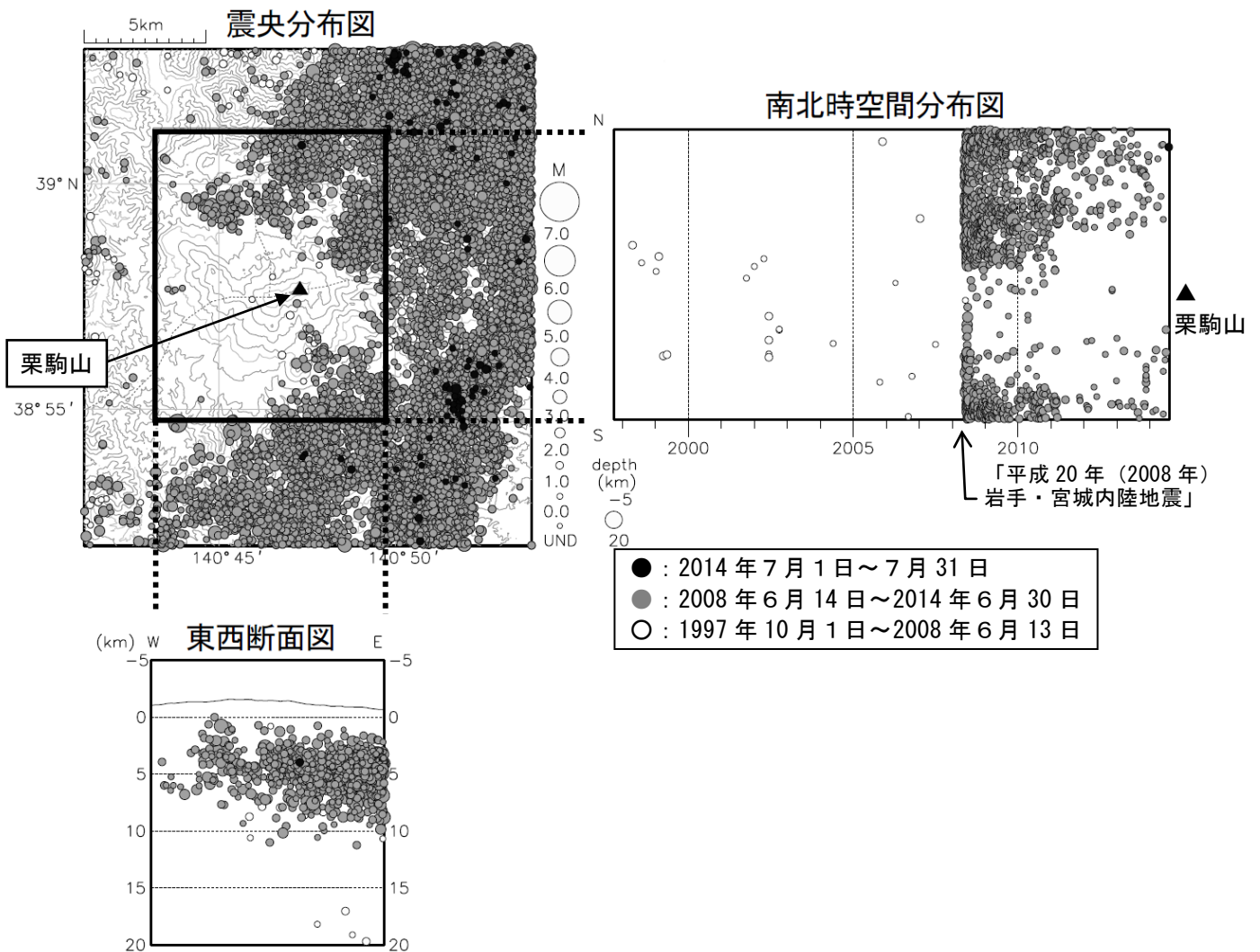
図4 栗駒山 広域地震観測網による栗駒山周辺の地震活動（1997年10月～2014年7月）
