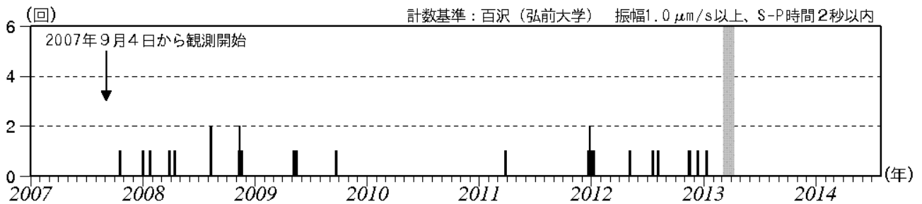
図2 岩木山 日別地震回数（2007年9月～2014年7月）
