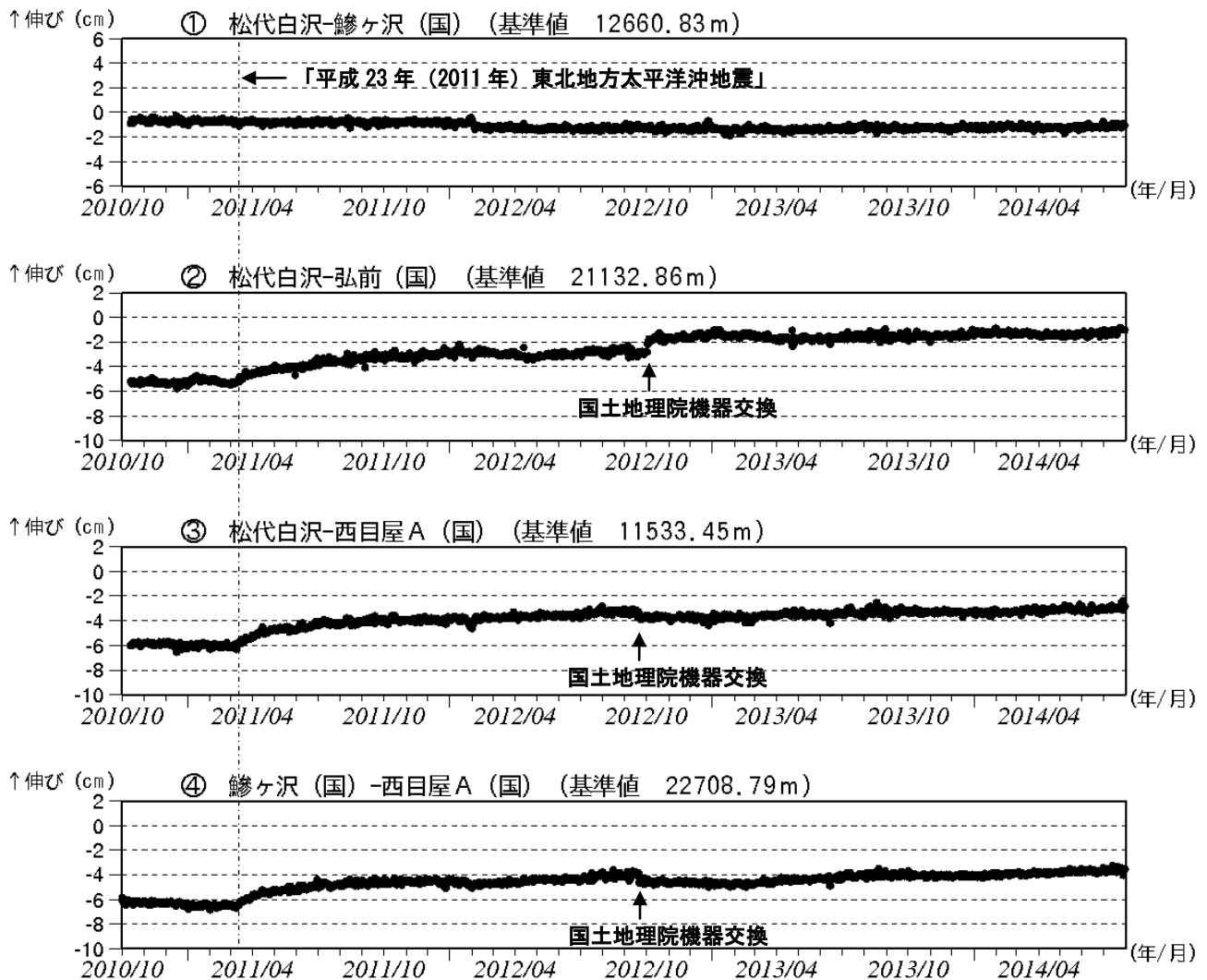
図3 岩木山 GNSS 1) 基線長変化図（2010年10月～2014年7月）
