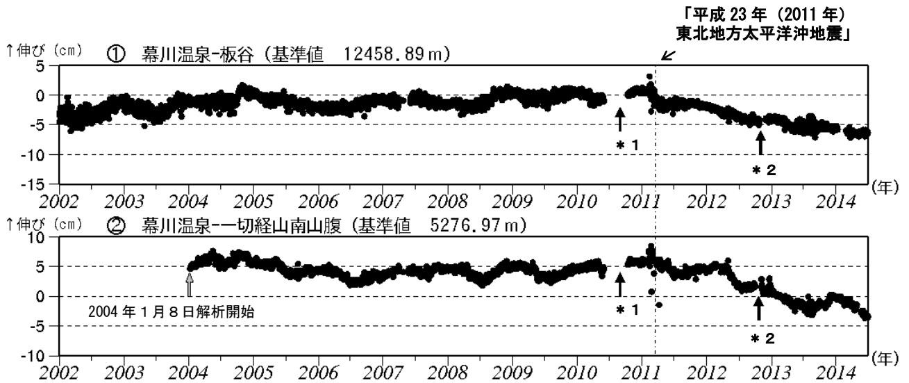
図4-① 吾妻山 GNSS 基線長変化図 (2002年1月～2014年6月)
