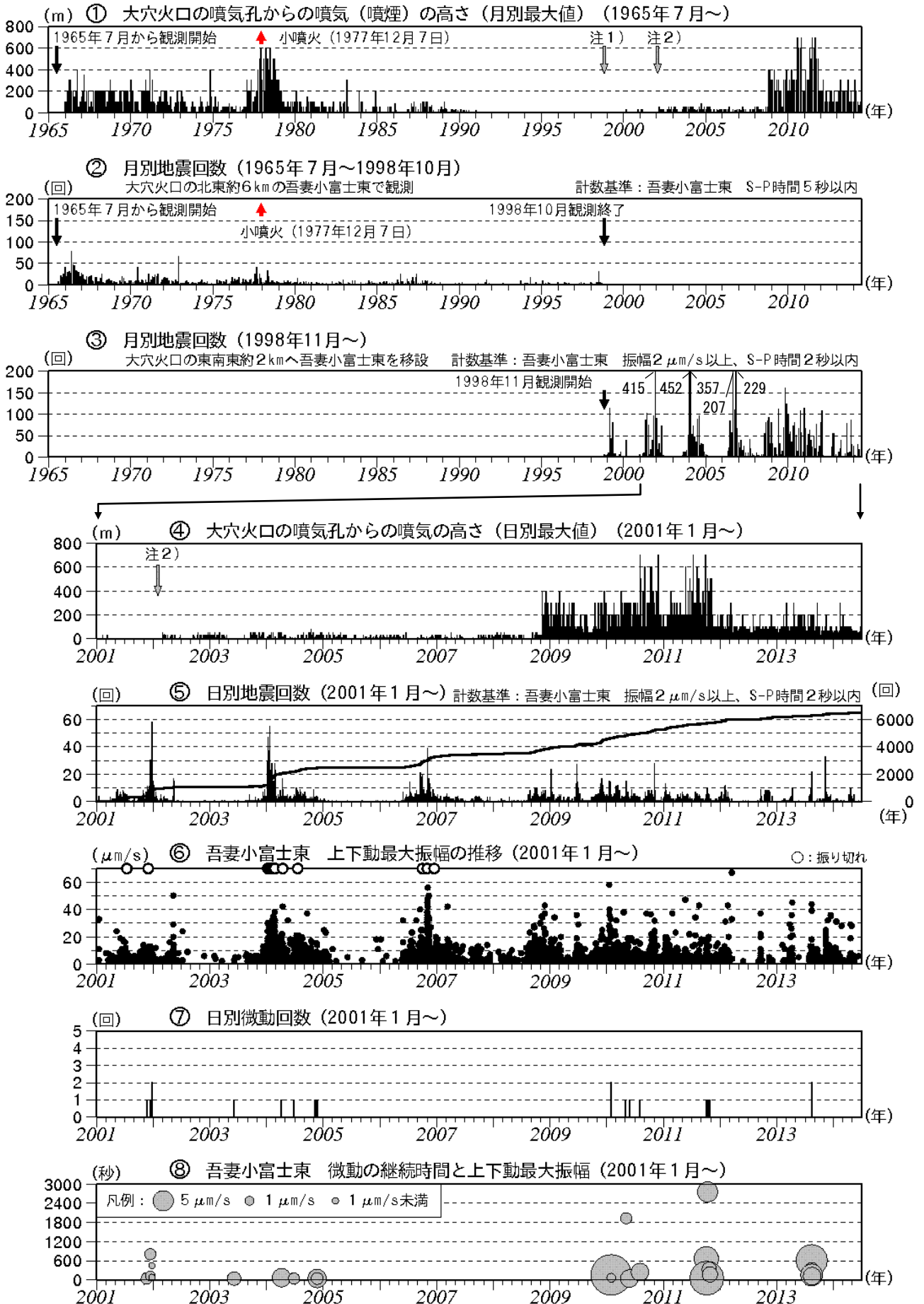
図2 吾妻山 火山活動経過図 (1965年7月～2014年6月)
