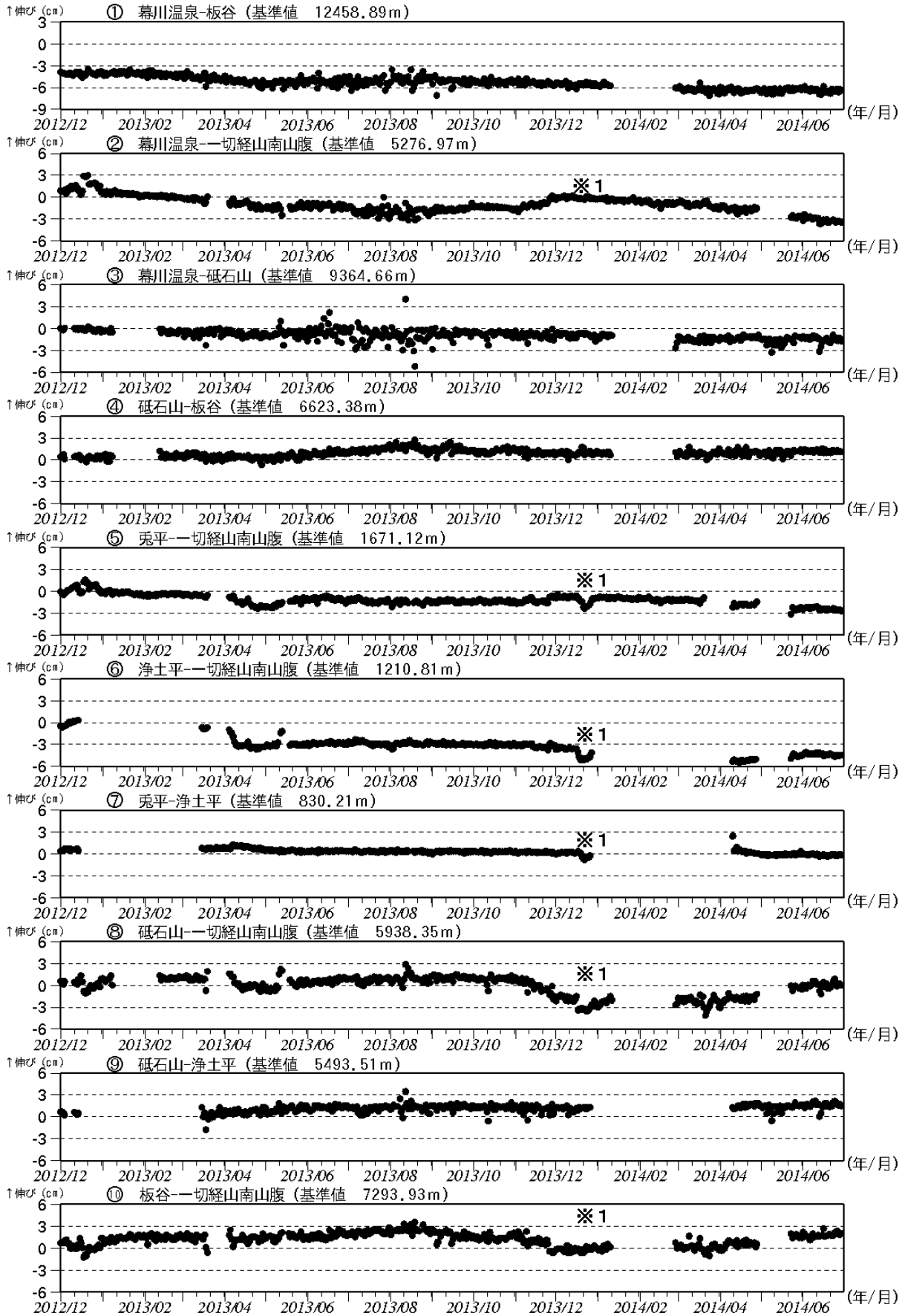
図 4-② 吾妻山 GNSS 基線長変化図 (2012 年 12 月～2014 年 6 月)
