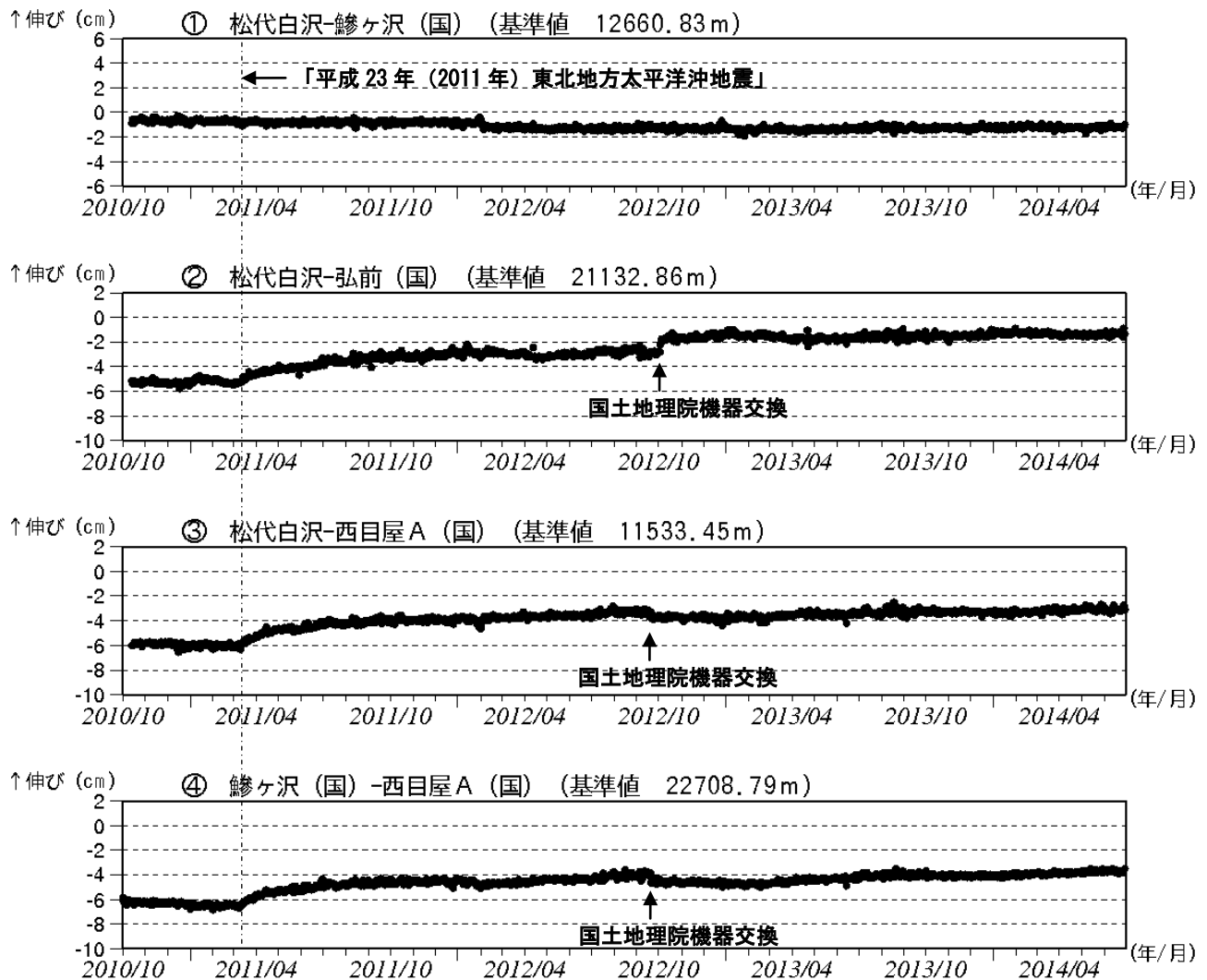
図3 岩木山 GNSS 1) 基線長変化図（2010年10月～2014年6月）
