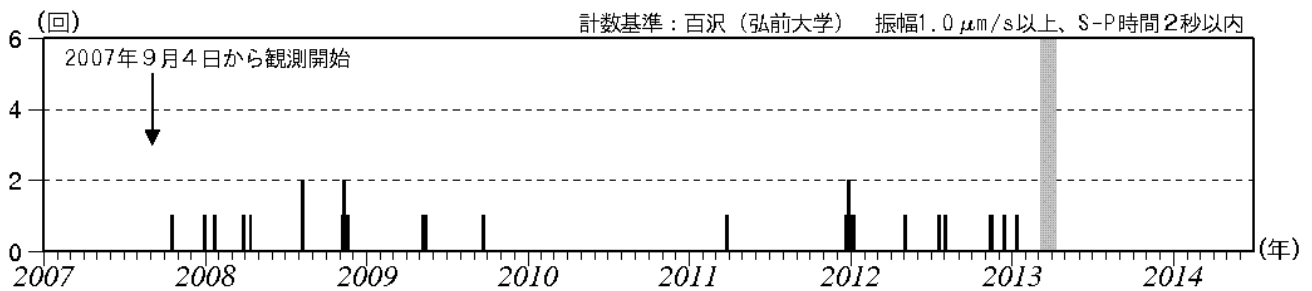
図2 岩木山 日別地震回数（2007年9月～2014年6月）
