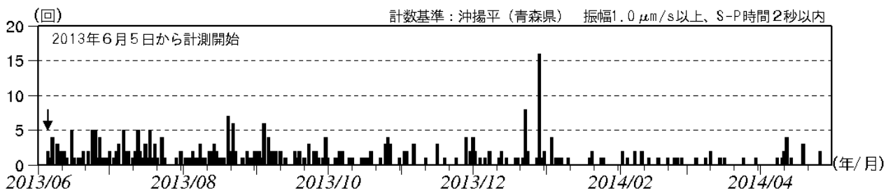
図 2 八甲田山 日別地震回数（2013 年 6 月～2014 年 4 月）
