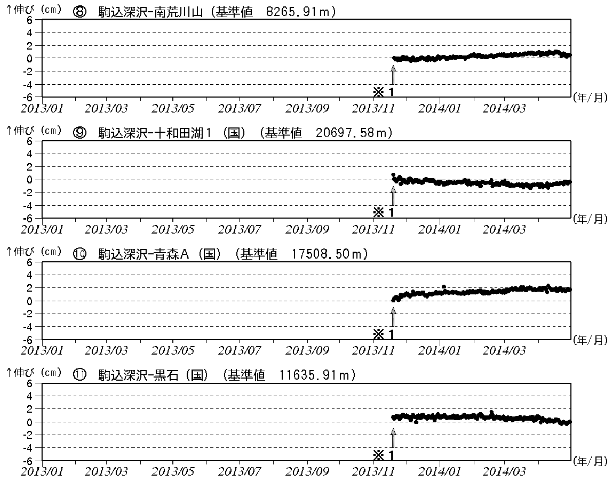
図5-2 八甲田山 GNSS 基線長変化図 (2013 年 1 月～2014 年 4 月)
