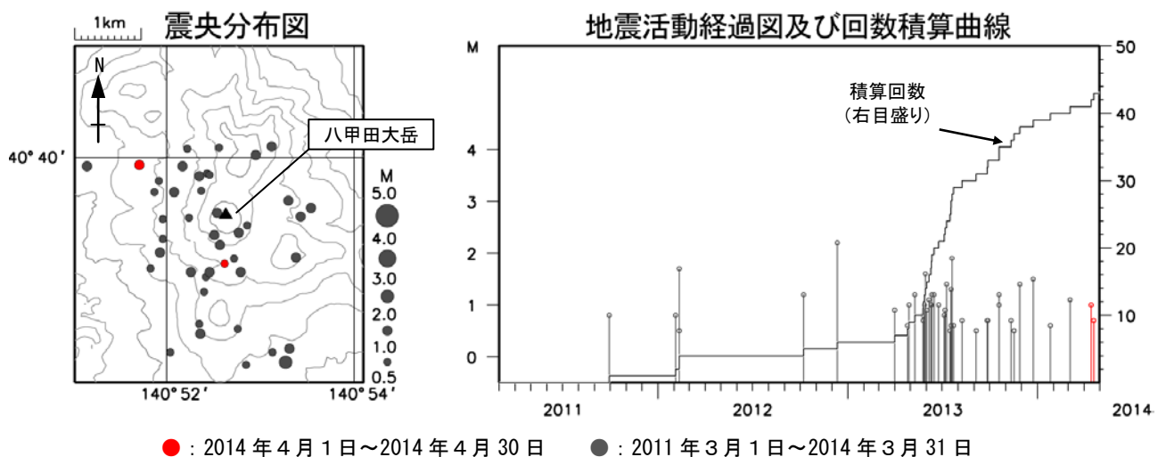
図 4 八甲田山 広域地震観測網による八甲田大岳山頂付近の地震活動図 （2011 年 3 月～2014 年 4 月）
