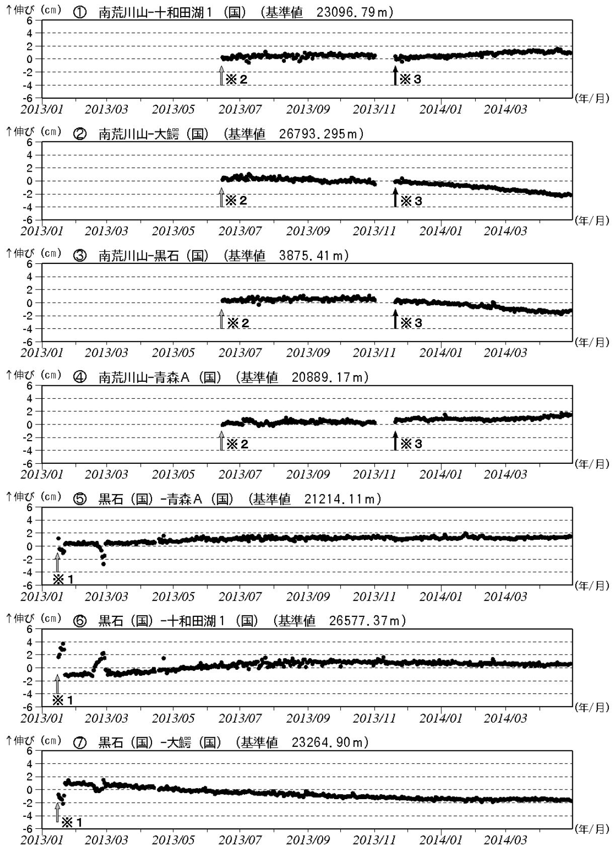
図5-1 八甲田山 GNSS 基線長変化図 (2013 年 1 月～2014 年 4 月)
