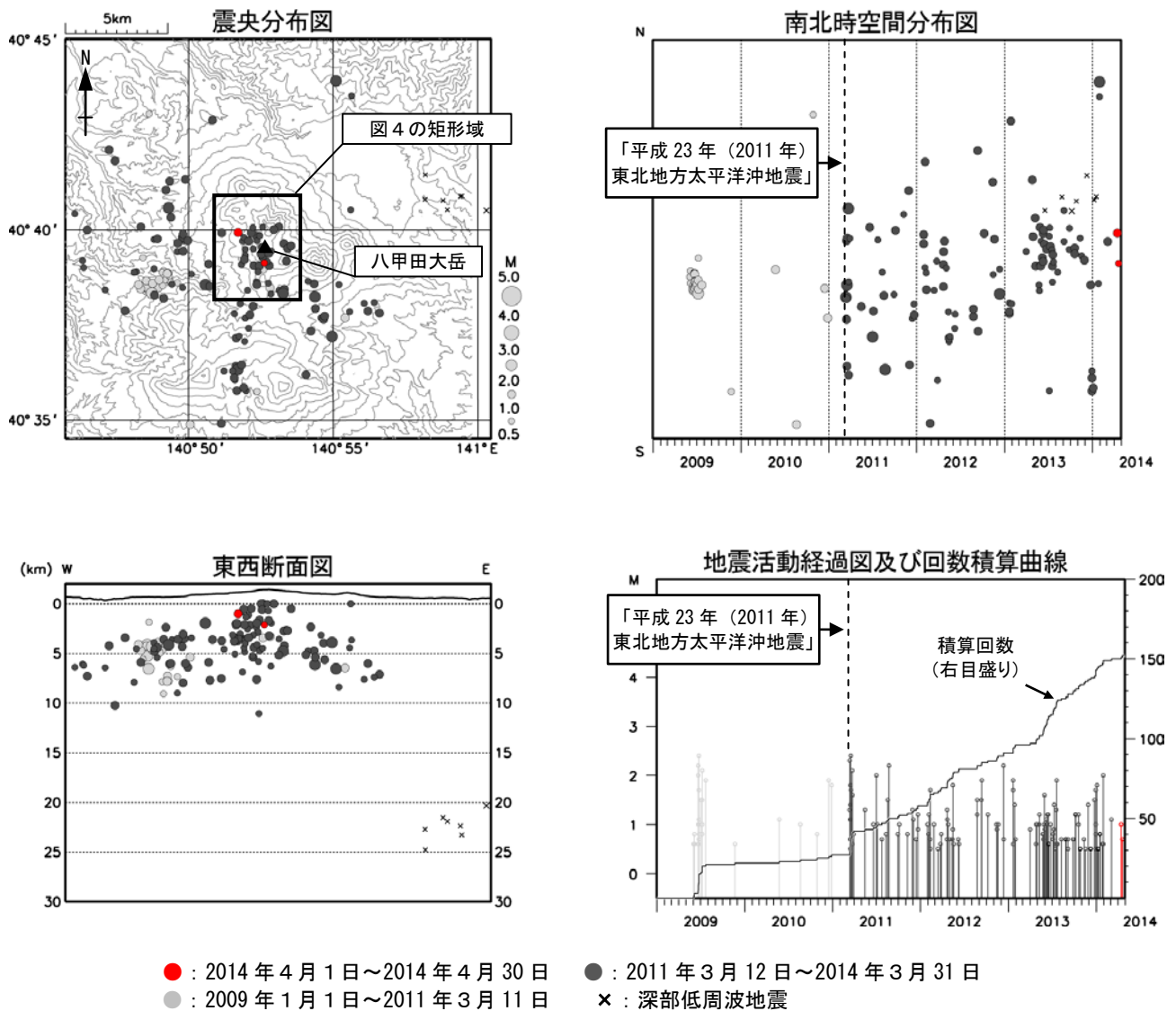
図 3 八甲田山 広域地震観測網による八甲田山周辺の地震活動図（2009 年 1 月～2014 年 4 月） 沖揚平観測点（青森県）が 2013 年 2 月 14 日～5 月 24 日まで障害のため検知能力が低下しています。
