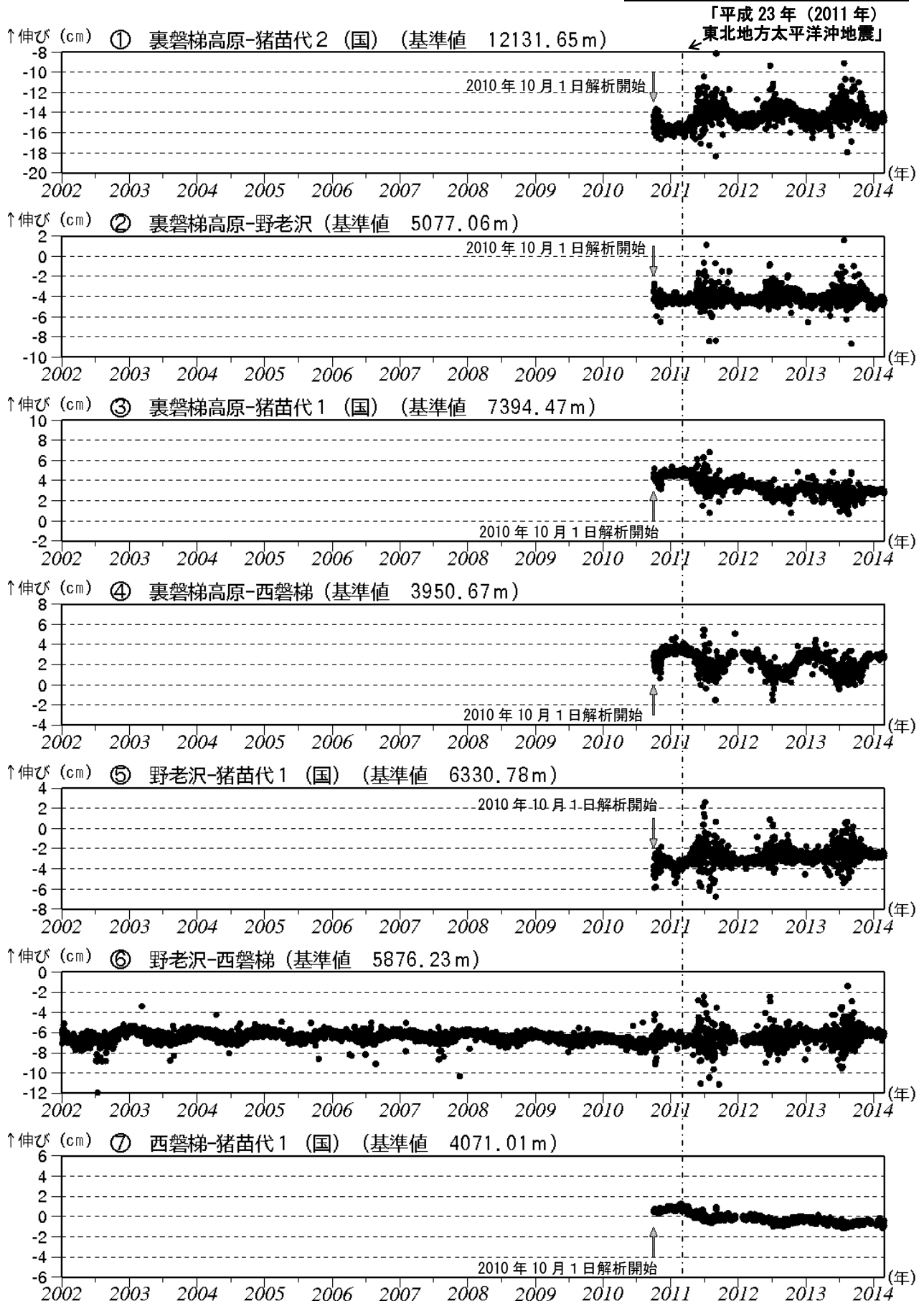
図3 磐梯山 GNSS 基線長変化図 (2002 年 1 月～2014 年 2 月)
