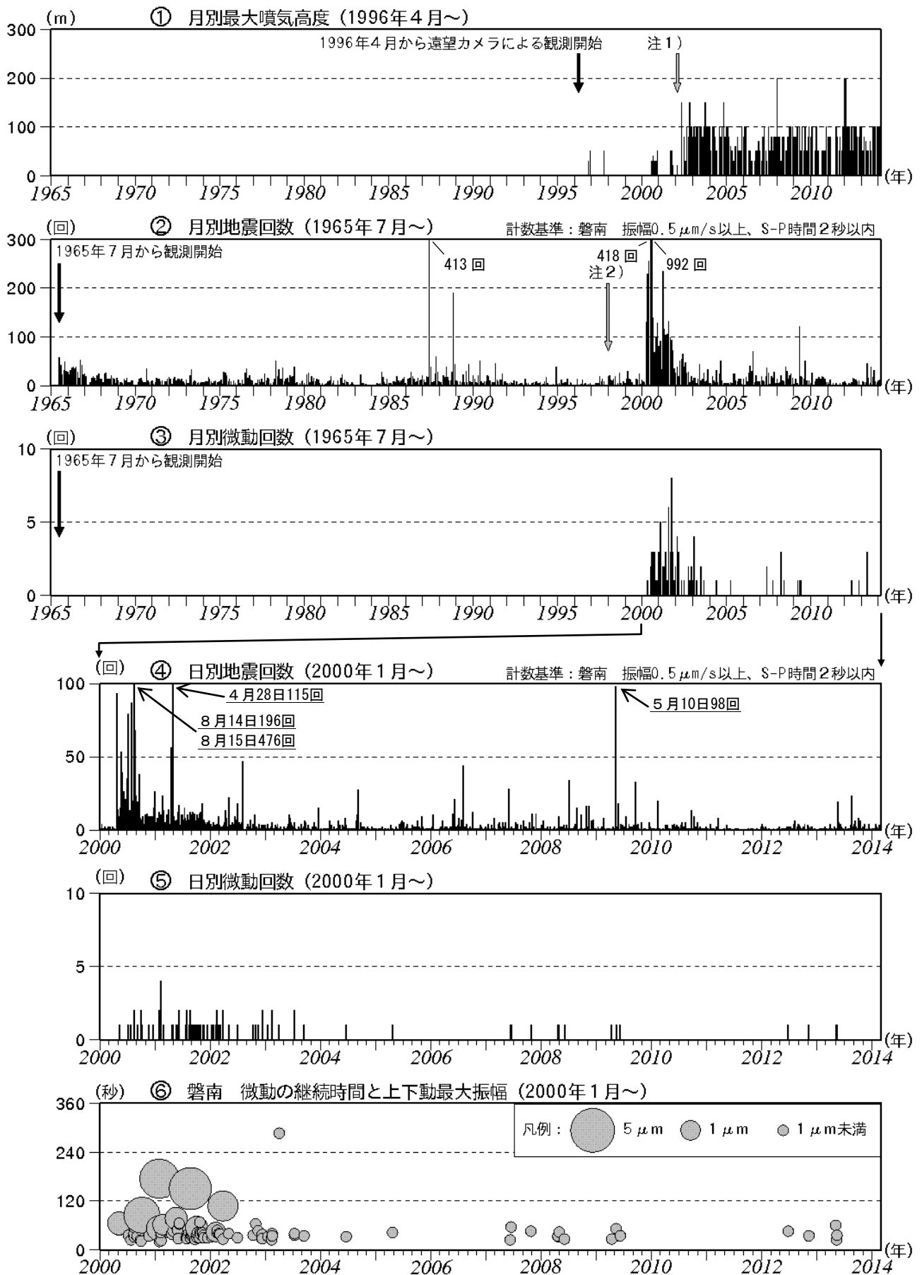
図2 磐梯山 火山活動経過図 (1965年7月～2014年2月)
