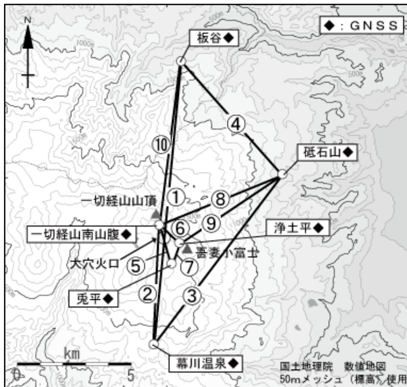
図3 吾妻山 GNSS 観測点配置図
