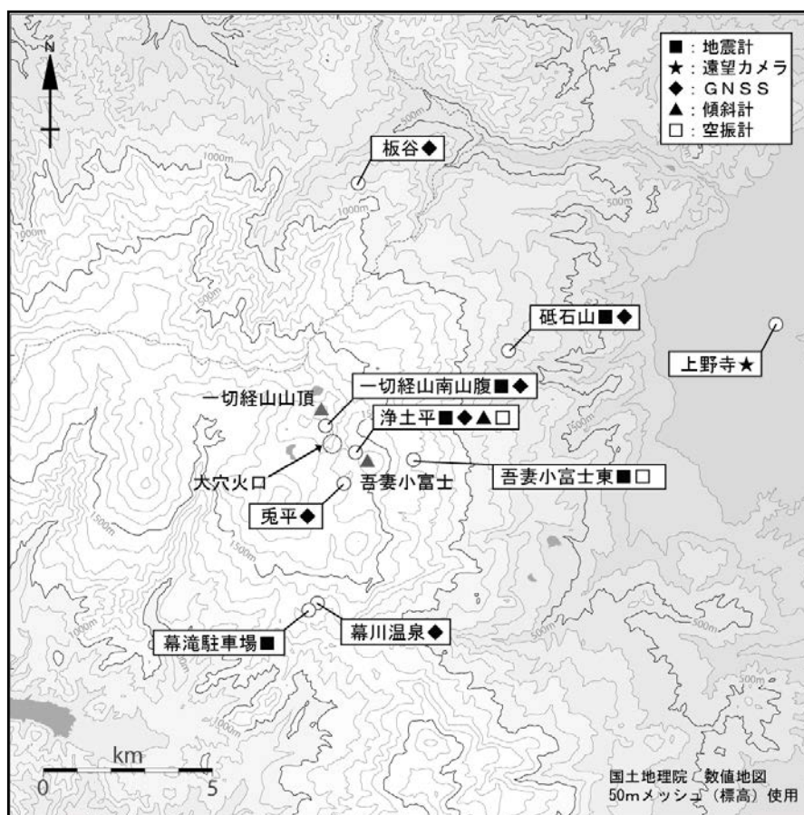
図6 吾妻山 観測点配置図
