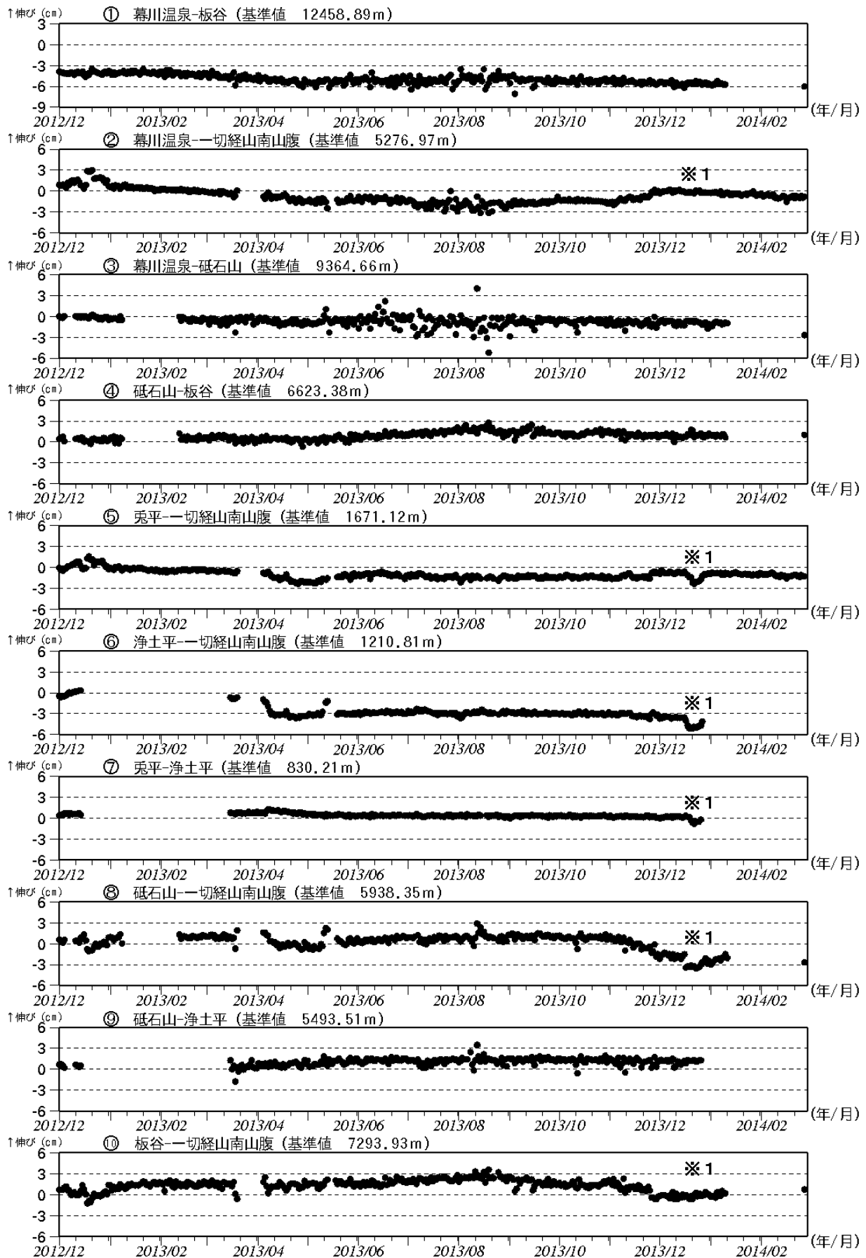
図5 吾妻山 GNSS 基線長変化図（2012 年 12 月～2014 年 2 月）
