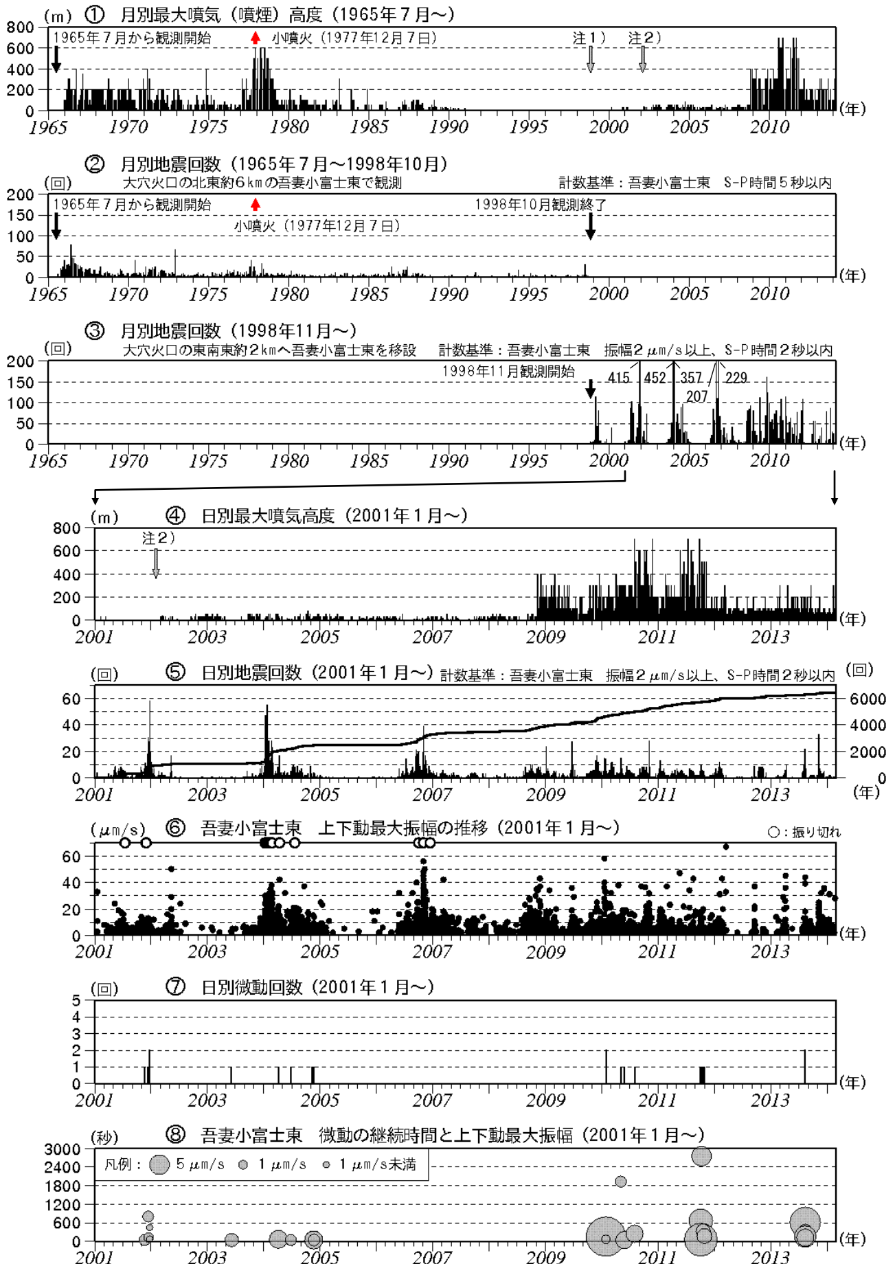
図2 吾妻山 火山活動経過図（1965年7月～2014年2月）
