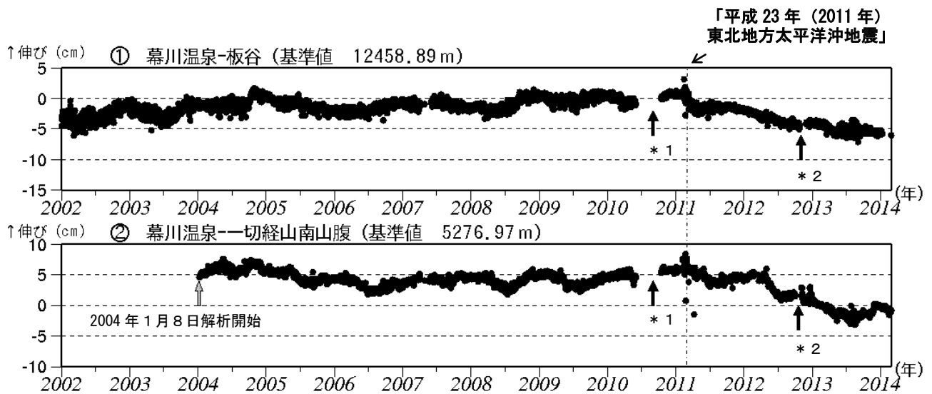
図4 吾妻山 GNSS 基線長変化図（2002 年 1 月～2014 年 2 月）
