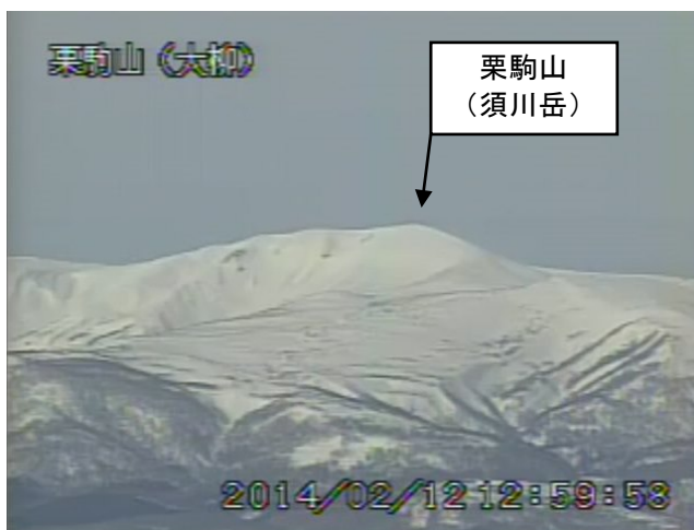
図 1 栗駒山 山頂周辺の状況 （2 月 12 日 13 時 00 分頃）
