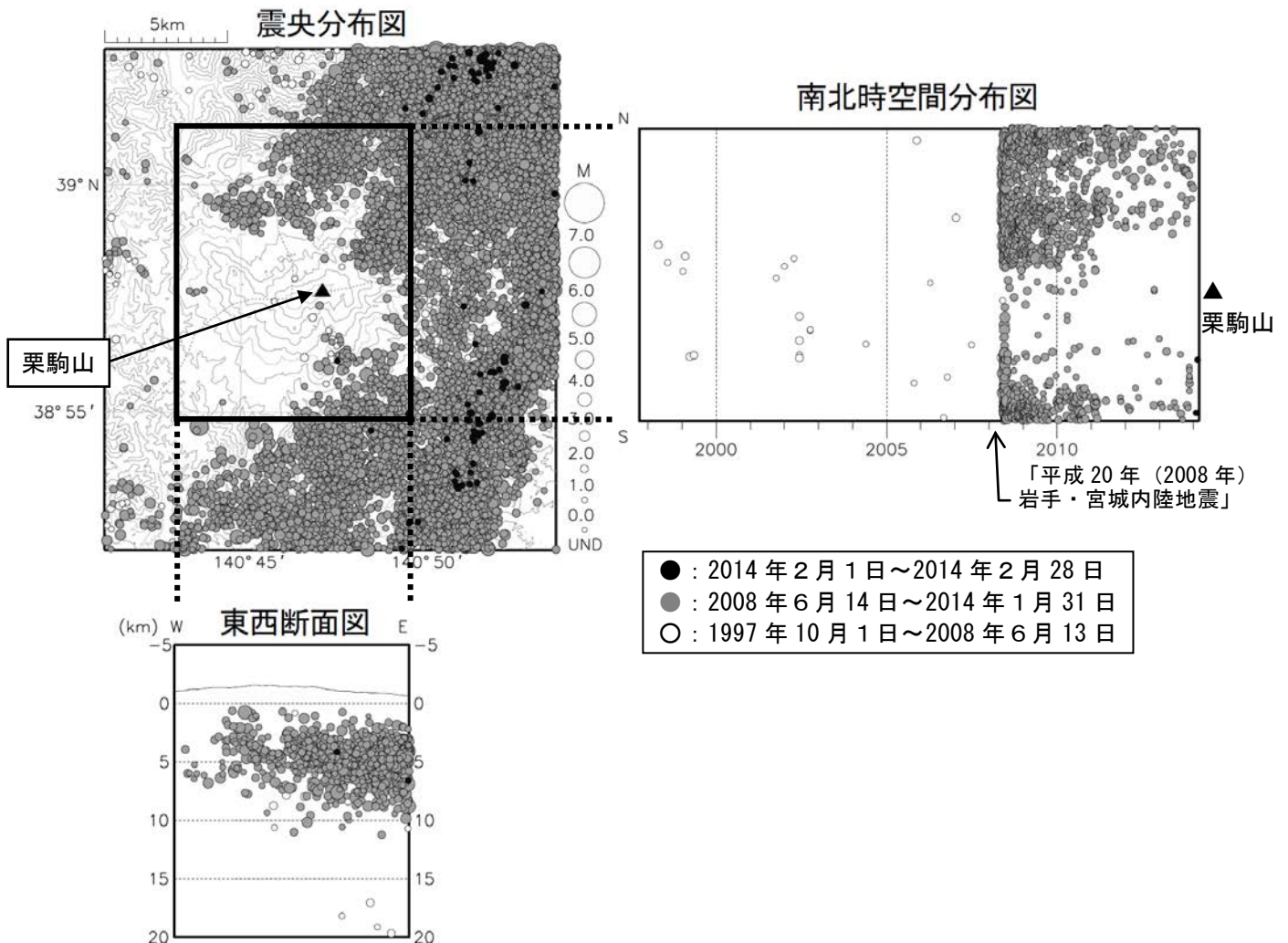
図4 栗駒山 広域地震観測網による栗駒山周辺の地震活動（1997年10月～2014年2月）
