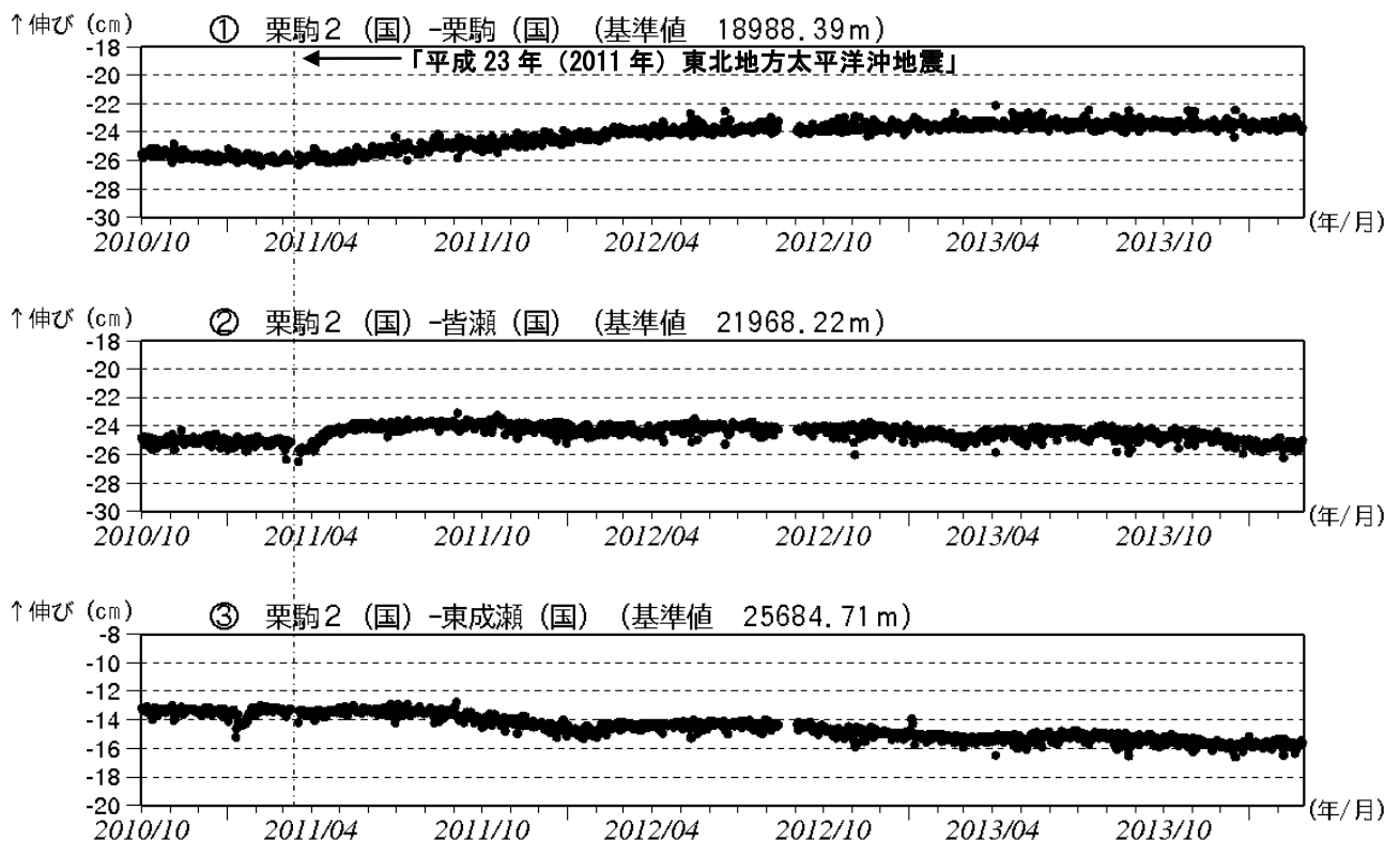
図6 栗駒山 GNSS 基線長変化図 (2010 年 10 月～2014 年 2 月)
