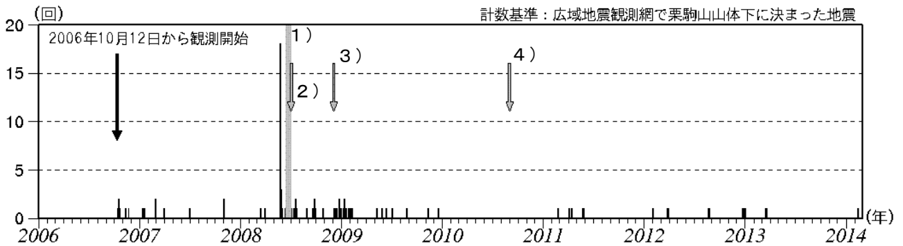
図3 栗駒山 日別地震回数（2006年10月～2014年2月）
