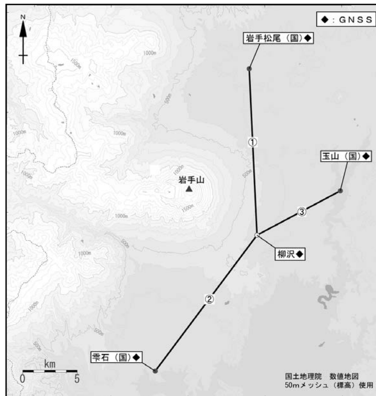
図3 岩手山 GNSS 観測点配置図
