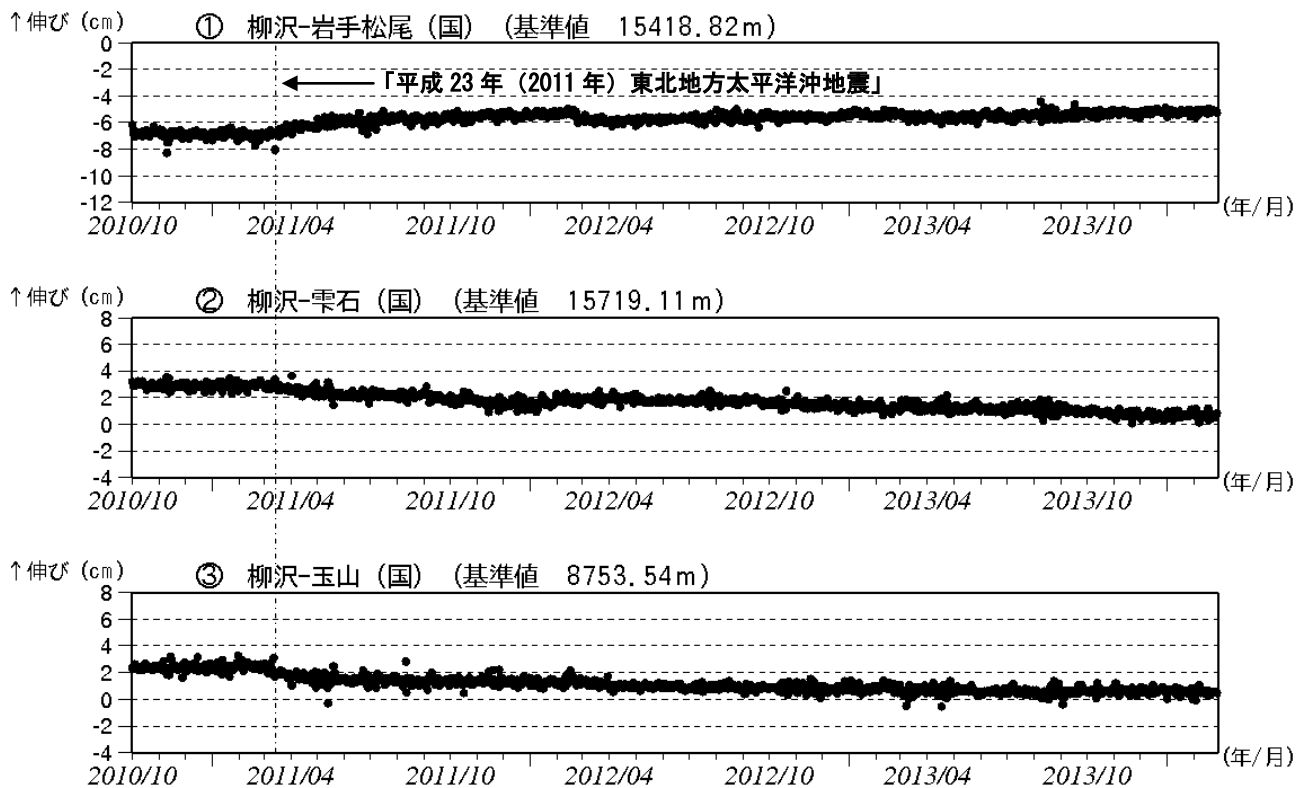
図4 岩手山 GNSS 基線長変化図（2010年10月～2014年2月）
