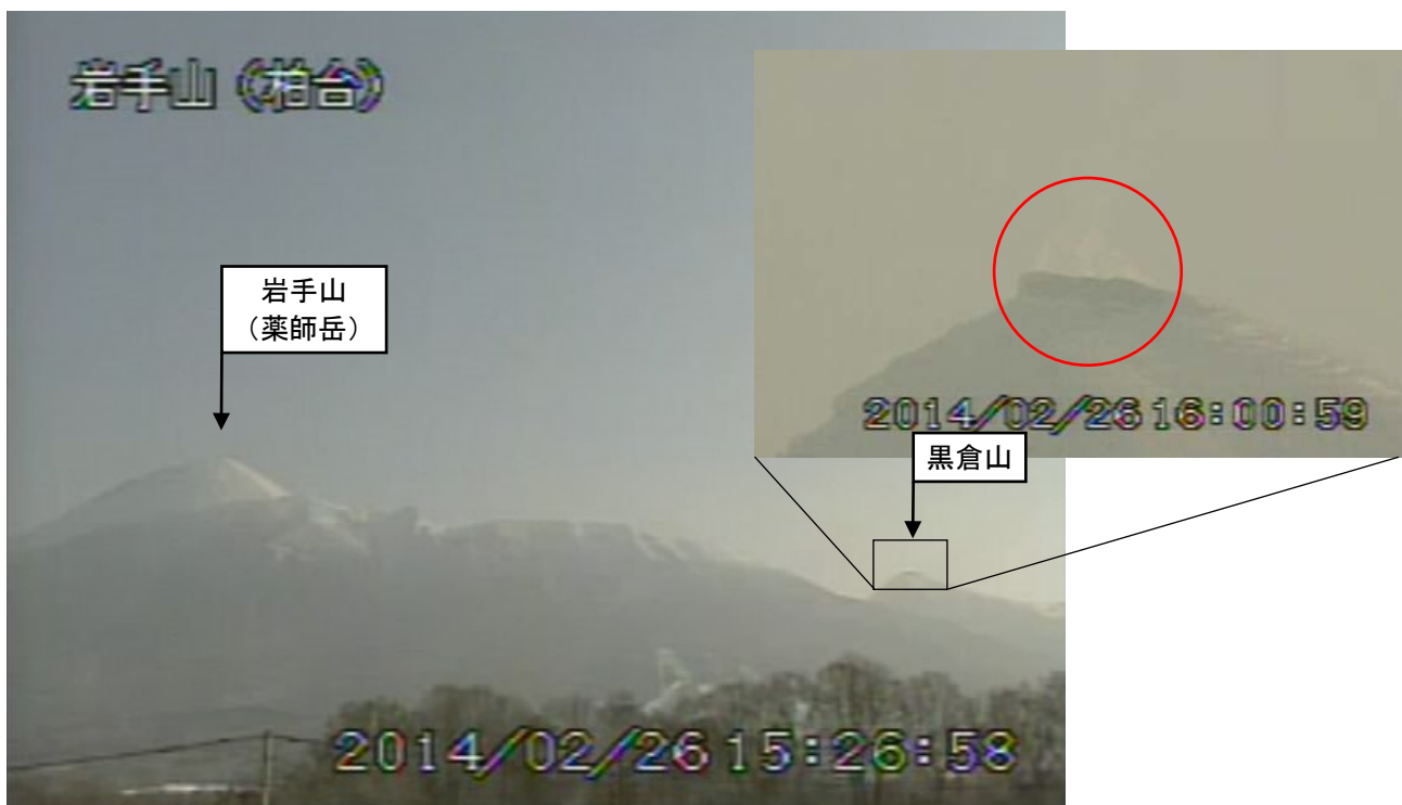
図 1 岩手山 黒倉山の噴気の状況（2 月 26 日 15 時 27 分頃）
