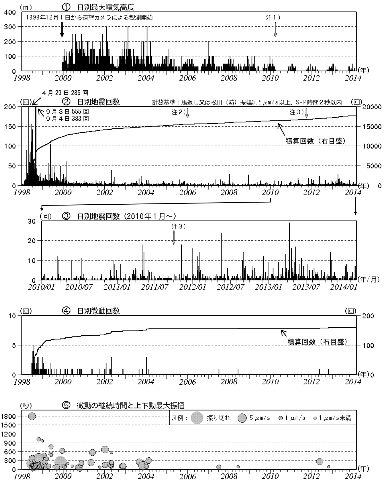
図2 岩手山 火山活動経過図（1998年1月～2014年2月）
