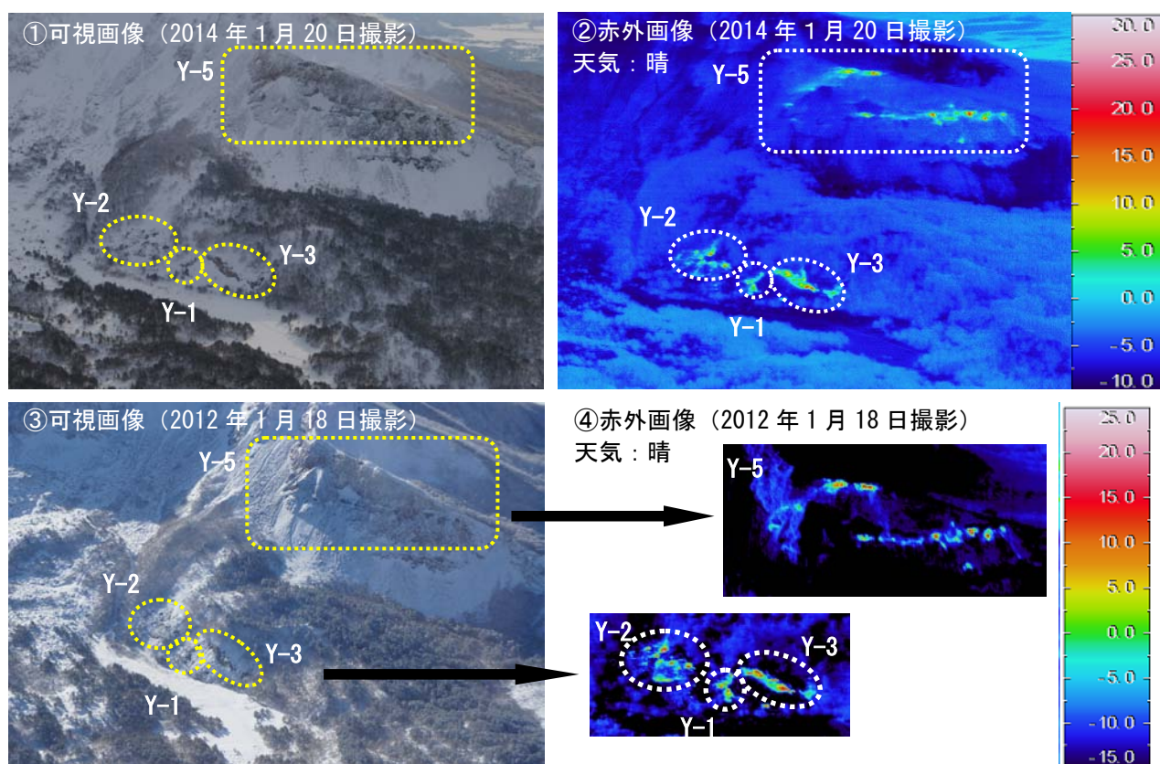
図 4 磐梯山 火口壁噴気地帯（Y-1、2、3、5）の可視画像（左）と地表面温度分布 1) （右）
