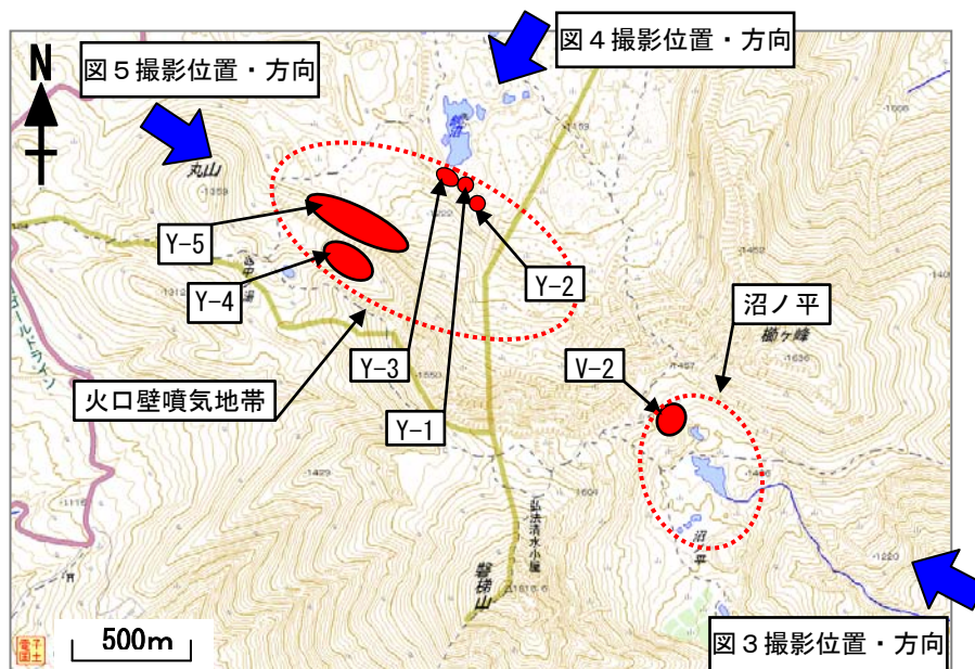
図 2 磐梯山 噴気地熱域の分布図及び可視画像・地表面温度分布 1) の撮影位置と方向
