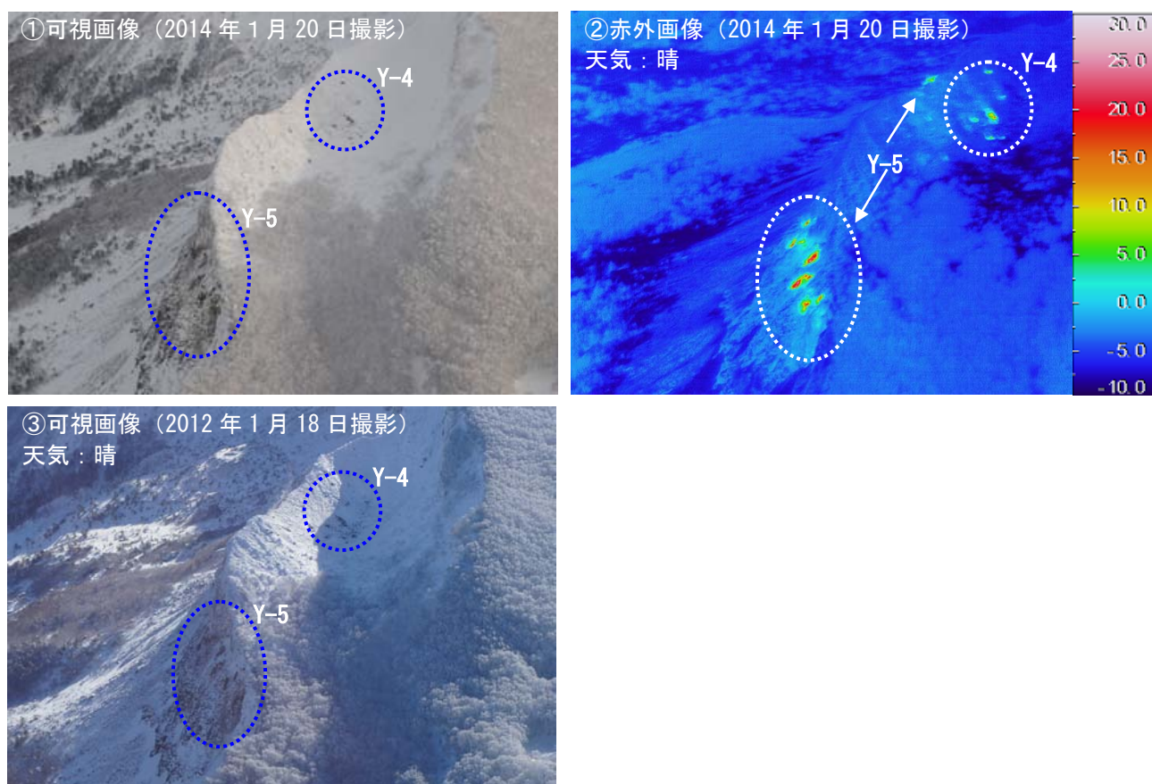
図 5 磐梯山 火口壁噴気地帯（Y-4、5）の可視画像（左）と地表面温度分布 1) （右）
