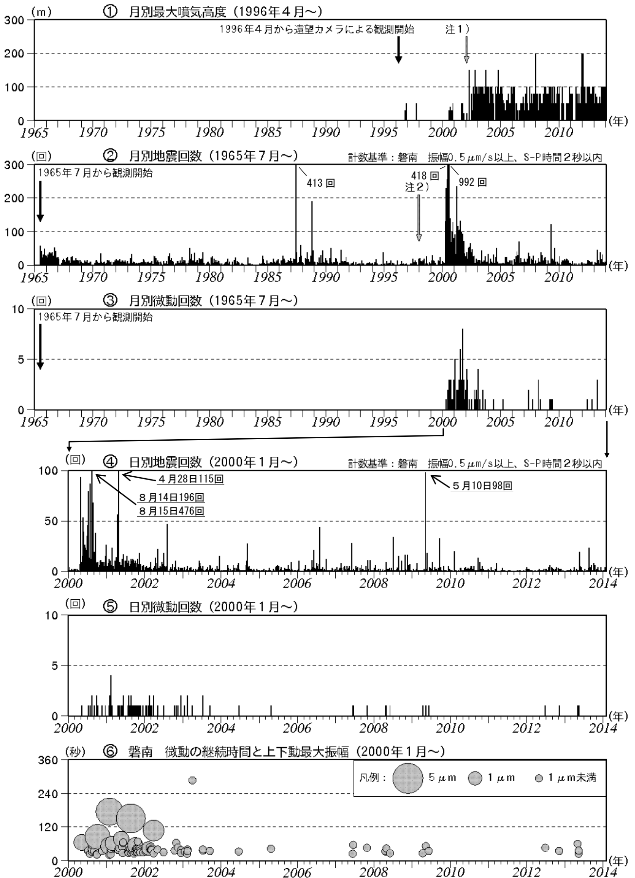
図6 磐梯山 火山活動経過図 (1965年7月～2014年1月)
