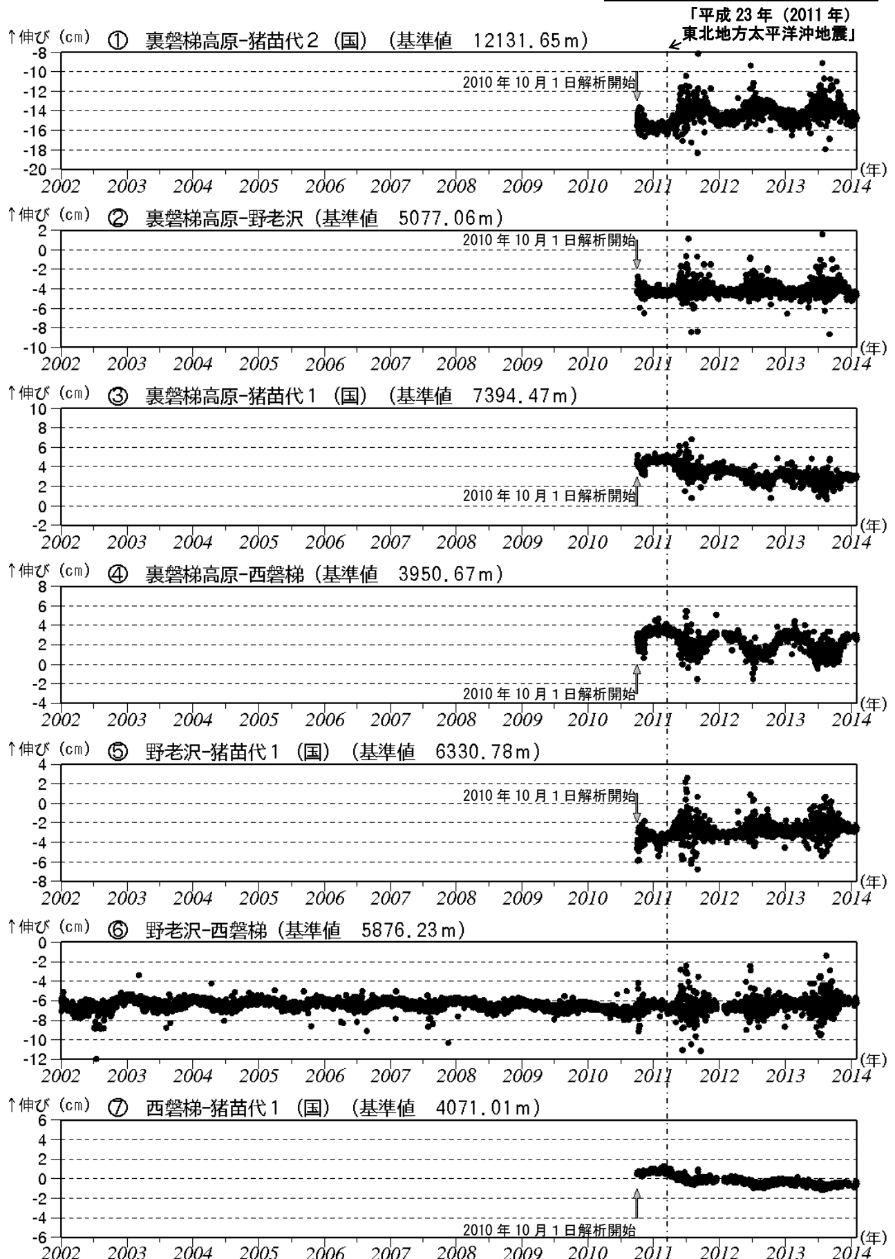
図7 磐梯山 GNSS 基線長変化図 (2002 年 1 月～2014 年 1 月)
