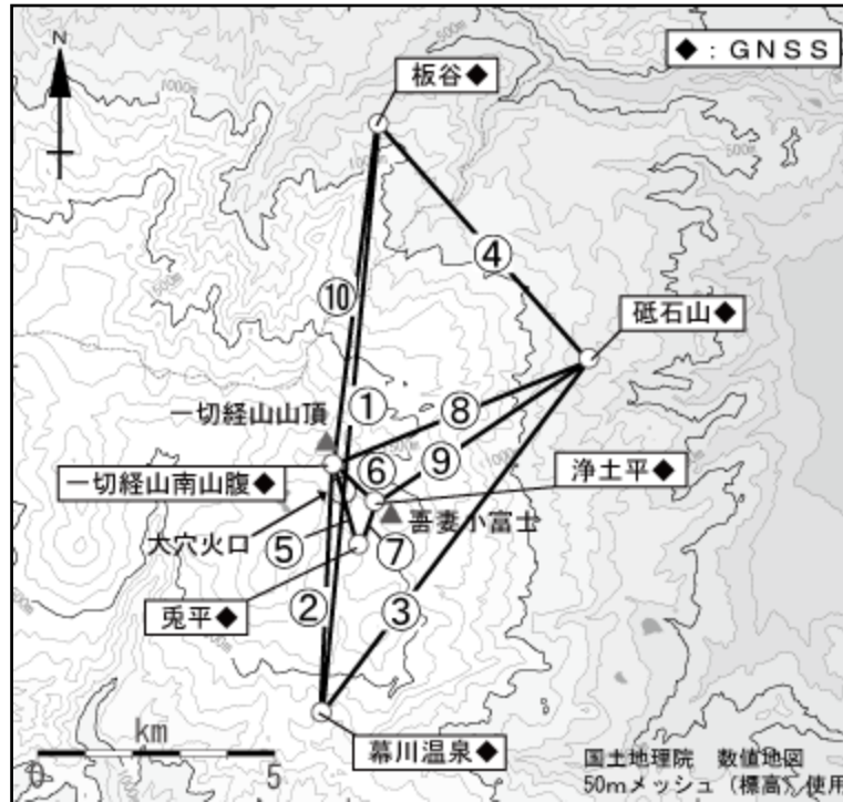
図5 吾妻山 GNSS 観測点配置図
