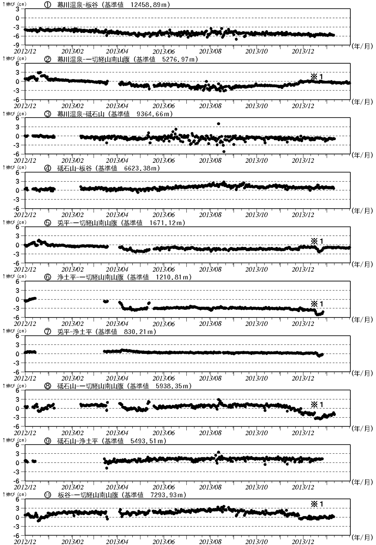
図7 吾妻山 GNSS 基線長変化図 (2012 年 12 月～2014 年 1 月)
