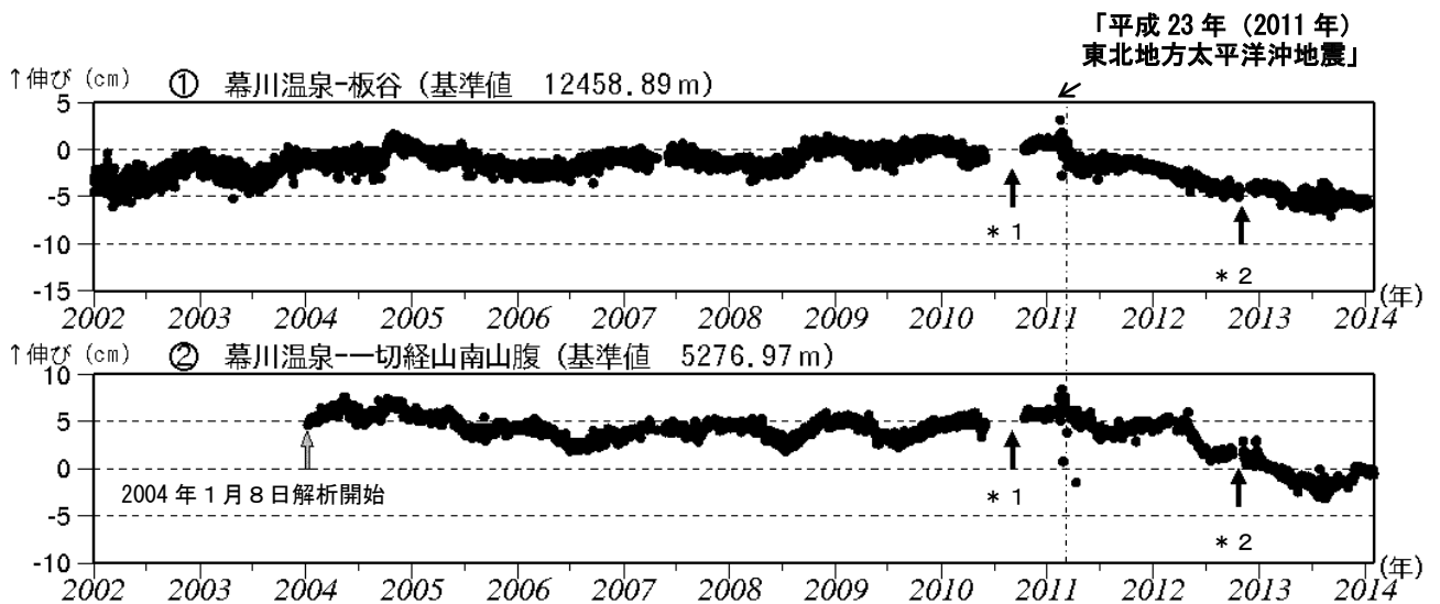
図6 吾妻山 GNSS 基線長変化図 (2002 年 1 月～2014 年 1 月)
