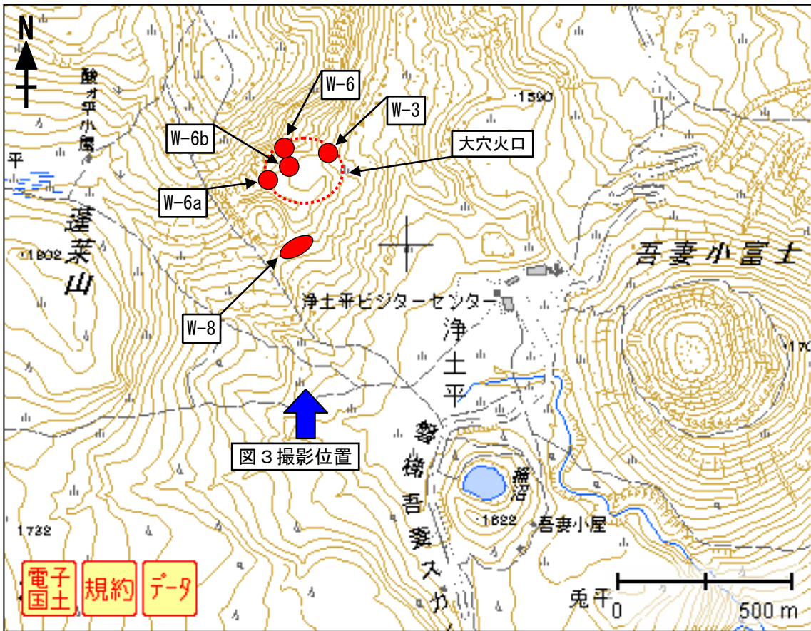
図2 吾妻山 噴気地熱域の分布図及び可視画像と地表面温度分布 1) 撮影位置
