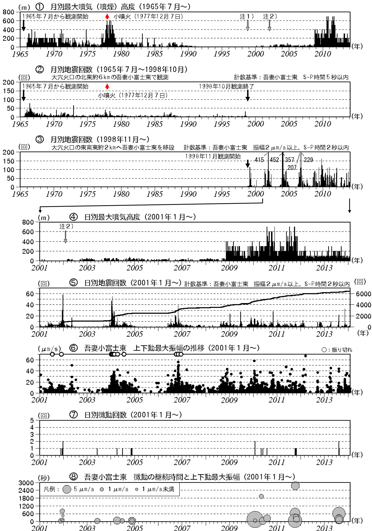
図4 吾妻山 火山活動経過図(1965年7月~2014年1月)
