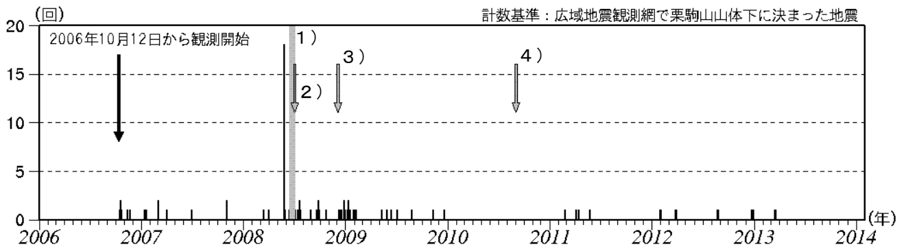
図3 栗駒山 日別地震回数（2006年10月～2014年1月）
