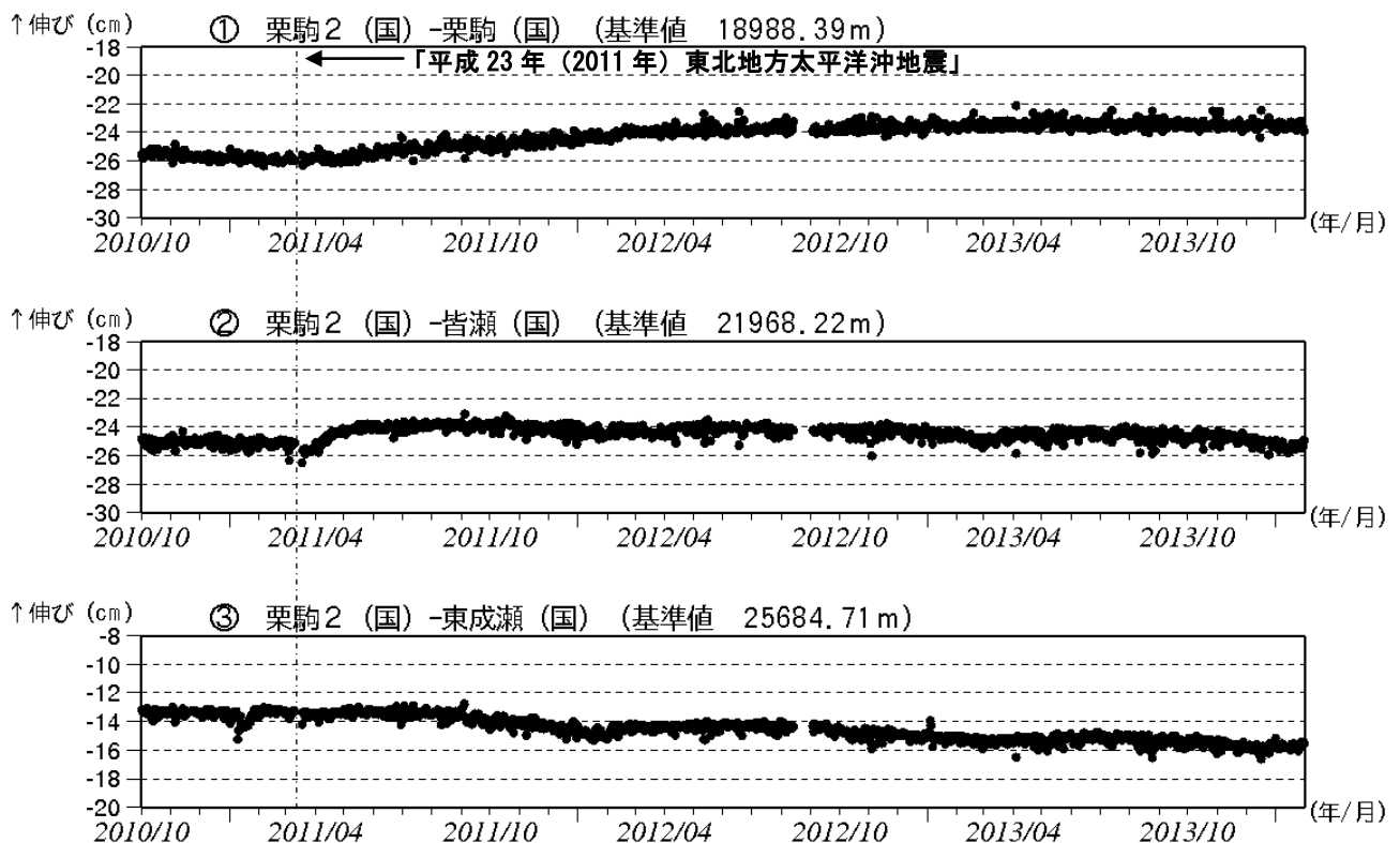
図6 栗駒山 GNSS 基線長変化図（2010 年 10 月～2014 年 1 月）
