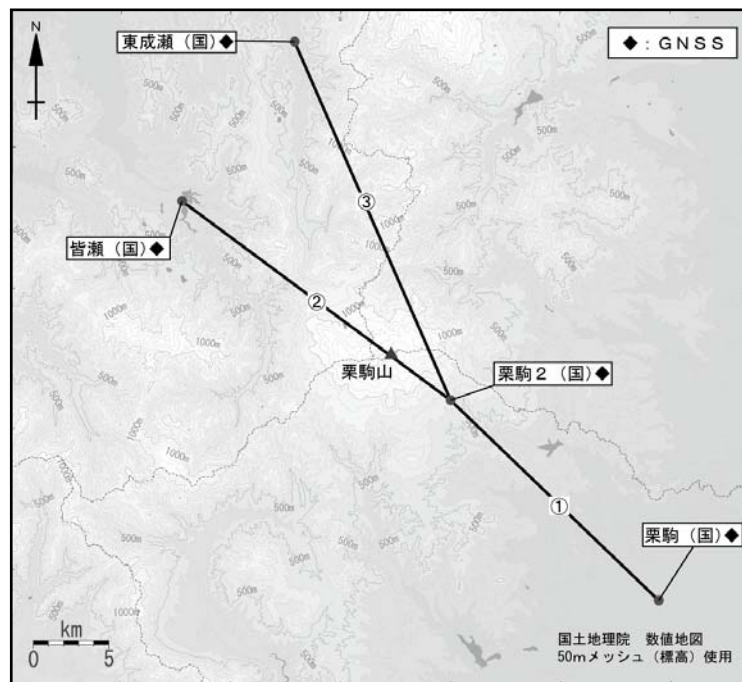
図5 栗駒山 GNSS 観測点配置図
