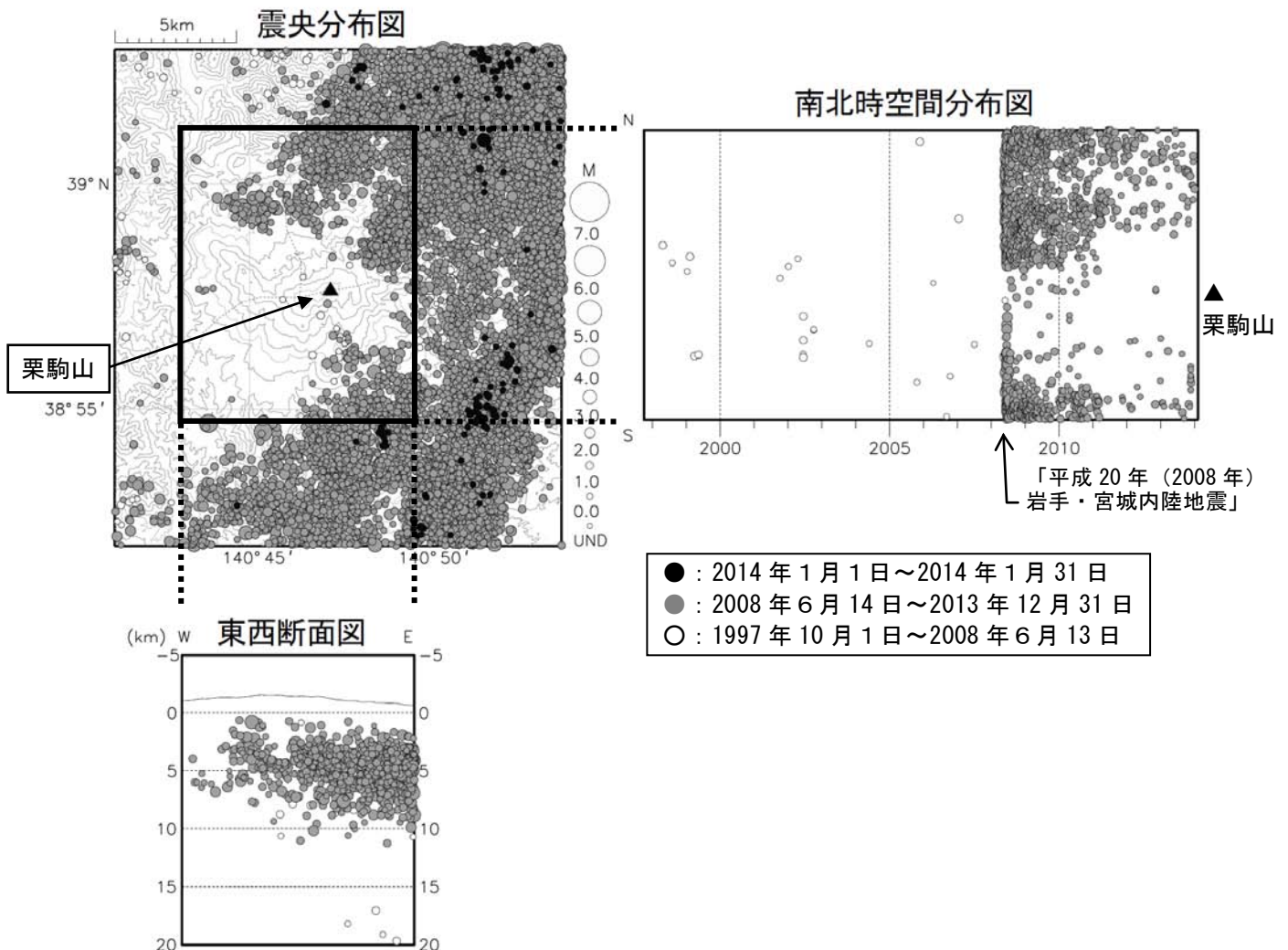
図4 栗駒山 広域地震観測網による栗駒山周辺の地震活動（1997年10月～2014年1月）
