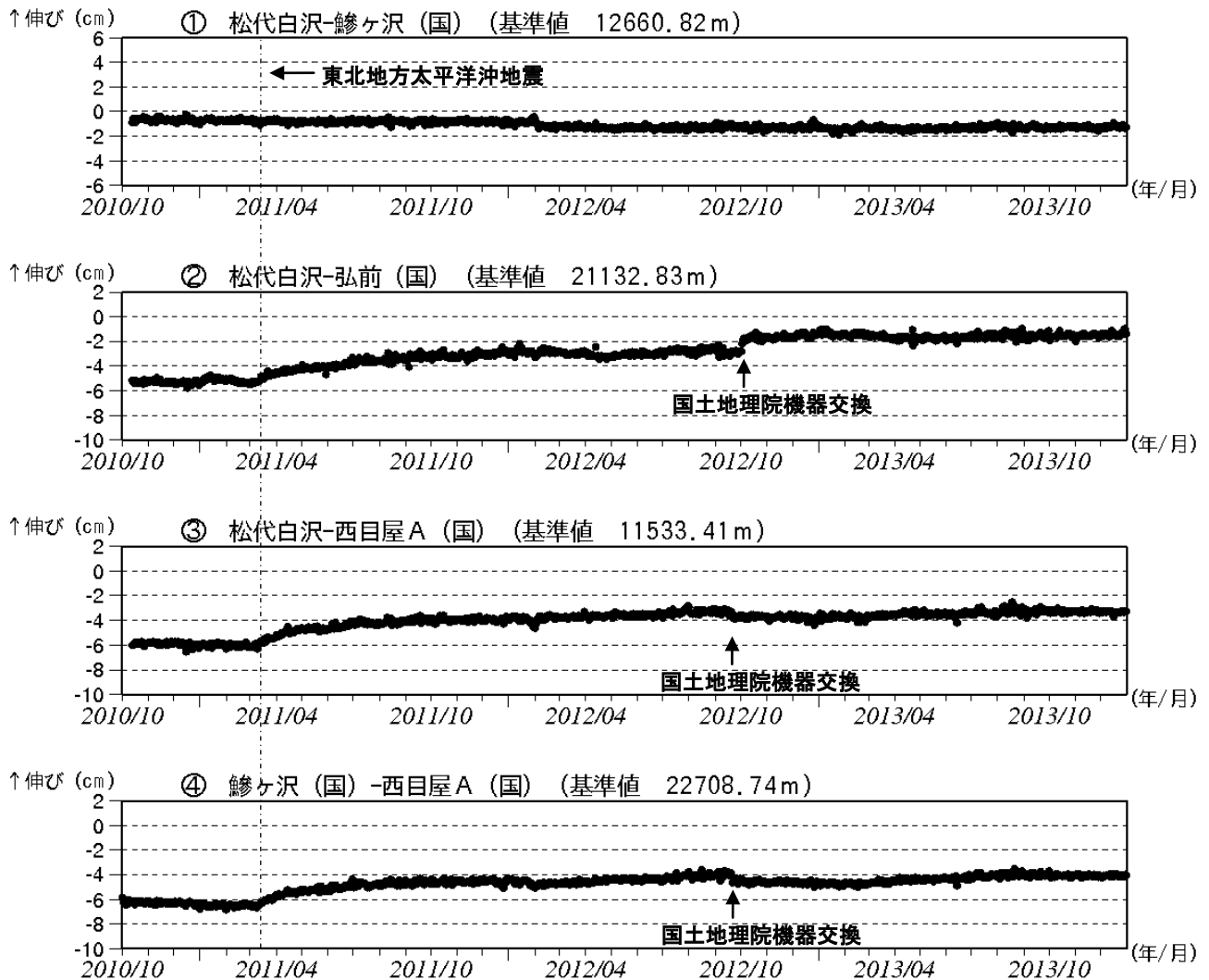
図3 岩木山 GPS 基線長変化図（2010年10月～2013年12月）
