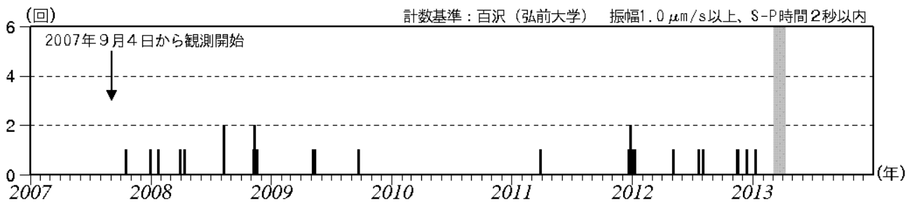
図2 岩木山 日別地震回数（2007年9月～2013年12月）
