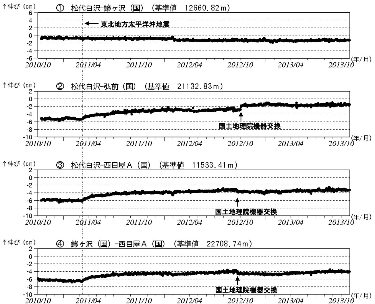
図3 岩木山 GPS 基線長変化図（2010年10月～2013年10月）
