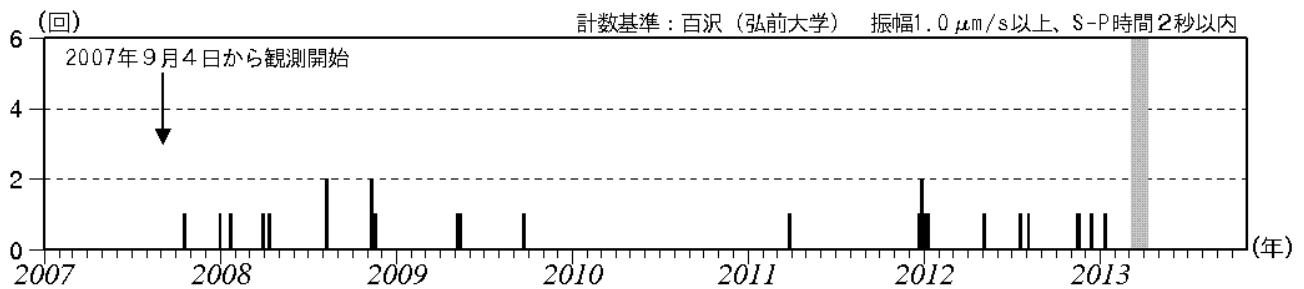
図2 岩木山 日別地震回数（2007年9月～2013年10月）
