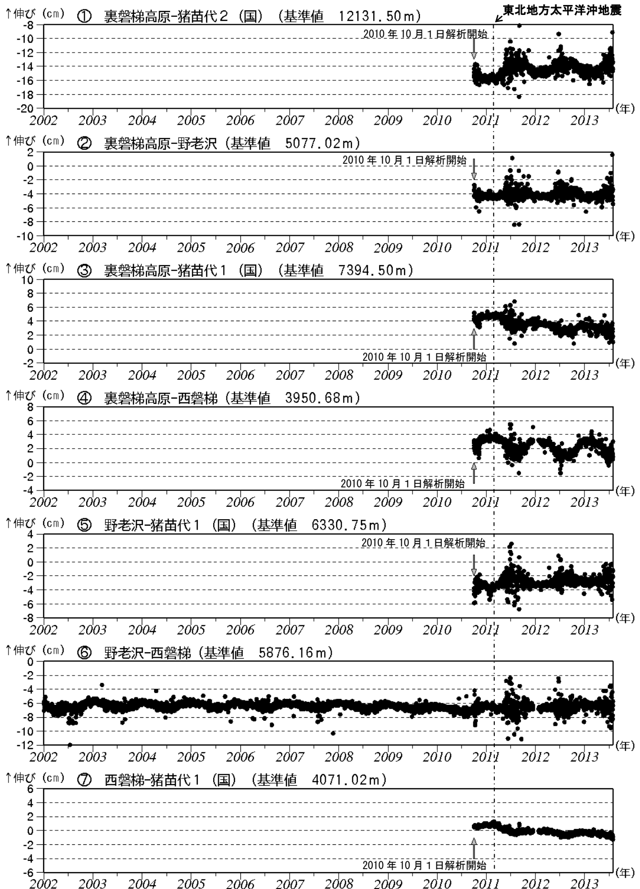
図3 磐梯山 GPS 基線長変化図 (2002年1月～2013年7月)
