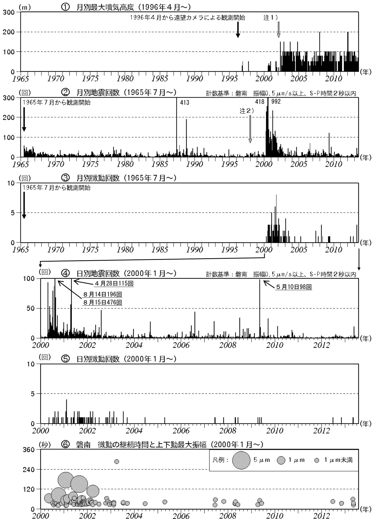
図2 磐梯山 火山活動経過図（1965年7月～2013年7月）
