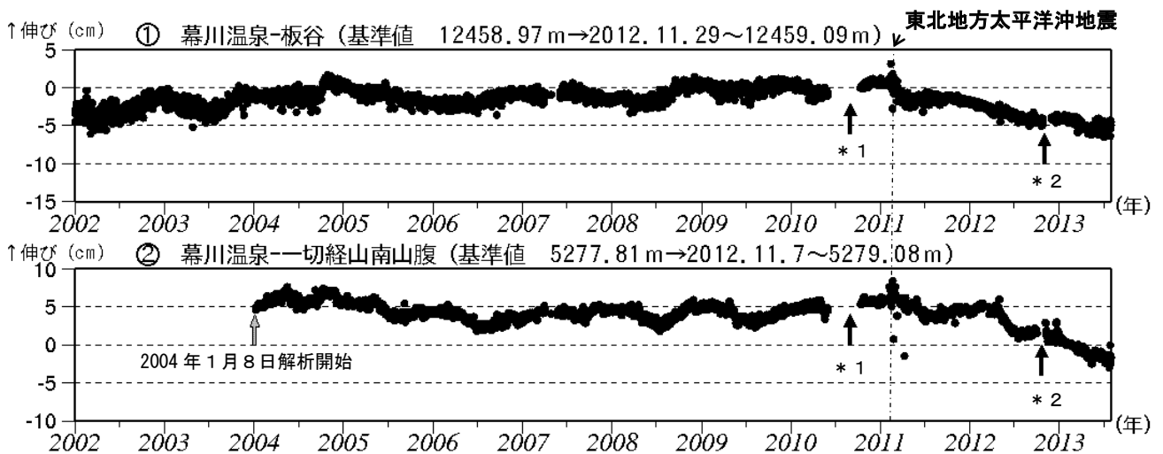
図4 吾妻山 GPS 基線長変化図 (2002年1月~2013年7月)
