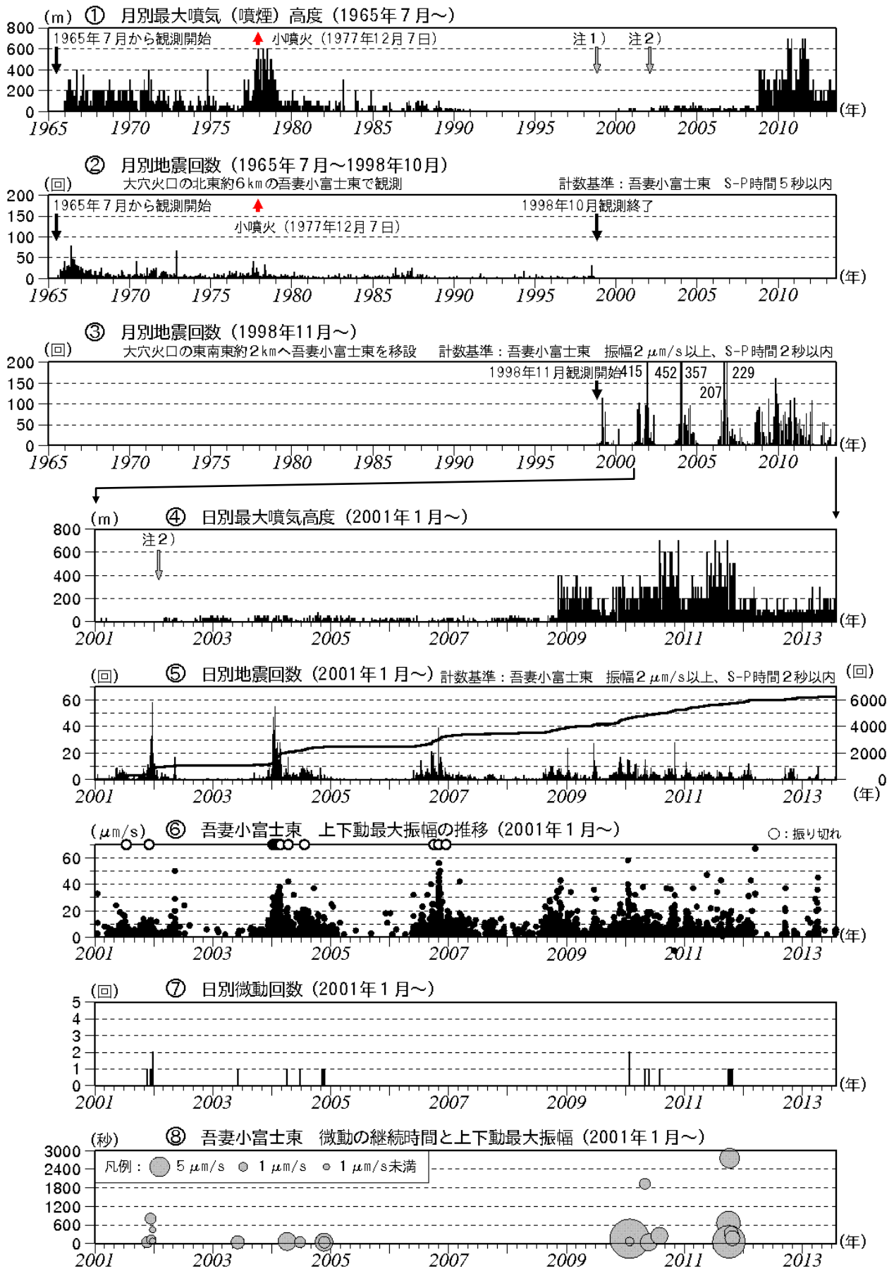
図2 吾妻山 火山活動経過図(1965年7月~2013年7月)
