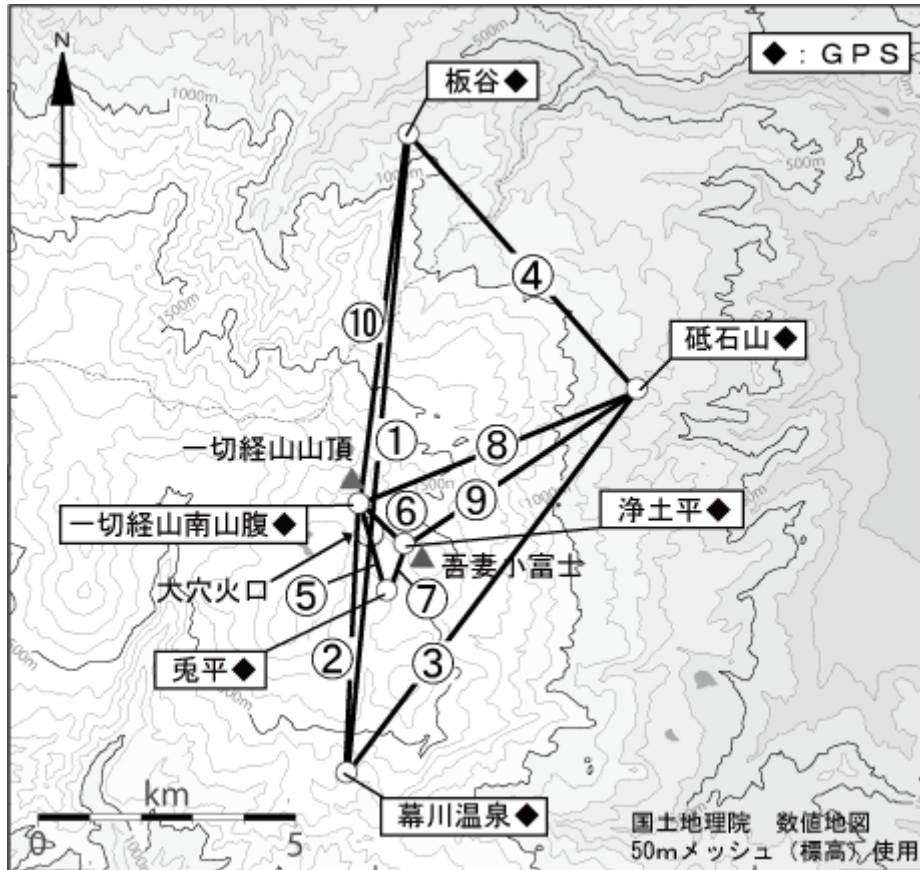
図3 吾妻山 GPS 観測点配置図
