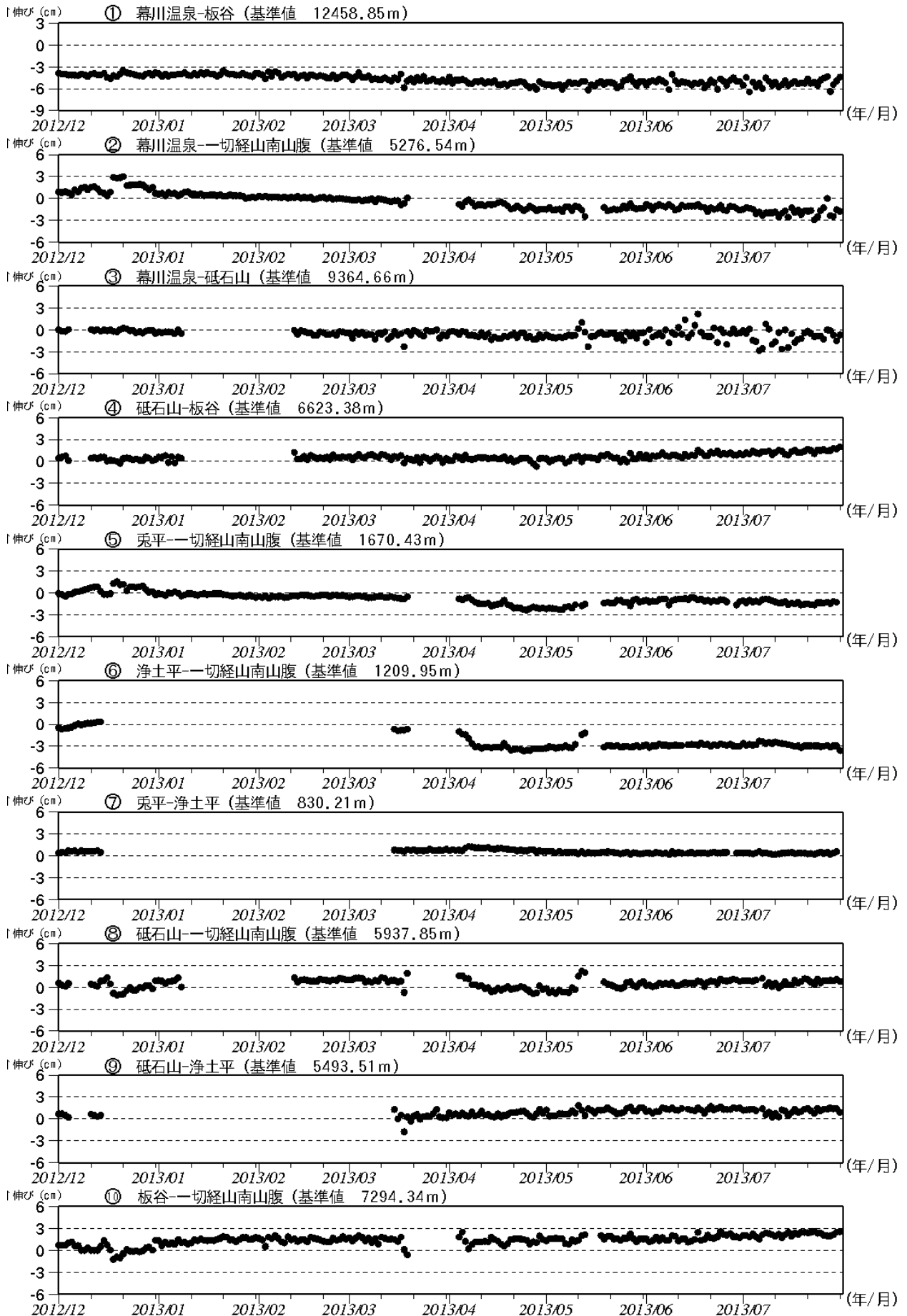
図5 吾妻山 GPS 基線長変化図 (2012 年 12 月~2013 年 7 月)
