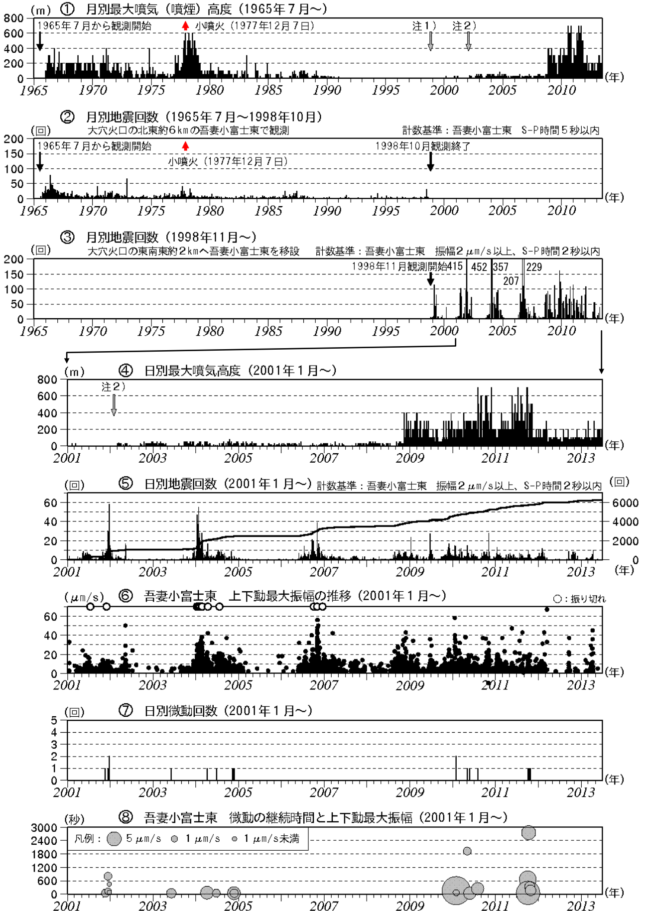
図2 吾妻山 火山活動経過図(1965年7月～2013年6月)
