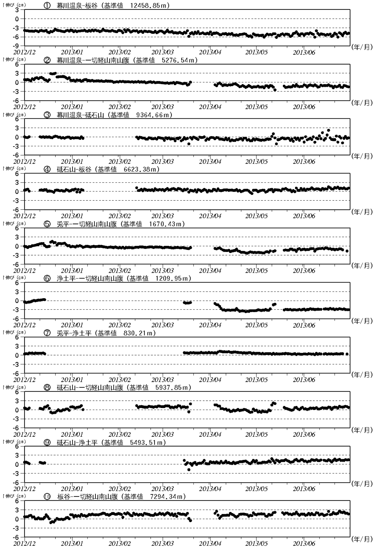
図5 吾妻山 GPS 基線長変化図 (2012 年 12 月～2013 年 6 月)
