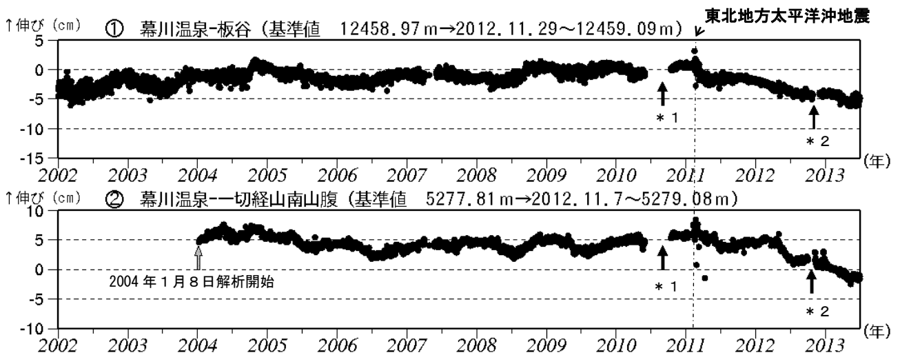
図4 吾妻山 GPS 基線長変化図 (2002年1月～2013年6月)
