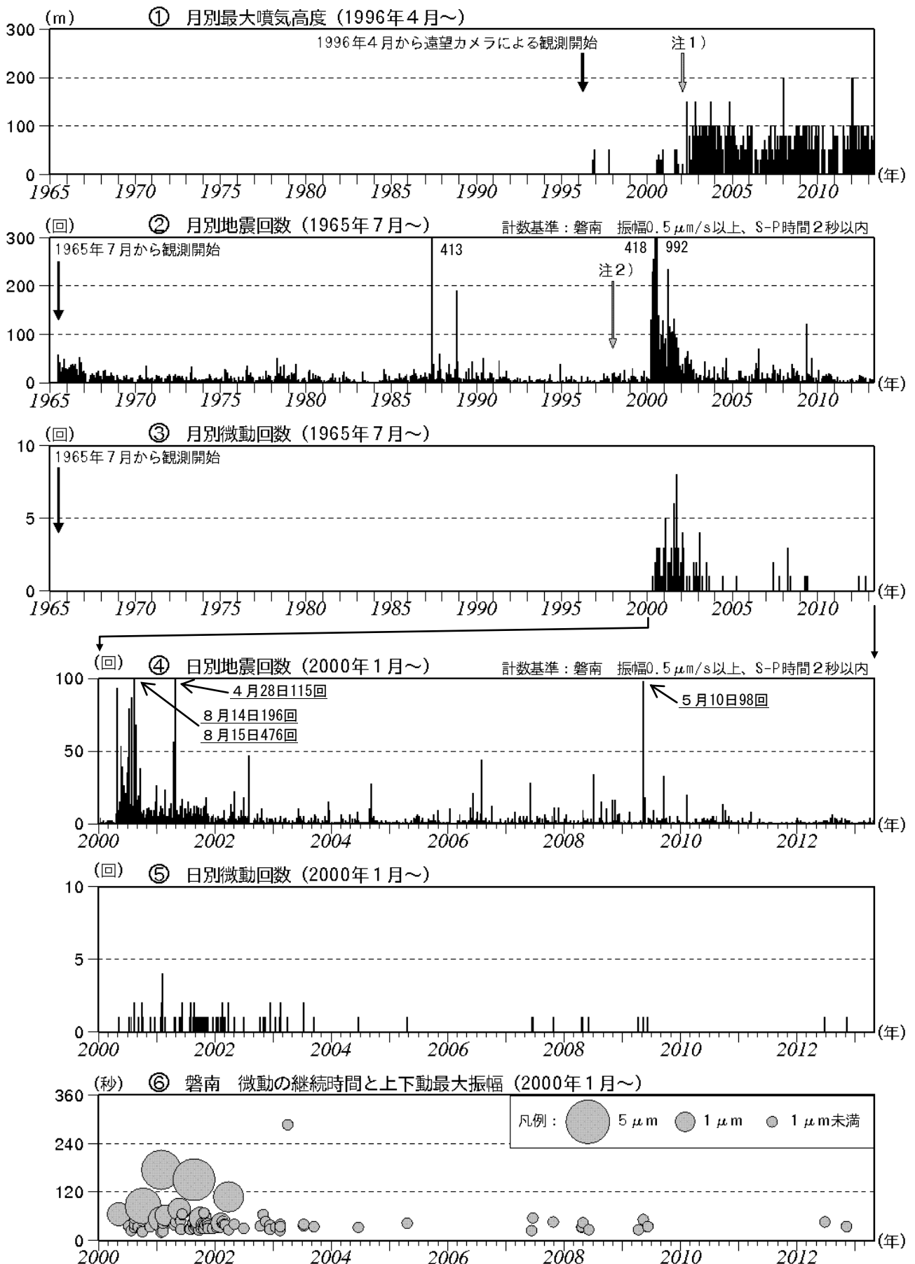
図2※ 磐梯山 火山活動経過図（1965年7月～2013年4月）
