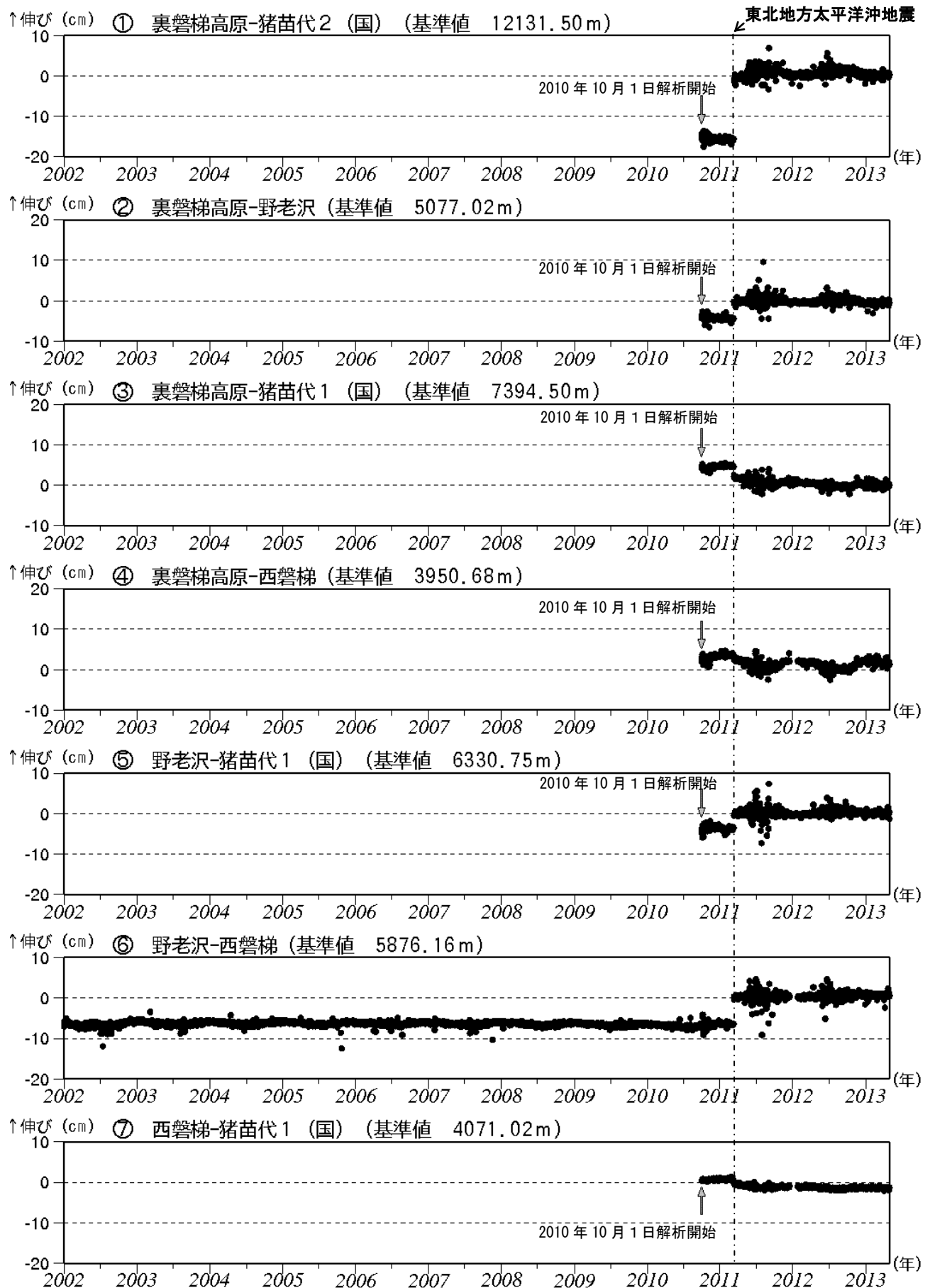
図 3※ 磐梯山 GPS 基線長変化図 (2002 年 1 月～2013 年 4 月)
