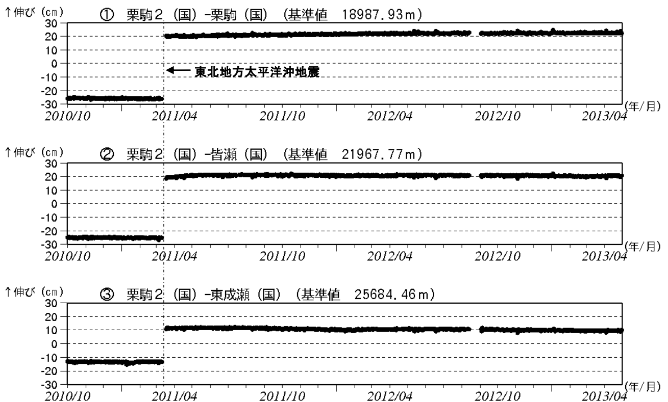
図 5※ 栗駒山 GPS 基線長変化図 (2010 年 10 月～2013 年 4 月)
