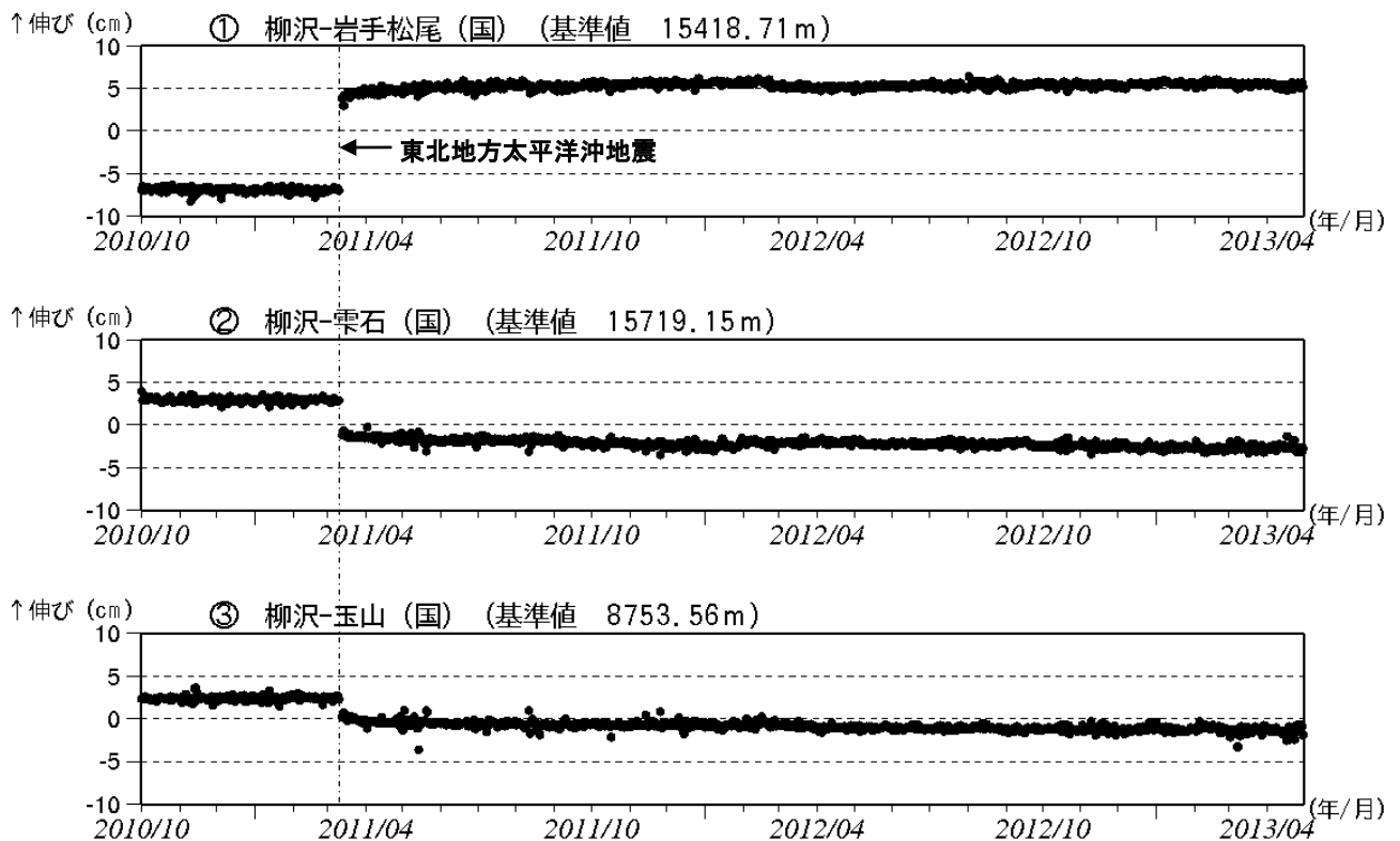
図4※ 岩手山 GPS 基線長変化図（2010 年 10 月～2013 年 4 月）
