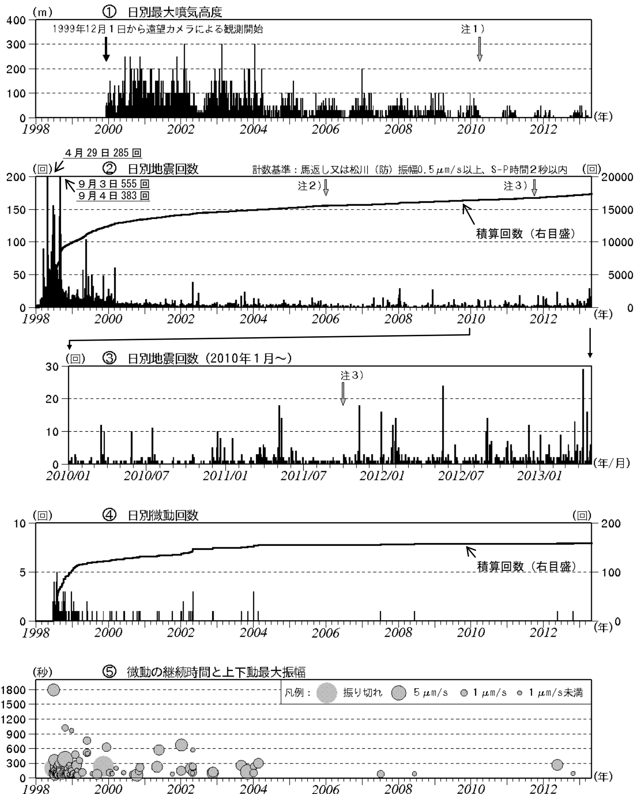
図2※ 岩手山 火山活動経過図（1998年1月～2013年4月）
