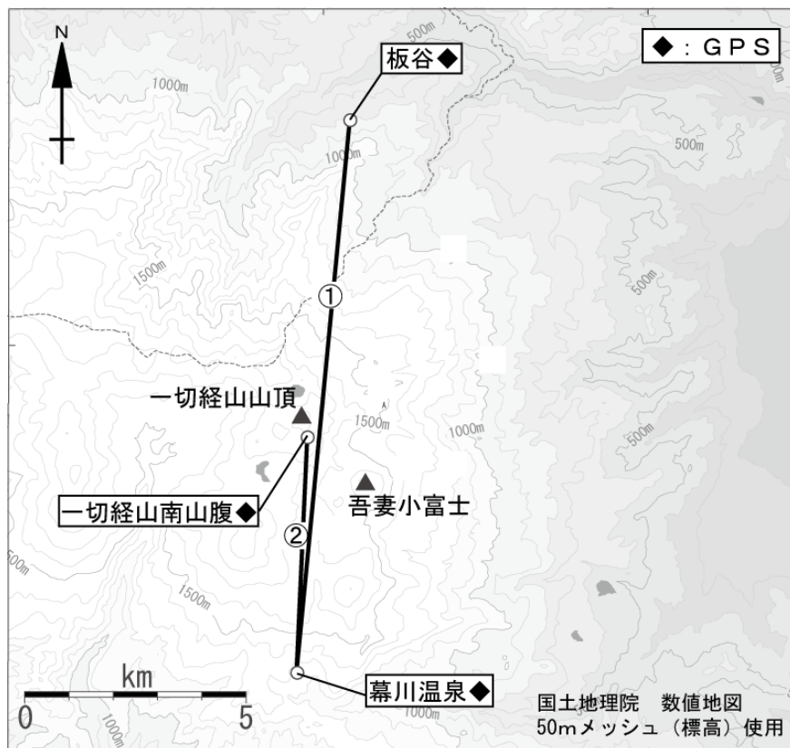
図7 吾妻山 GPS 観測点配置図
