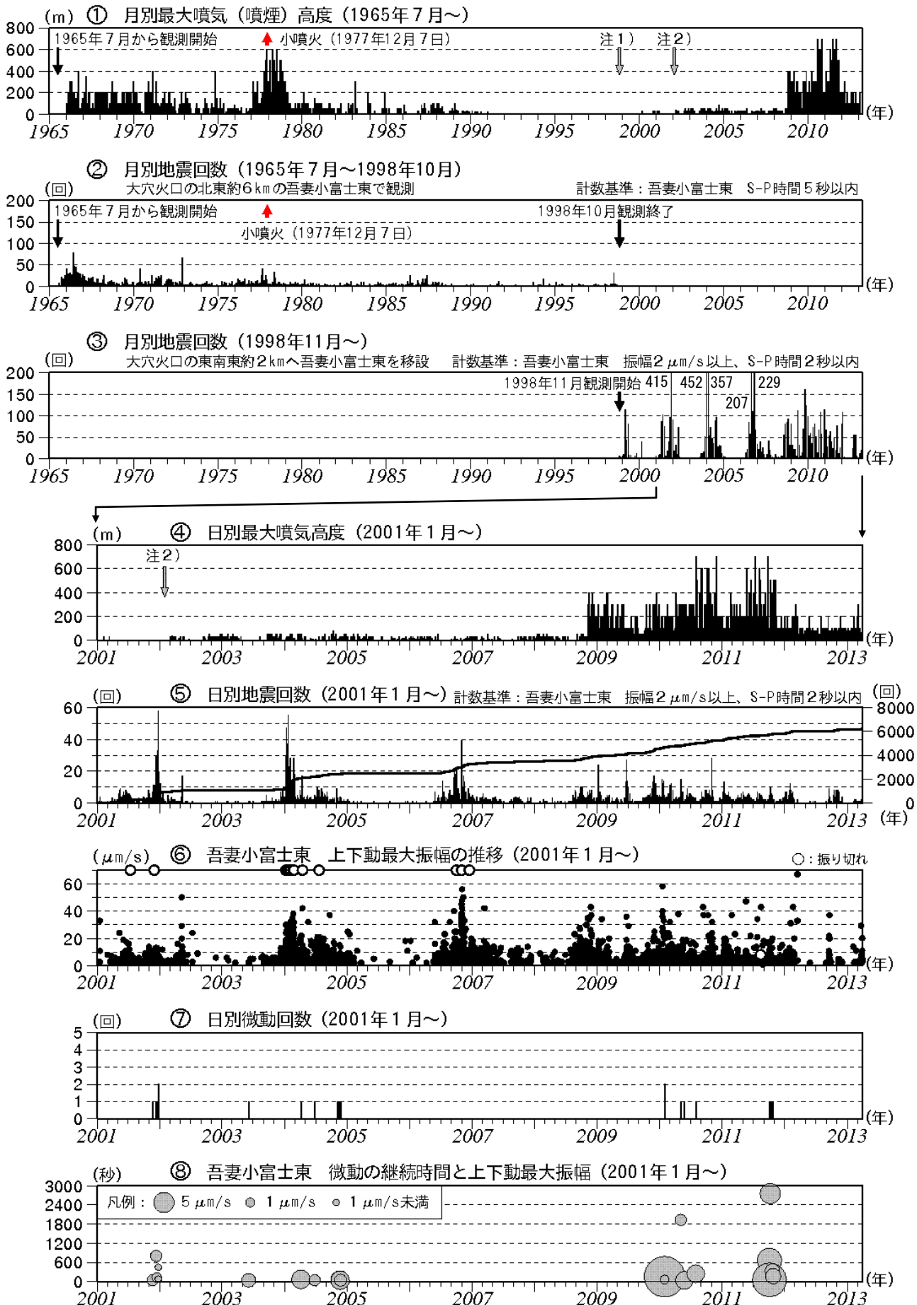
図5 吾妻山 火山活動経過図（1965年7月～2013年3月）
