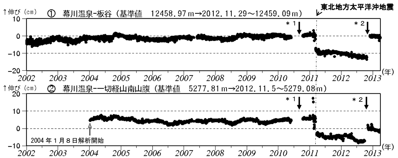
図6 吾妻山 GPS 基線長変化図 (2002 年 1 月～2013 年 3 月)
