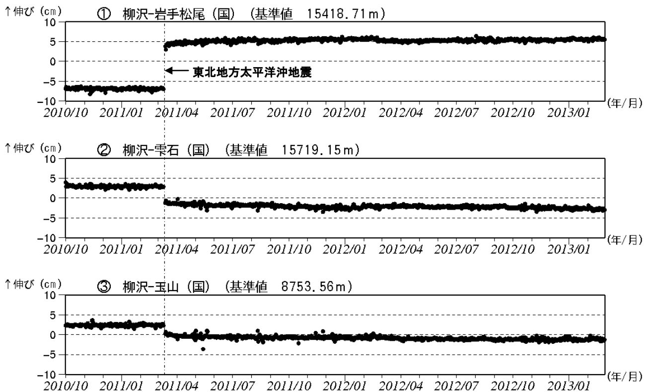
図4※ 岩手山 GPS 基線長変化図（2010 年 10 月～2013 年 2 月）
