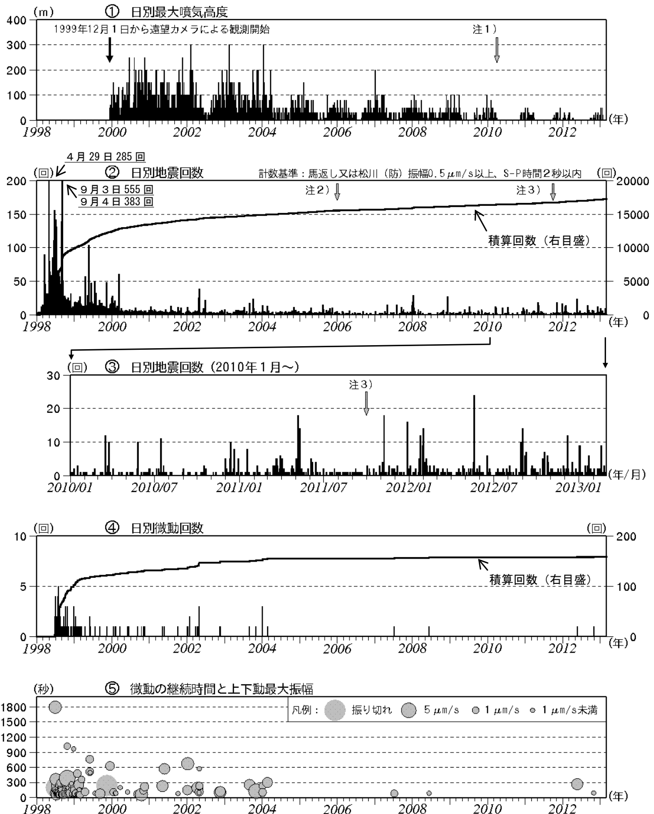
図2※ 岩手山 火山活動経過図（1998年1月～2013年2月）
