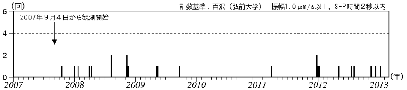
図 2※ 岩木山 日別地震回数（2007 年 9 月～2013 年 2 月）
