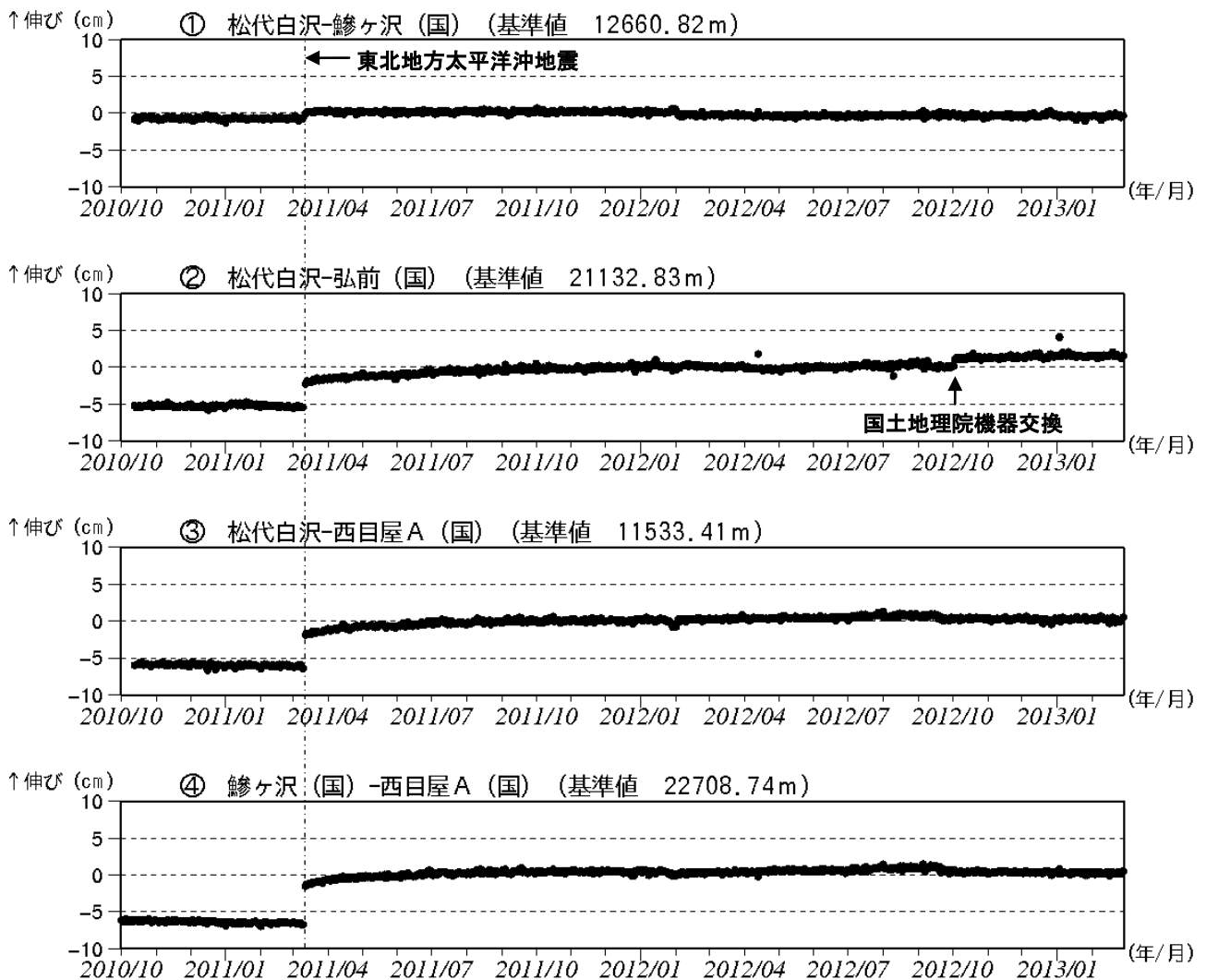
図 3※ 岩木山 GPS 基線長変化図（2010 年 10 月～2013 年 2 月）
