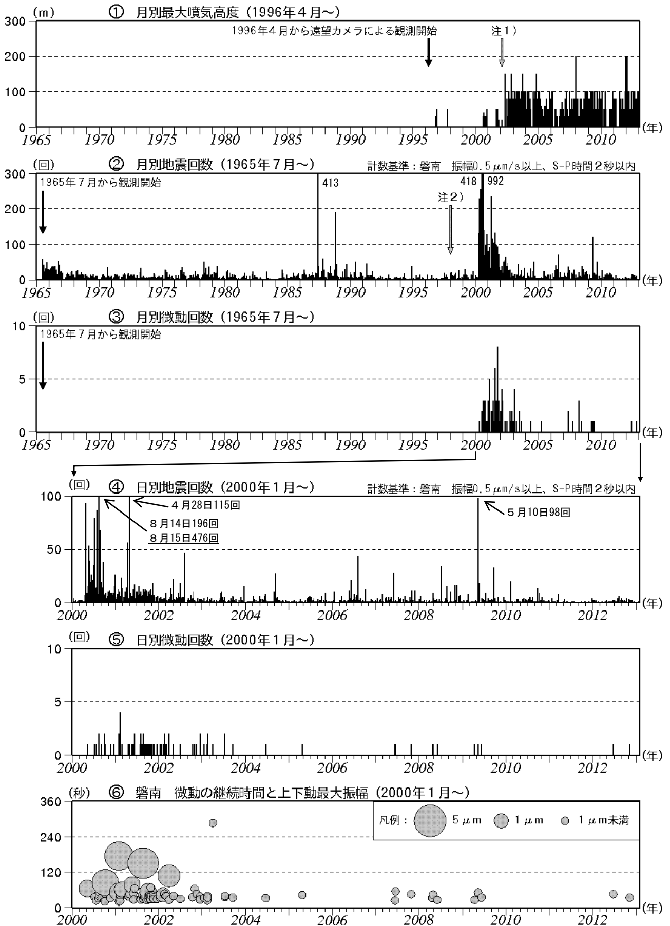
図2※ 磐梯山 火山活動経過図（1965年7月～2013年1月）
