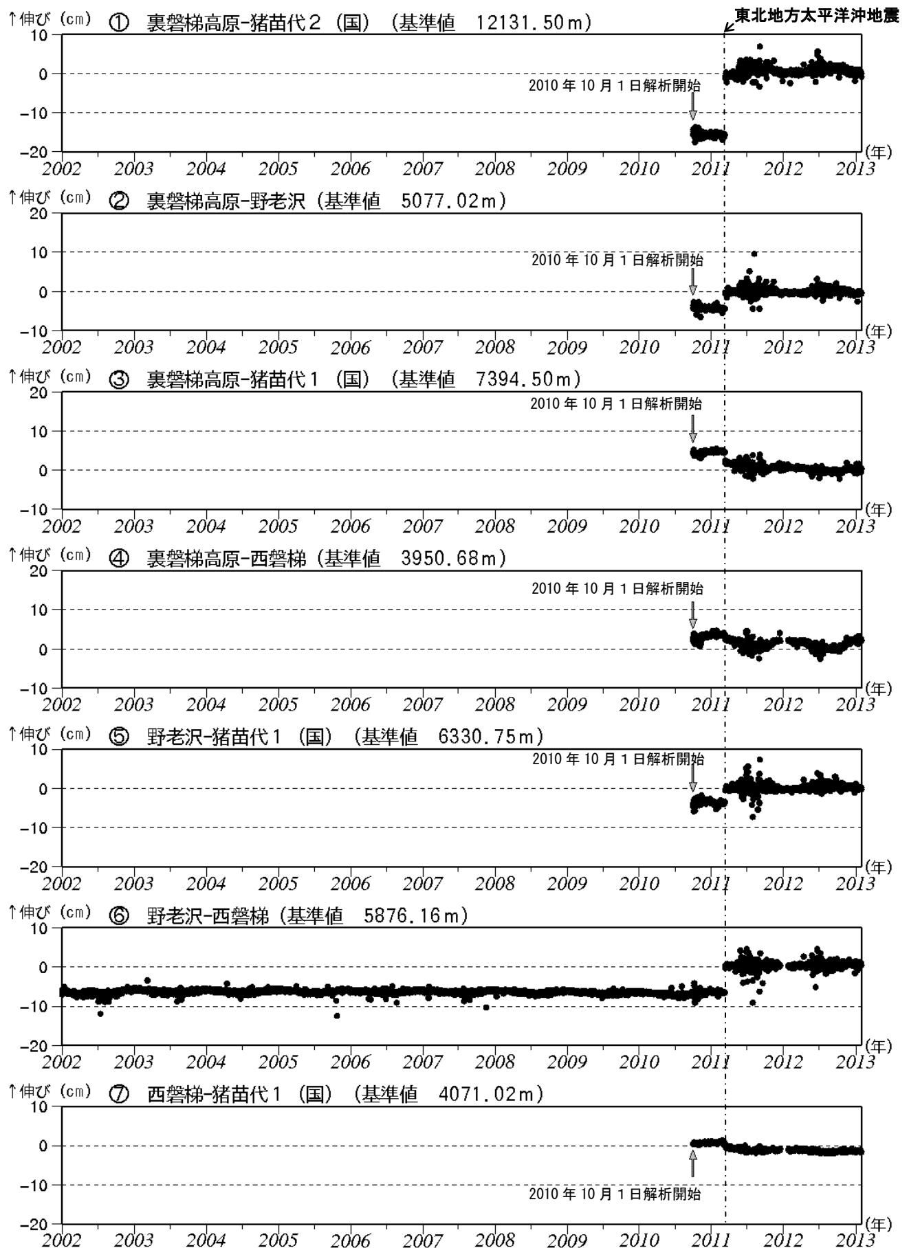
図 3※ 磐梯山 GPS 基線長変化図 (2002 年 1 月～2013 年 1 月)
