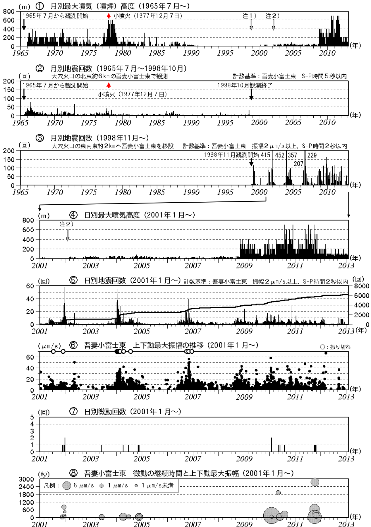
図2 吾妻山 火山活動経過図（1965年7月～2013年1月）
