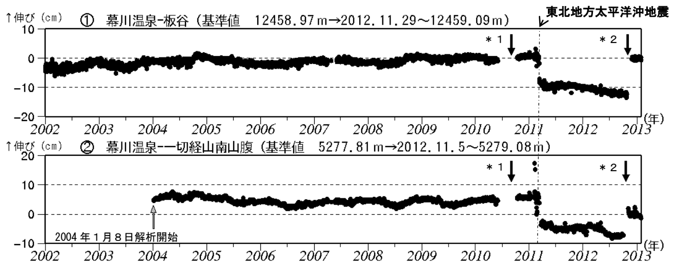
図3 吾妻山 GPS 基線長変化図 (2002 年 1 月～2013 年 1 月)
