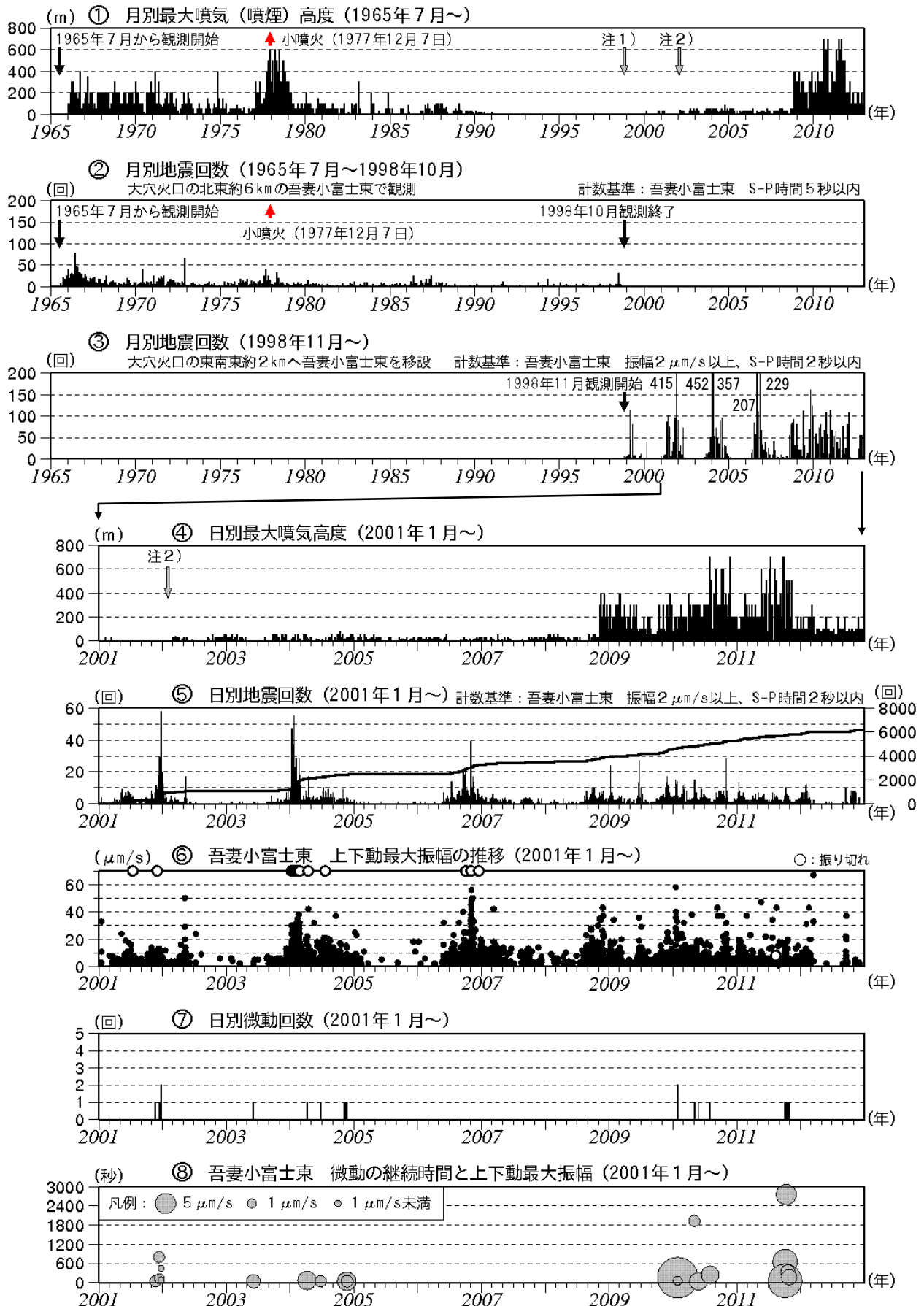
図2 吾妻山 火山活動経過図（1965年7月～2012年12月）
