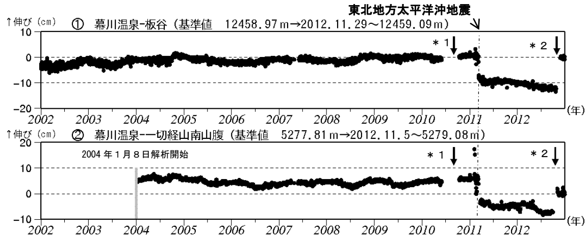
図3 吾妻山 GPS 基線長変化図 (2002 年 1 月～2012 年 12 月)
