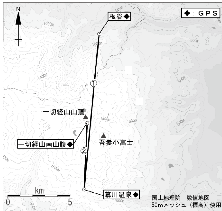
図4 吾妻山 GPS 観測点配置図
