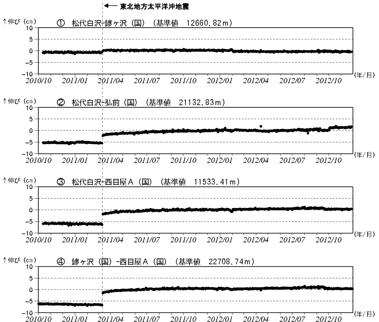
図 3※ 岩木山 GPS 基線長変化図（2010 年 10 月～2012 年 11 月）
