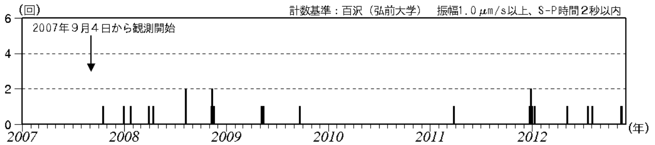
図 2※ 岩木山 日別地震回数（2007 年 9 月～2012 年 11 月）
