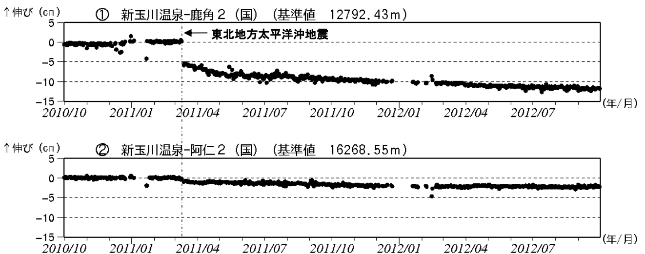
図 3※ 秋田焼山 GPS 基線長変化図（2010 年 10 月～2012 年 9 月）
