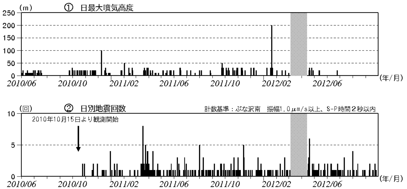
図 2 秋田焼山 火山活動経過図（2010 年 6 月～2012 年 9 月）
