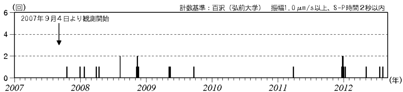
図 3※ 岩木山 日別地震回数（2007 年 9 月～2012 年 8 月）
