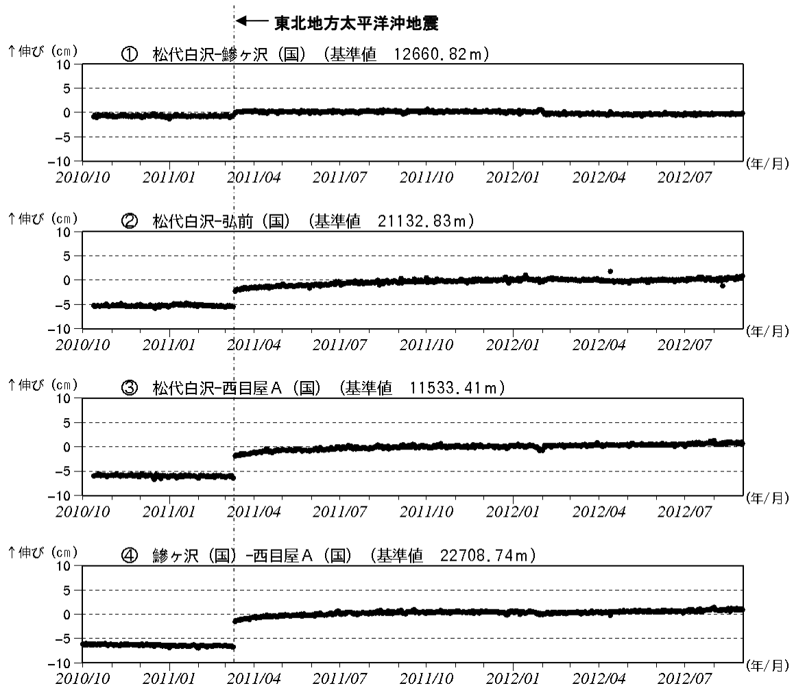
図5 岩木山 GPS 基線長変化図（2010 年 10 月～2012 年 8 月）
