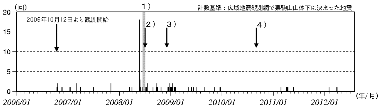
図 3※ 栗駒山 日別地震回数（2006 年 10 月～2012 年 7 月）
