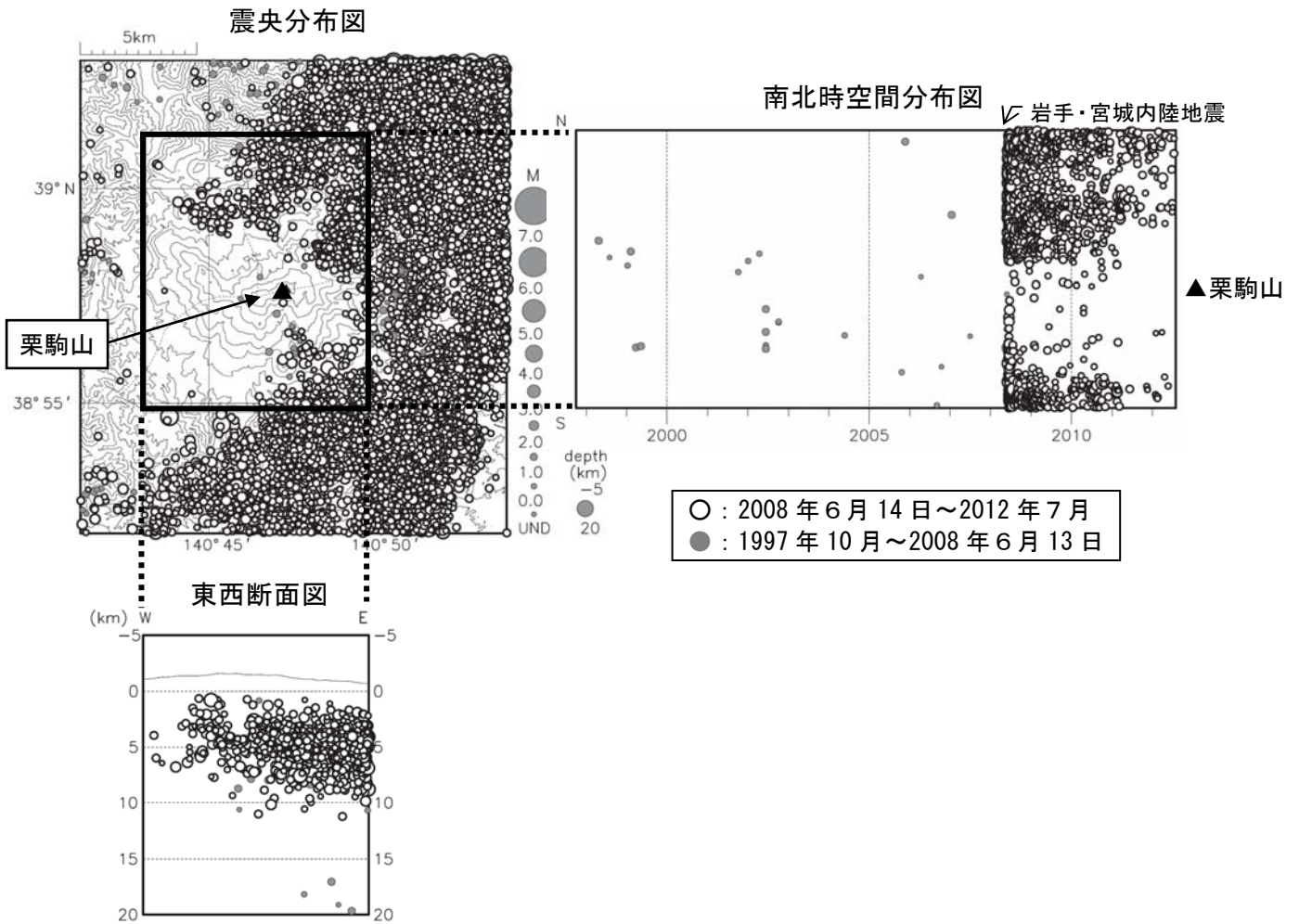
図 4※ 栗駒山 広域地震観測網による栗駒山周辺の地震活動（1997 年 10 月～2012 年 7 月）
