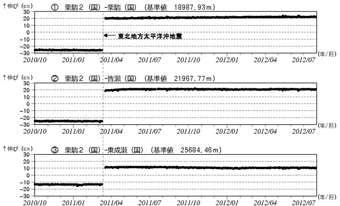
図6 栗駒山 GPS 基線長変化図（2010年10月～2012年7月）
