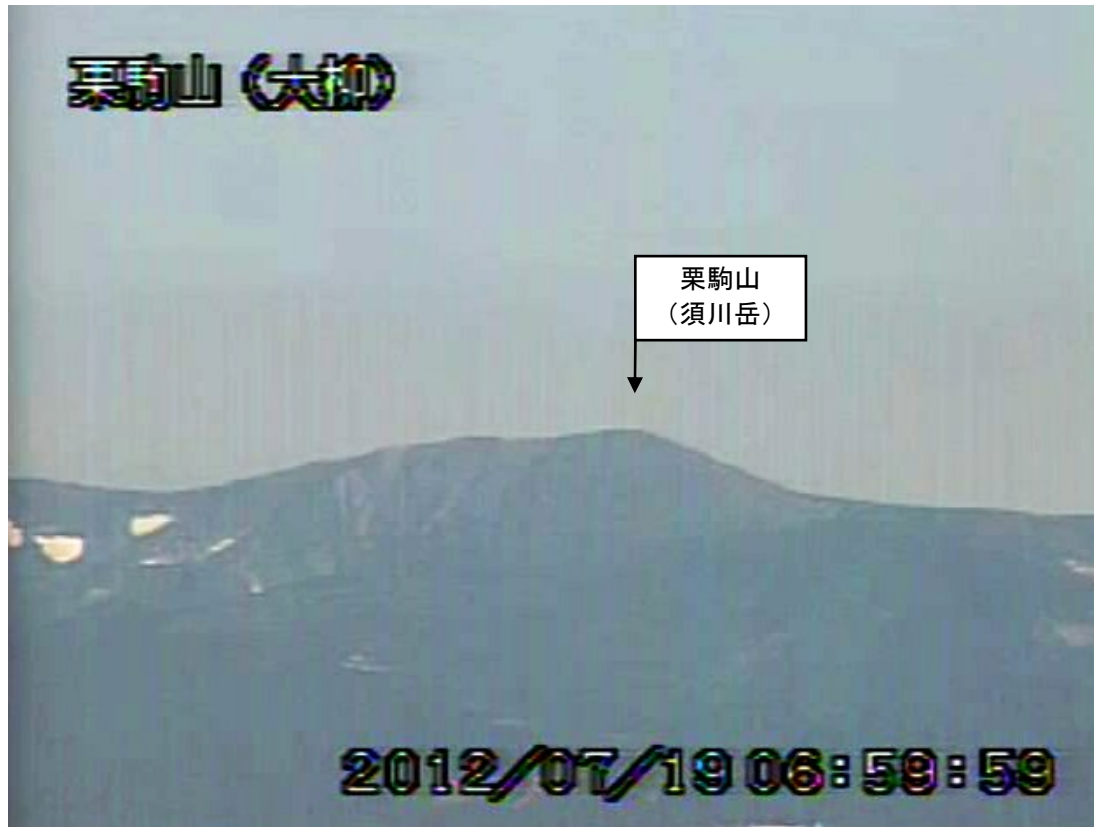
図 2 栗駒山 遠望カメラの映像（7 月 19 日 07 時 00 分頃） ・大柳（山頂の南東約 20km）に設置してある遠望カメラによる。
