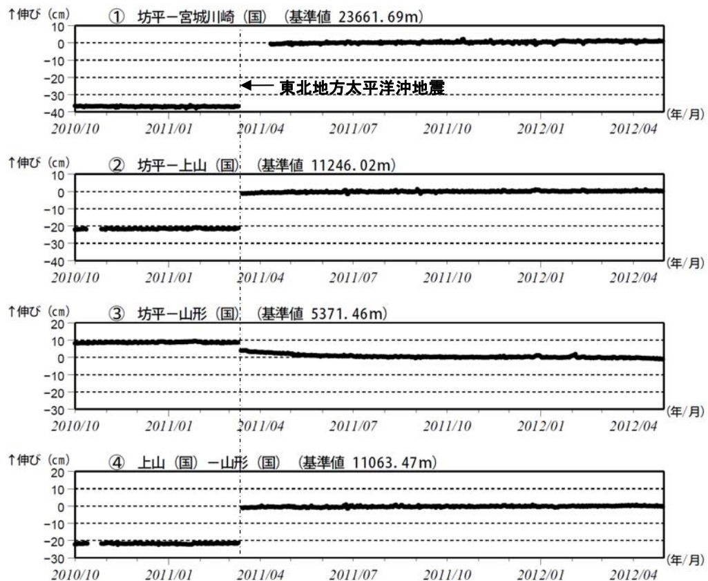
図5 蔵王山 GPS 基線長変化図（2010 年 10 月～2012 年 4 月） 2011 年 3 月 11 日以降の変動は、東北地方太平洋沖地震による影響であり、火山活動によるものではないと考えられます。 ①～④は図4の GPS 基線①～④に対応しています。 グラフの空白部分は欠測を表しています。
