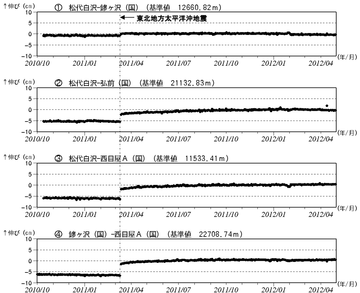
図5 岩木山 GPS 基線長変化図 (2010 年 10 月～2012 年 4 月)
