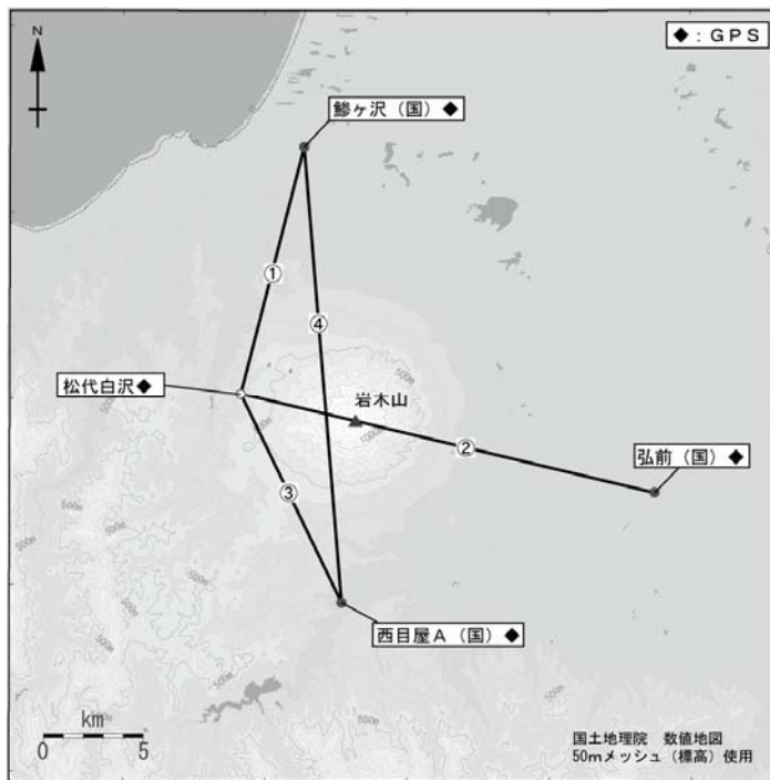
図4 岩木山 GPS 観測点配置図 小さな白丸 (○) は気象庁、小さな黒丸 (●) は気象庁以外の機関の観測点位置を示しています。(国)：国土地理院
