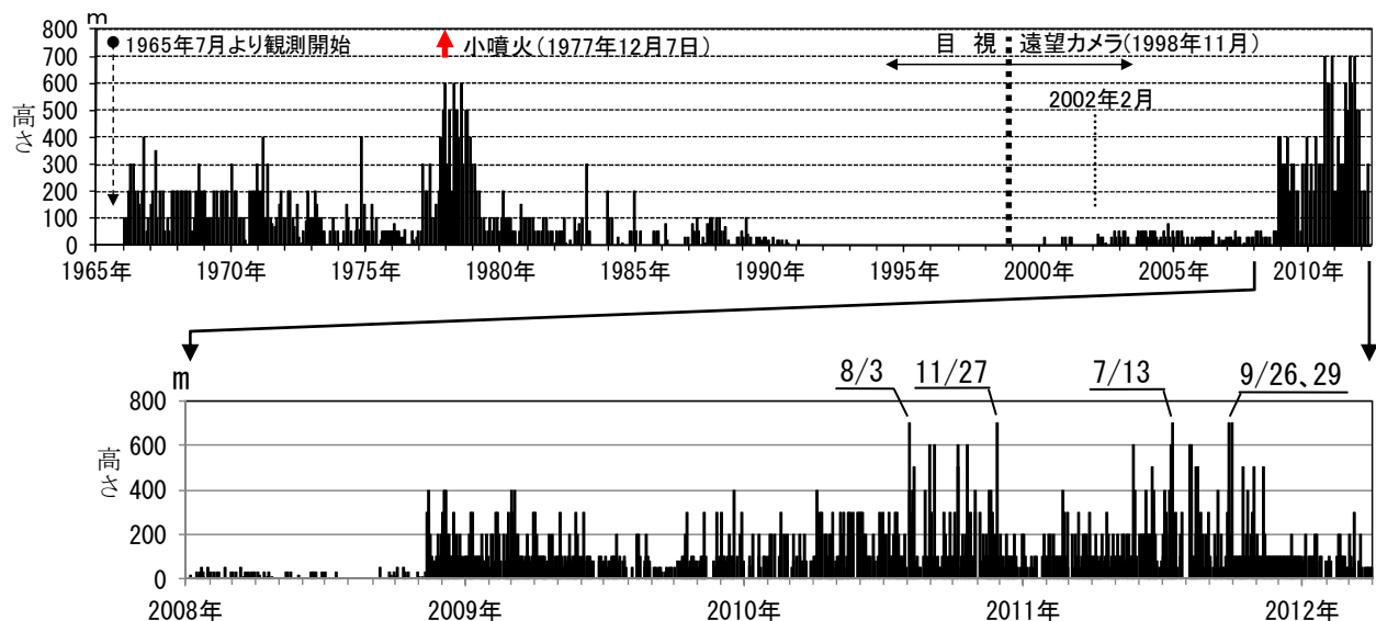
図3 吾妻山の噴気の高さ 上段：月別最大噴気（噴煙）高（1965年7月～2012年3月） 下段：日別最大噴気高（2008年1月～2012年3月）
