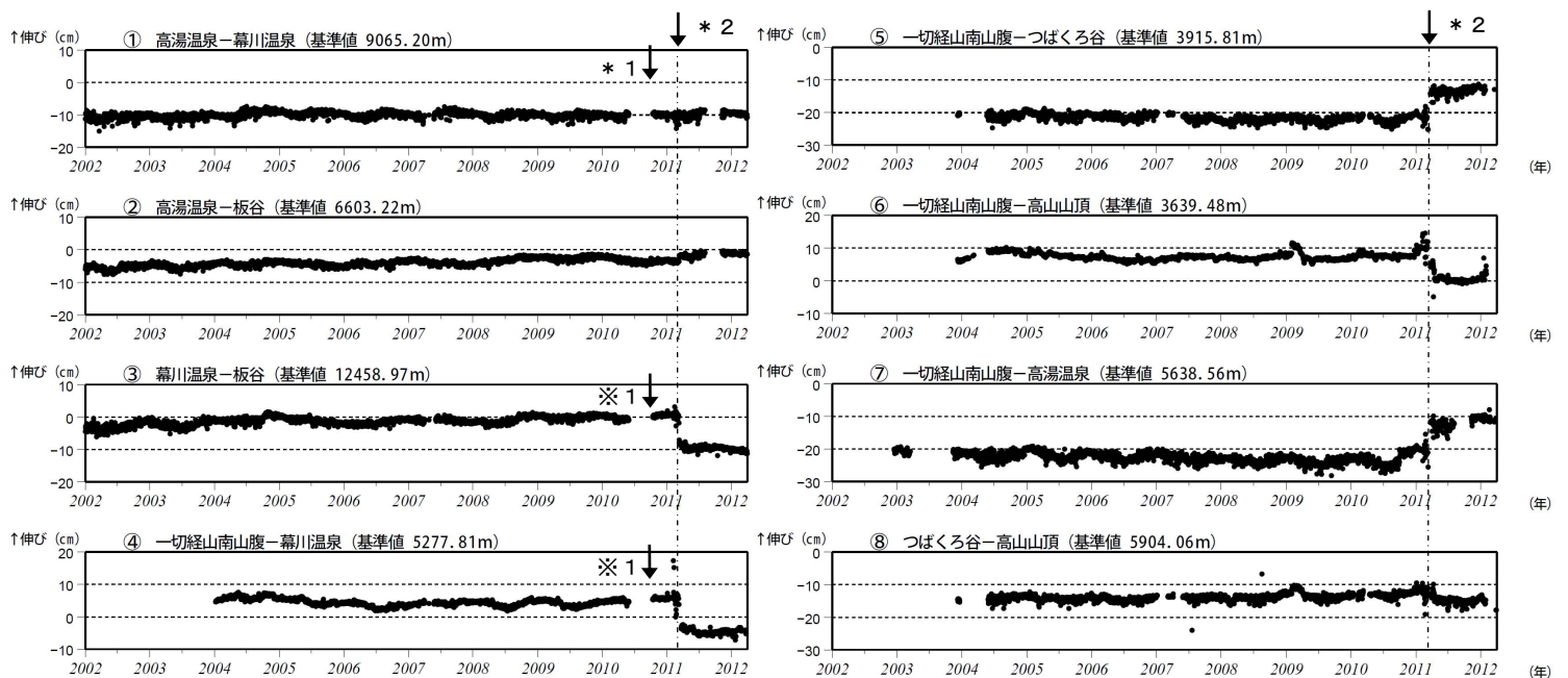
図 6 吾妻山 GPS 基線長変化図（2002 年 1 月～2012 年 3 月）
