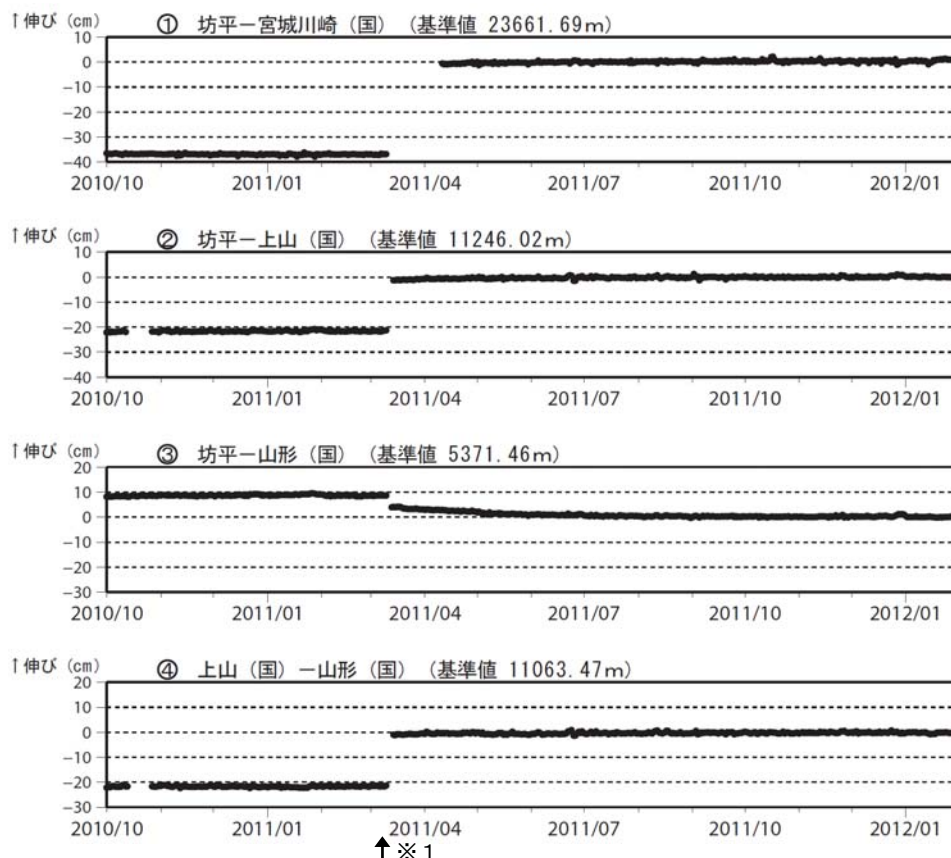
図 5※ 蔵王山 GPS 基線長変化図 (2010 年 10 月～2012 年 1 月) 2011 年 3 月 11 日以降の変動は、東北地方太平洋沖地震による影響であり、火山活動によるものではないと考えられます。
