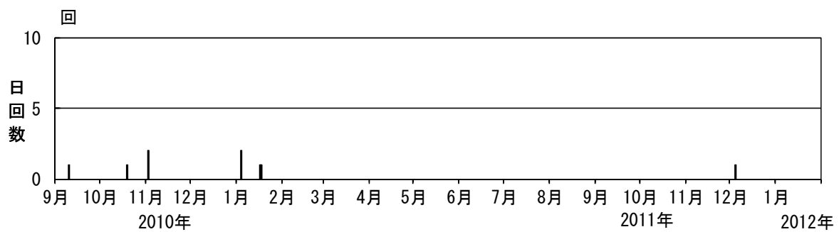
図3 蔵王山 火山性地震の日別回数（2010年9月～2012年1月）
