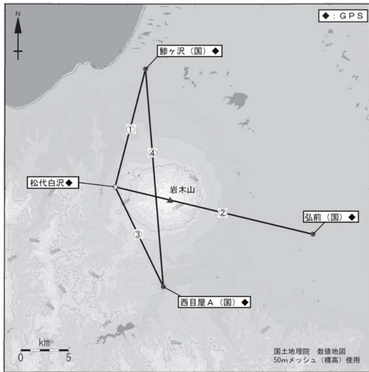
図 4 岩木山 GPS 観測点配置図
