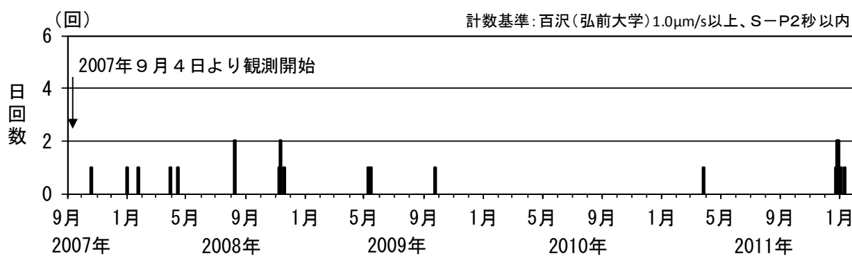
図3※ 岩木山 日別地震回数（2007年9月～2012年1月） 弘前大学からのデータ提供により、2007年9月4日から観測を開始しています。
