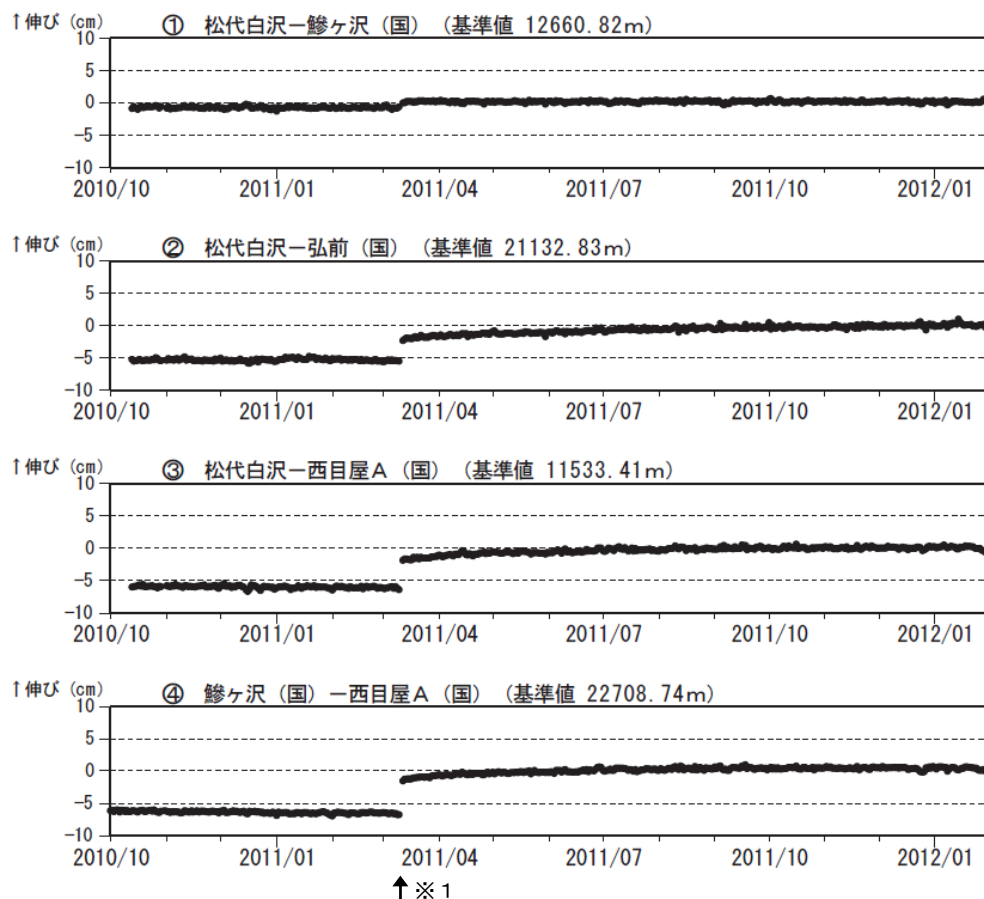
図 5※ 岩木山 GPS 基線長変化図（2010 年 10 月～2012 年 1 月）
