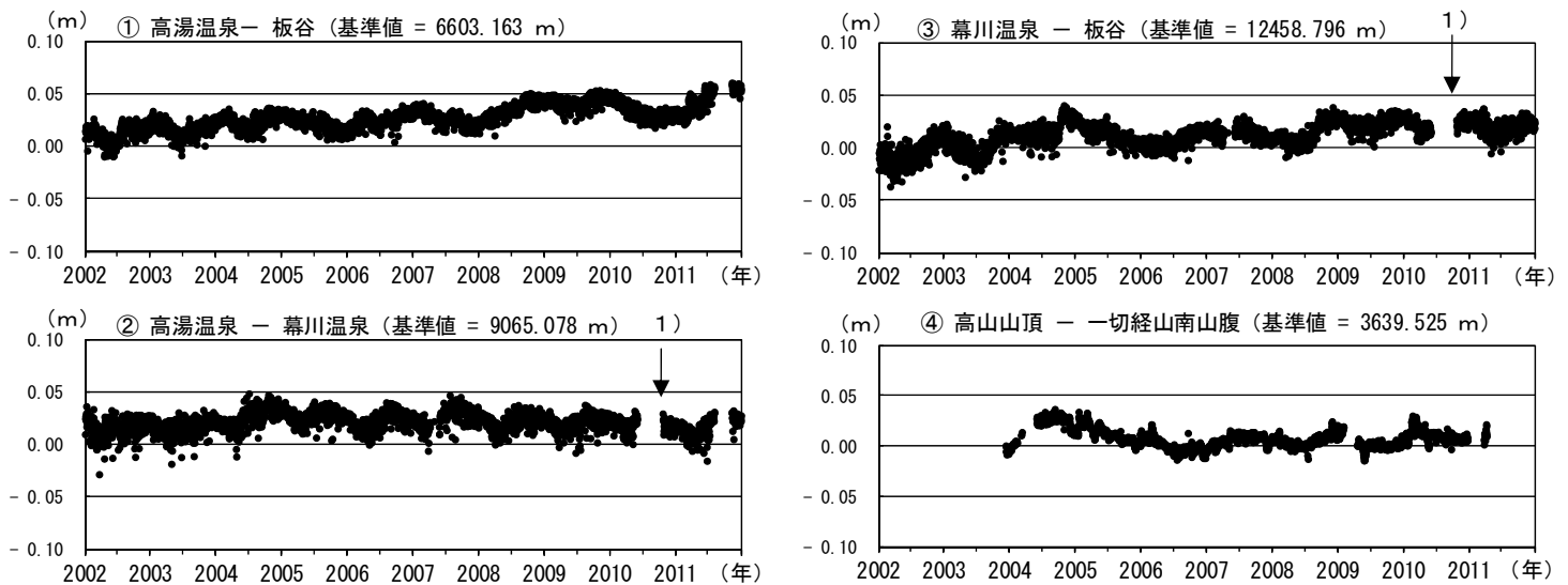
図6 吾妻山 GPS 基線長変化図（2002 年 1 月～2011 年 12 月）
